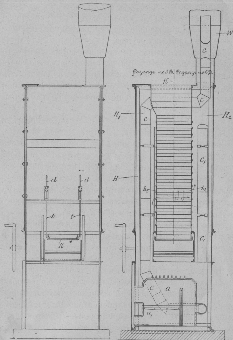
Рис. 11. Боковой видъ и долевоу вертикальный разрѣзъ зерносушилки Дюгиль.
