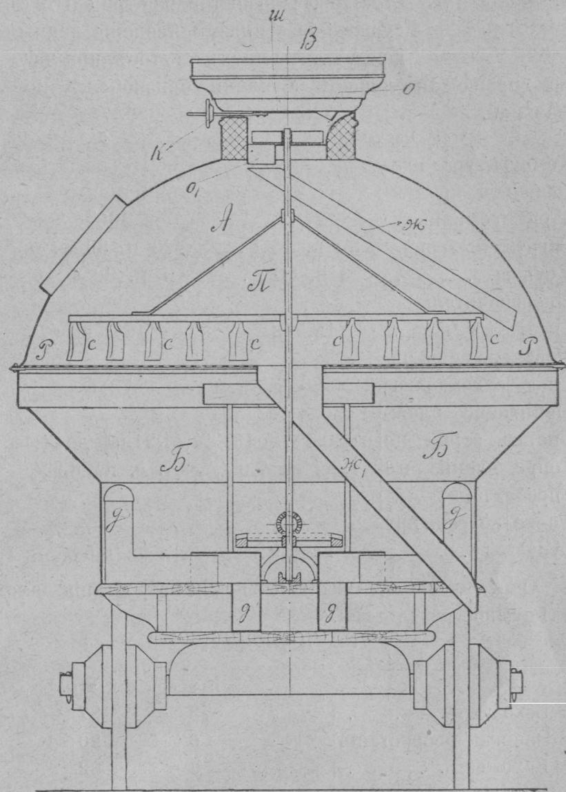
Рис. 8. Поперечный вертикальный разрѣзъ зерносушилки Растргина.
