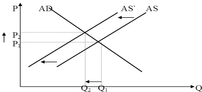
Рис. 7.4. Стагфляция
