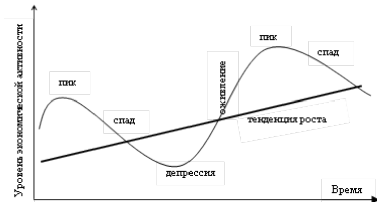
Рис. 10.1. Экономический цикл
