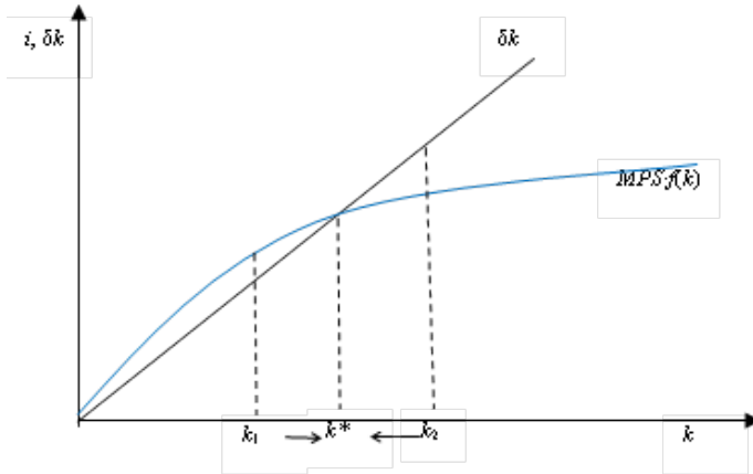
Рис. 10.6. Капиталовооруженность
