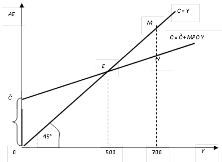
Рис. 3.2. Функция потребления
