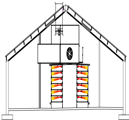
Рис. 2.21. Птичник с установленной системой «Патюо»
