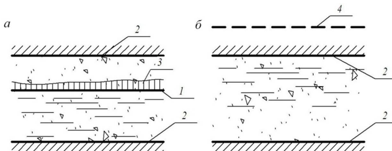
Рис. 5.7. Схема залегания межпластовых вод: а – безнапорных; б – напорных; I – уровень безнапорных вод; 2 – водоупор; 3 – капиллярная кайма; 4 – пьезометрический уровень
