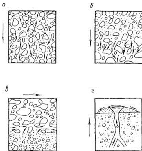
Рис. 7.11. Схемы разновидностей внутренней суффозии нескальных грунтов: а – объемная; б – фронтальная; в – контактный размыв мелкозернистого проплатка; г – канальная
