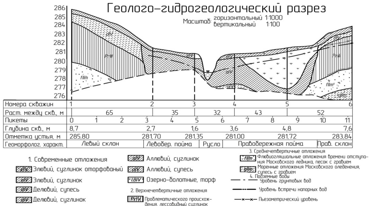
Рис. 8.3. Геолого-гидрогеологический разрез
