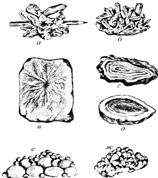
Рис. 2.5. Формы нахождения минералов в природе: а , б – друзы кристаллов гипса и кварца; в – дендрит марганцевых соединений на известняке; г – секрция; д – жеода; е – шаровидные конкреции; жс – почковидные натечные формы
