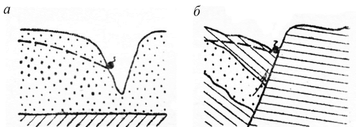
Рис. 5.10. Виды родников: а – нисходящие; б – восходящие
