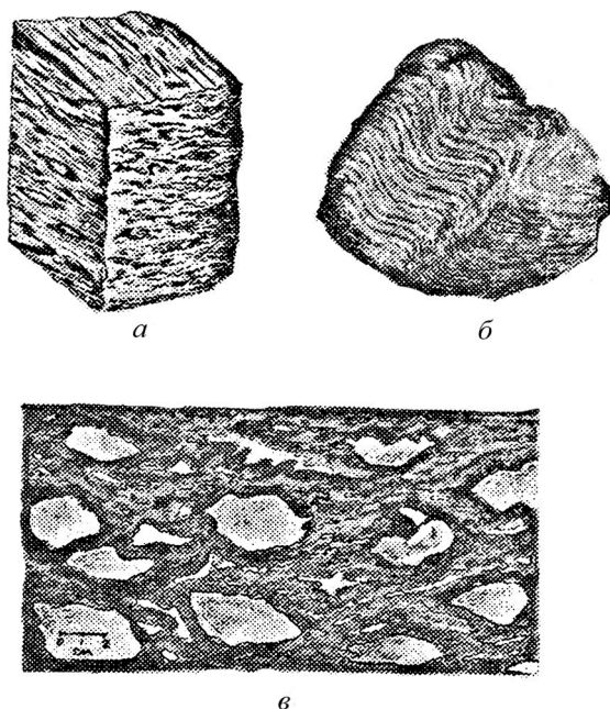
Рис. 2.11. Текстура метаморфических горных пород: а – сланцеватая; б – полосчатая; в – очковая
