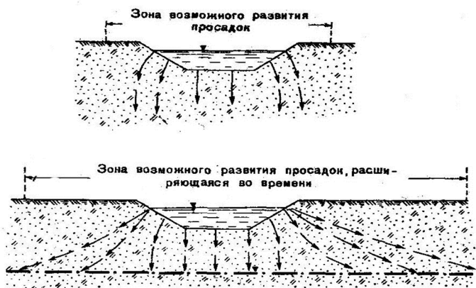
Рис. 7.8. Схема фильтрационного потока из канала и развитие просадки в лессовых породах
