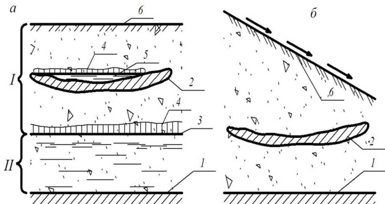
Рис. 5.4. Схема залегания верховодки: а – верховодка формируется за счет инфильтрации атмосферных осадков; б – верховодка формироваться не будет вследствие поверхностного стока; 1 – зона аэрации; II – зона насыщения; 1 – водоупор; 2 – водонепроницаемая прослойка пород в зоне аэрации; 3 – уровень грунтовых вод; 4 – капиллярная кайма; 5 – верховодка; 6 – поверхность земли
