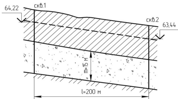
Рис. 6.11. Расчетная схема к примеру 6.4
