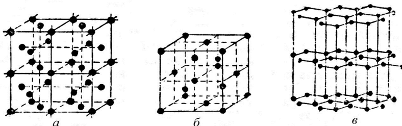
Рис. 2.1. Кристаллические решетки некоторых минералов: а – медь (спайность отсутствует); б – алмаз (спайность совершенная в четырех направлениях); в – графит (спайность весьма совершенная)
