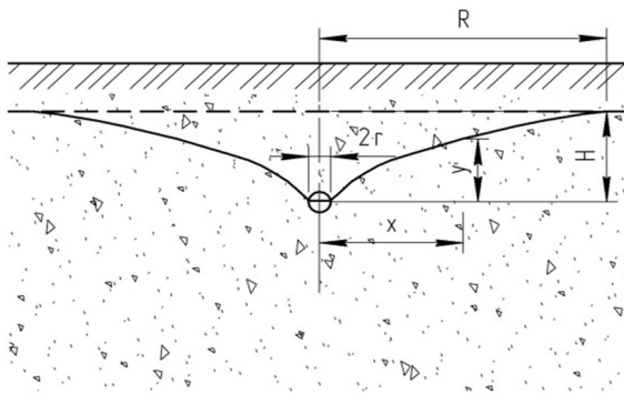
Рис. 6.30. Схема притока воды в несовершенную дренау
