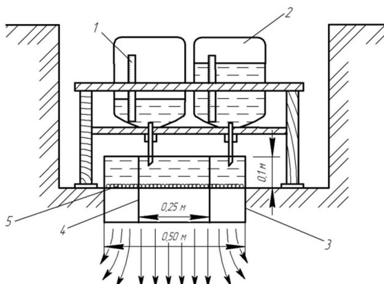
Рис. 6.35. Общий вид опытной установки по Н. С. Нестерову:
