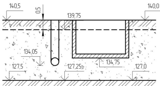
Рис. 6.31. Схема к расчету защитного дренажа промышленного предприятия
