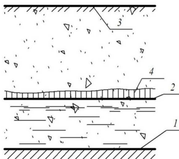
Рис. 5.5. Схема залегания грунтовых вод: 1 – водопор; 2 – уровень грунтовых вод; 3 – поверхность земли; 4 – капиллярная кайма
