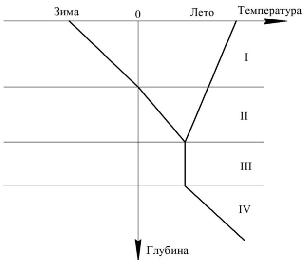
Рис. 1.2. График изменения температур с глубиной: I – зона промерзания; II – зона сезонных колебаний температур; III – зона постоянных температур; IV – зона геотермической закономерности
