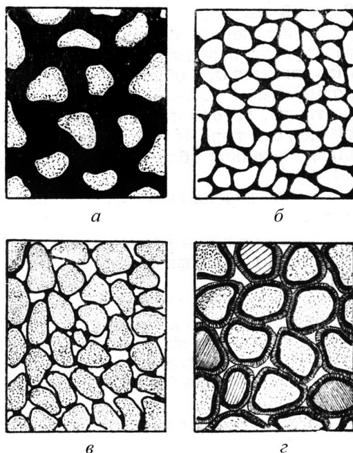
Рис. 2.10. Типы цементации (по М. С. Швецову): а – цемент базальный; б – цемент пор; в – цемент контактовый; г – цемент обрастания
