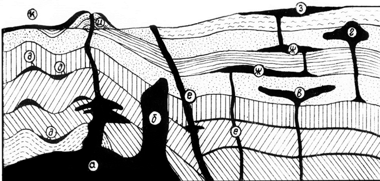
Рис. 2.6. Формы залегания магматических горных пород: а – батолит; б – штوك; в – лополит; г – лакколит; д – факолит; е – магматические жилы (дайки); ж – силлы; з – покров; и – вулканический конус; к – лавовый поток
