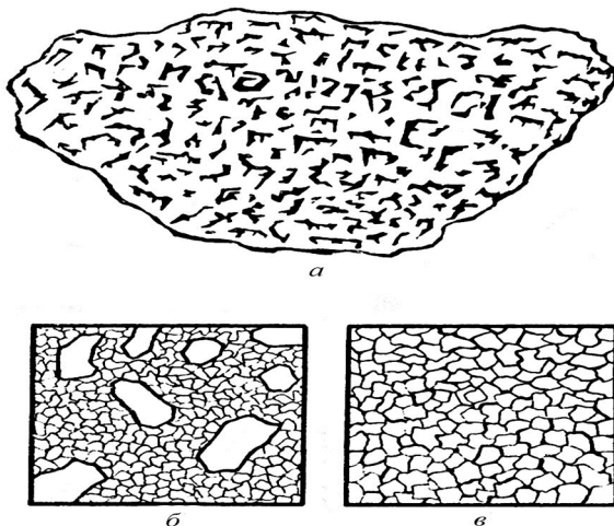
Рис. 2.7. Структура интрузивных пород: а – пегматитовая; б – полнокристаллическая, неравномерно-зернистая (порфировидная); в – полнокристаллическая, равномерно-зернистая
