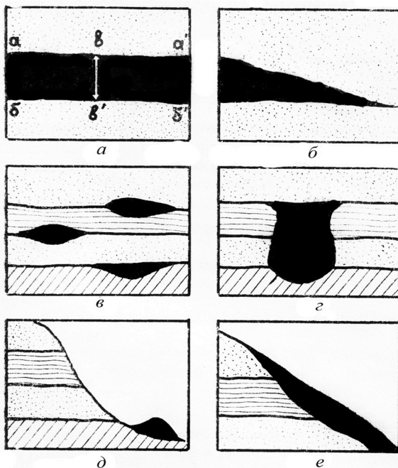
Рис. 2.9. Формы залегания осадочных пород:
