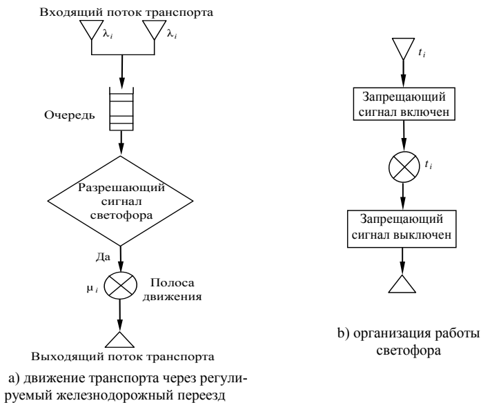
Рис. 1. Математическая модель железнодорожного переезда
