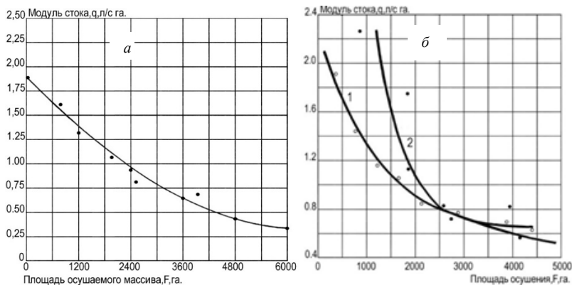
Рис. 2. Фактические значения модулей стока с польдерных систем и аппроксимирующие их зависимости: a – Белорусское Полесье от площади осушаемого массива, q = 1,98\exp(-0,0003F)[5] ; б – 1 – весеннее половодье q = 2\exp(-0,0003F) , 2 – летне-осенний паводок q = 3,1\exp(-0,0004F) [4]
