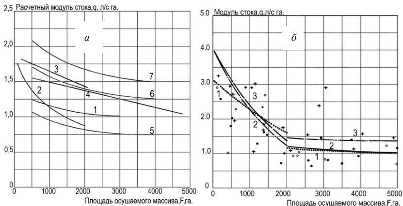
Рис. 1. а – нормативные данные, использовавшиеся при проектировании польдерных систем: 1-РПИ-82. Белоруссия, 2-НТД-85, Украина, 3-формула Т. Кадревич, 4 – формула А. Рикетса, 5, 6, 7 – «Временная инструкция по водохозяйственным и гидравлическим расчетам осушительных систем с механическим водоподъемом в Калининградской области»;
