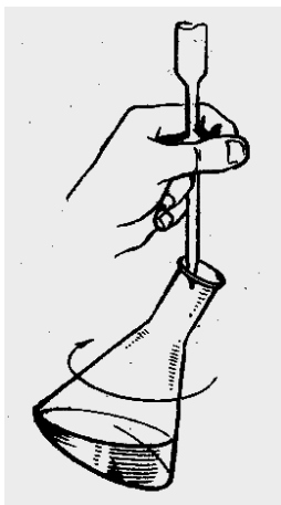
Рис. 14.4. Выполнение титрования
