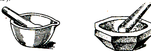
Рис. 13.5. Фарфоровая ступка с пестиком и агатовая ступка с пестиком
