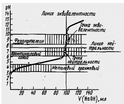
Рис. 14.7. Кривая титрования 100,0 мл 0,1 М CH 3 COOH 0,1 М раствором NaOH
