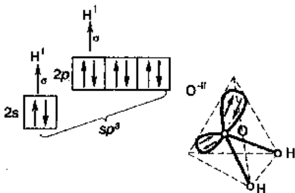
Рис. 4.6. Геометрия молекулы воды
