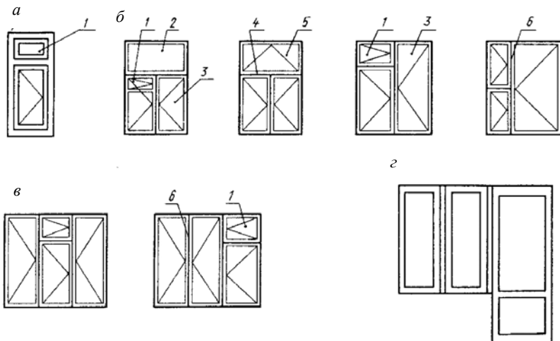
Рис. 5.3. Типы окон:
