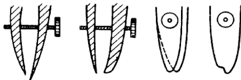
Рис. 1.4. Дефекты рейсфедера
