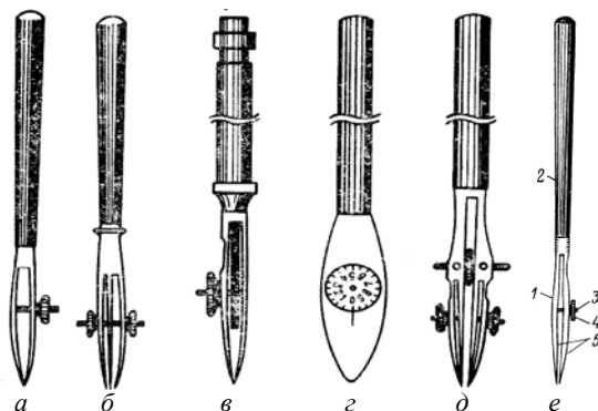
Рис. 1.3. Рейсфедеры:
