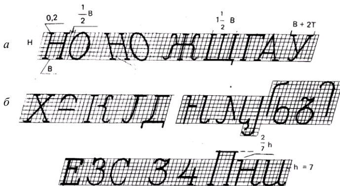
Рис. 2.4. Образец построения шрифта остовный курсив: a – нормативы и правила построения букв; б – элементы букв и примеры их сочетания
