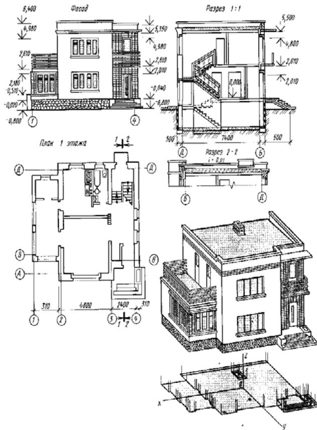
Рис. 6.1. Разрезы здания
