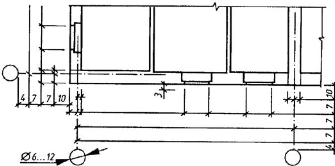
Рис. 6.7. Основные правила вычерчивания размерных линий на чертежах
