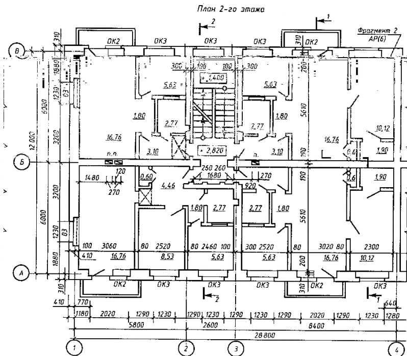
Рис. 6.15. План 2-го этажа многоквартирного жилого дома
