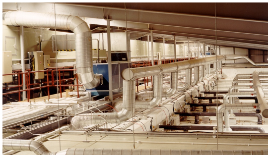
Рис. 1.3. Основной воздуховод вентиляционной системы
