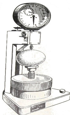
Рис. 3.12. ПУД-2Э
