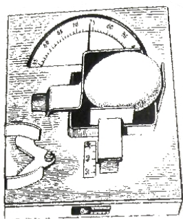
Рис. 3.11. Индексмер ИМ-1
