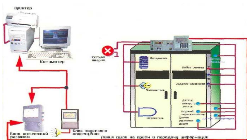
Рис. 1.23. Система управления инкубатором
