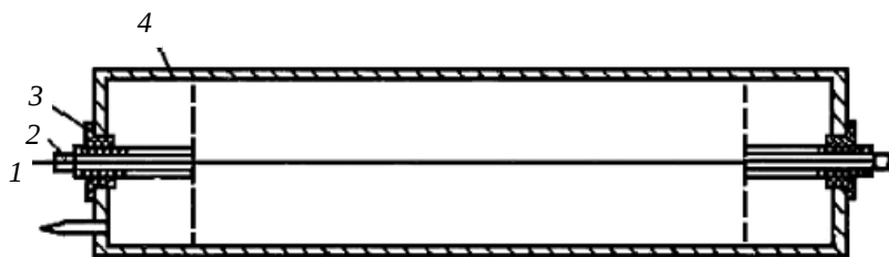
Рис. 29. Конструкция цилиндрического пропорционального счетчика: 1 – собирающий электрод; 2 – охранный электрод; 3 – изолятор; 4 – корпус
