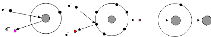
Рис. 7. Взаимодействие электронов и позитронов с веществом: — упругое рассеяние \beta -частиц на ядрах атомов; — упругое рассеяние \beta -частиц на электронах атома; — вариант смещения ядра атома с кристаллической решетки
