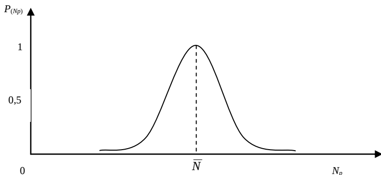
Рис. 3. Кривая распределения Пуассона: N – число импульсов, регистрируемых детектором; \bar{N} – среднее число регистрируемых импульсов
