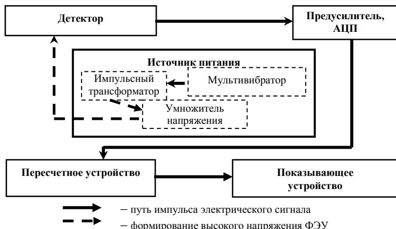
Рис. 17. Блок-схема радиометра
