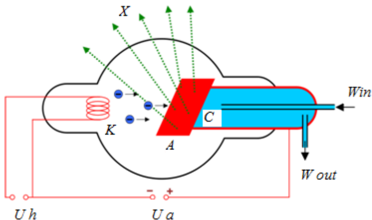
Рис. 10. Схематическое изображение рентгеновской трубки:
