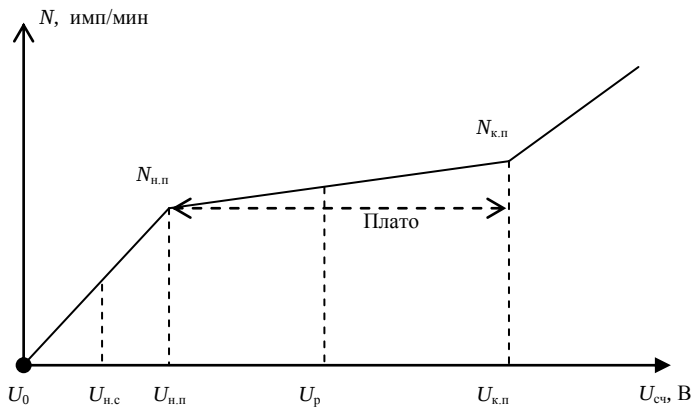
Рис. 34. Счетная характеристика счетчика Гейгера – Мюллера: U_{н.с} – напряжение начала счета; U_{н.п} – напряжение начала плато; U_{к.п} – напряжение конца плато; U_{р} – рабочее напряжение счетчика
