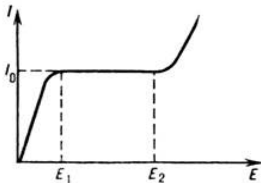
Рис. 23. Зависимость ионизационного тока I от приложенного электрического поля
