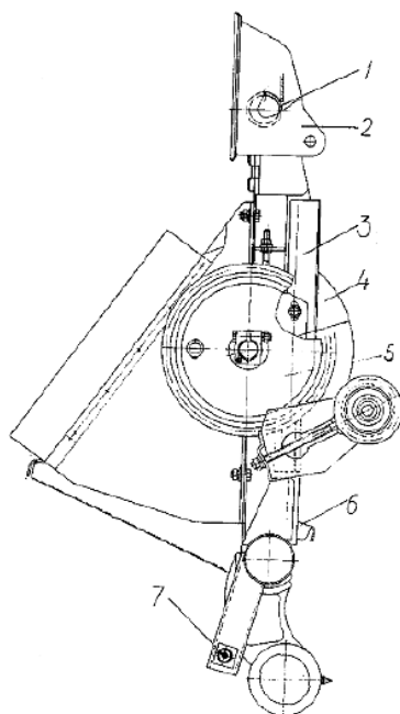
Рис. 4.16. Проставка: 1 – верхняя несущая труба; 2 – щека; 3 – корпус; 4 – битер; 5 – звездочка; 6 – днище; 7 – упорный ролик
