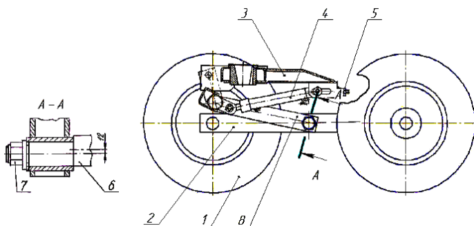
Рис. 2.5. Ходовая система: 1 – колесо с шиной; 2 – балансир; 3 – опора ротора; 4 – гидроцилиндр; 5 – гайка регулировочная; 6 – цапфа эксцентриковая; 7 – гайка цапфы; 8 – балка балансиров
