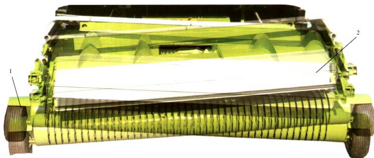
Рис. 4.35. Подборщик для комбайна Jaguar: 1 – копирующее колесо; 2 – рулонные направляющие
