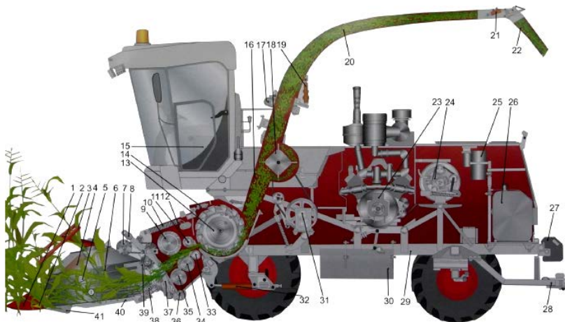
Рис. 4.2. Схема технологического процесса комбайна «Дон-680»: 1 – носок делителя; 2 – блок делителей; 3 – брус; 4 – активный делитель; 5 – барабан; 6 – прижим; 7 – устройство предохранительное; 8 – проставка жатки; 9 – валец верхний большой; 10 – механизм подпрессовки; 11 – валец верхний малый; 12 – питающий аппарат; 13 – барабан измельчающий; 14 – заточное устройство; 15 – кабина; 16 – конфузор; 17 – поворотное устройство; 18 – ускоритель массы; 19 – гидроцилиндр подъема силосопровода; 20 – силосопровод; 21 – гидроцилиндр подъема козырька силосопровода; 22 – козырек; 23 – моторно-силовая установка; 24 – гидропривод ходовой части; 25 – гидробак; 26 – топливный бак; 27 – груз противовеса; 28 – прицепное устройство; 29 – рама комбайна; 30 – инструментальный ящик; 31 – редуктор ускорителя; 32 – гидроцилиндр подъема адаптера; 33 – валец питателя задний нижний гладкий; 34 – валец нижний средний; 35 – валец нижний передний с металлодетектором; 36 – контрпривод жатки; 37 – бита проставки нижний; 38 – валец жатки; 39 – бита проставки верхний; 40 – режущий аппарат; 41 – подошва
