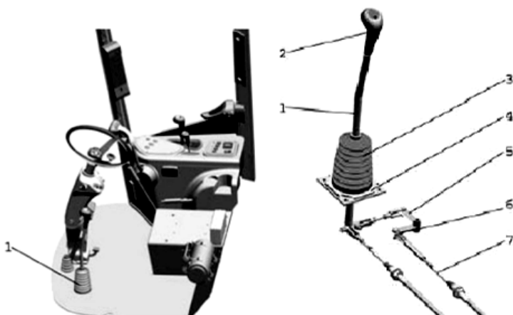
Рис. 4.29. Управление редуктором режима речки: 1 – рычаг управления редуктором режима речки; 2 – рукоятка; 3 – чехол; 4 – опора; 5 – блок рычагов; 6 – вилка; 7 – трос дистанционного управления
