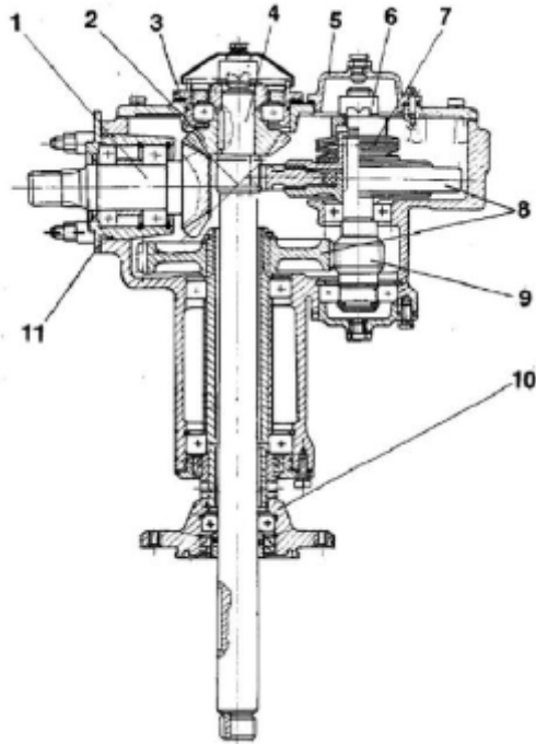
Рис. 4.8. Цилиндрический редуктор: 1, 2 – конические шестерни; 3, 11 – регулировочные прокладки; 4, 9 – вал шестерни; 5 – крышка; 6 – гайка; 7 – тарельчатая пружина; 8 – зубчатое колесо; 10 – вал привода барабана
