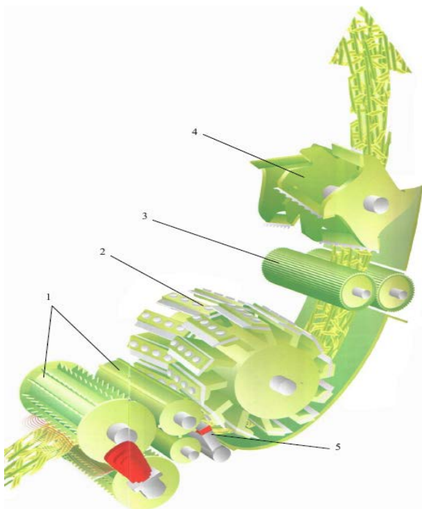
Рис. 4.34. Технологическая схема кормоуборочного комбайна Jaguar: 1 – питатели; 2 – измельчитель с V-образными ножами; 3 – доизмельчитель зерна кукурузы; 4 – ускоритель выброса доизмельченной растительной массы; 5 – противорежущая пластина
