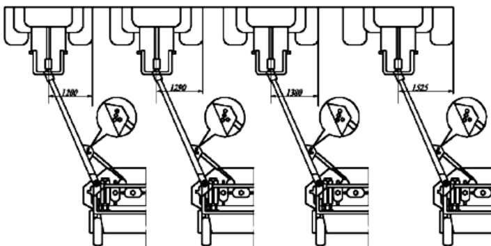
Рис. 1.5. Схема корректировки бокового смещения дышла прицепного устройства
