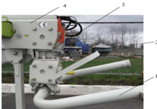
Рис. 1.6. Изменение числа оборотов вала отбора мощности: 1 – прицепная скоба; 2 – двойная передача; 3 – воздушный клапан; 4 – дышло
