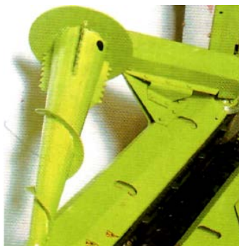
Рис. 4.41. Подающий шнек
