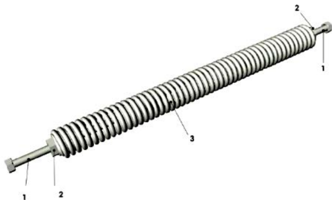
Рис. 2.12. Пружина: 1 – тяги; 2 – пробки; 3 – пружина
