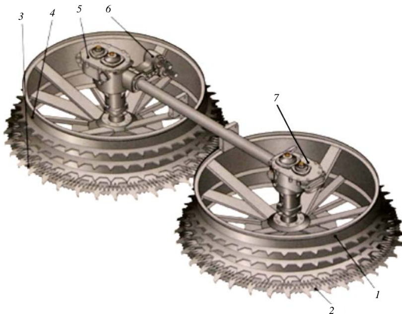
Рис. 4.4. Блок барабанов с угловым приводом: 1 – барабан левый; 2 – режущий аппарат левый; 3 – режущий аппарат правый; 4 – барабан правый; 5 – угловой редуктор правый; 6 – цилиндрический редуктор; 7 – угловой редуктор левый
