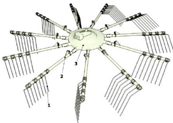
Рис. 2.8. Ротор: 1 – граблина; 2 – штанга; 3 – редуктор
