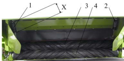
Рис. 1.8. Настройка натяжения валцов плющилки: 1, 2 – пружины; 3 – верхний валец; 4 – нижний валец
