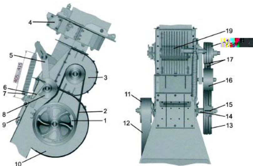
Рис. 4.32. Установка доизмельчителя зерна: 1, 13 – шкив привода доизмельчителя зерна; 2 – ремень привода доизмельчителя; 3 – доизмельчитель зерна; 4 – устройство поворотное; 5 – рычаг натяжного устройства; 6 – направитель потока массы; 7 – пружина натяжного устройства; 8, 16 – шкив натяжной; 9 – крышка; 10 – конфузор с ускорителем; 11 – шкив привода ротора ускорителя массы; 12 – ремень привода ускорителя массы; 13 – ведущий шкив; 14 – вал ротора ускорителя массы; 15 – шпонка; 17 – ремни привода ротора доизмельчителя зерна; 18 – шкив привода ротора доизмельчителя зерна; 19 – ротор доизмельчителя зерна
