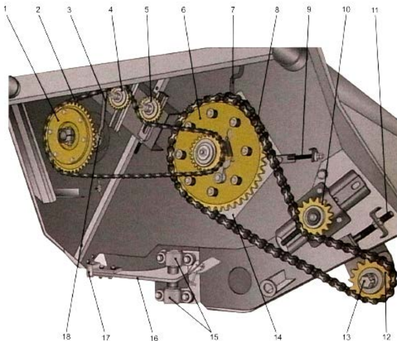
Рис. 4.14. Механизм привода шнека и мотовила: 1 – устройство предохранительное мотовила; 2 – цепь привода мотовила; 3 – тяга регулировки положения мотовила; 4 – обводная звездочка; 5 – натяжная звездочка; 6 – устройство предохранительное шнека жатки; 7 – тяга регулировки шнека по высоте; 8 – цепь привода шнека; 9 – тяга регулировки шнека по горизонтали; 10 – натяжная звездочка цепи привода шнека; 11 – тяга регулировки положения вала контрпривода; 12 – звездочка контрпривода; 13 – вал контрпривода; 14 – плита шнека; 15 – опора колебателя привода ножа; 16 – колебатель привода ножа режущего аппарата; 17 – головка привода ножа; 18 – пластина регулировки положения мотовила и наклона граблей
