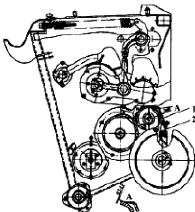
Рис. 4.26. Регулировка зазора между чистиком и гладким валцом питающего аппарата: 1 – чистик; 2 – регулировочная планка
