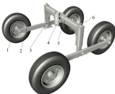
Рис. 2.10. Каретка: 1 – колесо; 2 – коромысло; 3 – стойка; 4 – обойма; 5 – балка; 6 – винт
