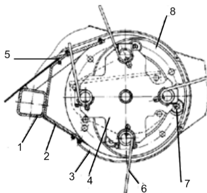
Рис. 4.18. Подбирающее устройство: 1 – труба; 2 – кронштейн; 3 – скат; 4 – вал; 5 – держатель; 6 – зуб; 7 – эксцентрик с роликом; 8 – беговая дорожка
