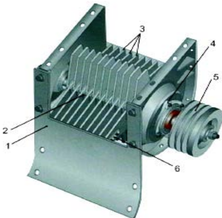
Рис. 4.31. Доизмельчитель зерна: 1 – корпус; 2 – ротор; 3 – ножи; 4 – опора с подшипником; 5 – шкив привода ротора; 6 – балансировочная пластина
