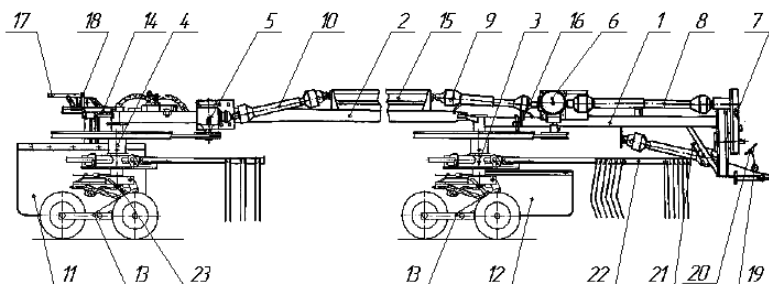
Рис. 2.2. Грабли роторные ГР-700: 1 – рама передняя; 2 – рама задняя; 3 – ротор передний; 4 – ротор задний; 5, 6 – конические редукторы; 7 – цепная передача; 8–10 – карданные валы; 11, 12 – фартуки; 13 – балансирная ходовая система; 14 – механизм перевода; 15 – трансмиссионный вал; 16 – фиксатор; 17 – ручка стопорная; 18 – фиксатор стопора; 19 – строп страховочный; 20 – замок; 21 – кронштейн огнетушителя; 22 – граблина с зубьями сребания; 23 – фиксатор транспортного положения
