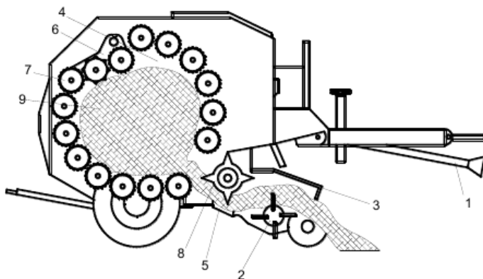
Рис. 3.1. Пресс-подборщик Rollant 250: 1 – карданный вал; 2 – барабанный подборщик; 3 – прижимное устройство; 4 – прессовальная камера; 5 – отражательный щиток; 6 – качающийся сегмент; 7 – прессовальные вальцы; 8 – захватывающий ротор; 9 – прессуемая масса
