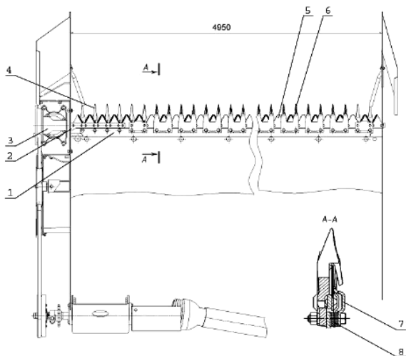
Рис. 4.12. Режущий аппарат: 1 – пальцевой брус; 2 – пятка ножа; 3 – кривошип редуктора; 4 – палец; 5 – сегмент; 6 – нож; 7 – прижим; 8 – прокладки
