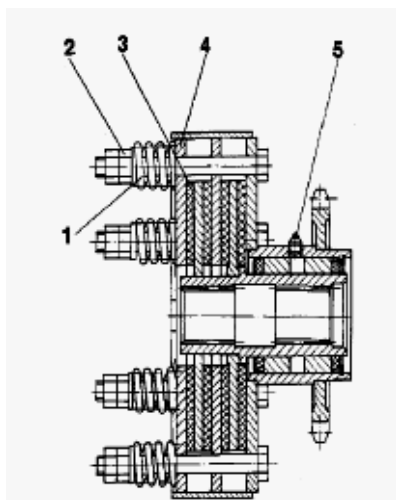
Рис. 4.7. Муфта проставки: 1 – пружина; 2 – гайка; 3 – фрикционная накладка; 4 – нажимной диск; 5 – масленка
