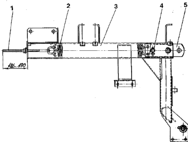
Рис. 4.6. Балка навески с механизмом уравнивания: 1 – винт регулировочный; 2 – блок пружин; 3 – балка навески; 4 – ось транспортная; 5 – хвостовик
