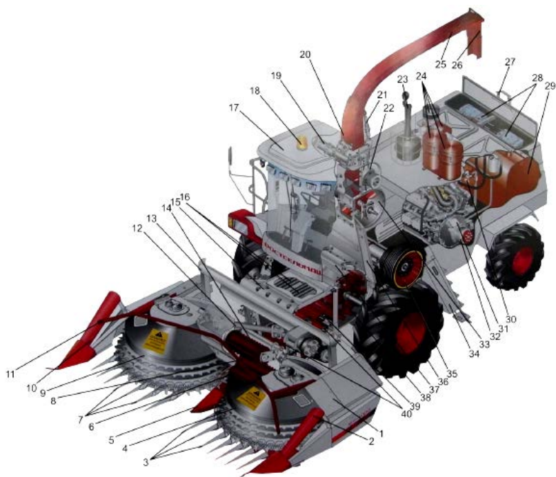
Рис. 4.1. Самоходный кормоуборочный комбайн «Дон-680М»: 1 – жатка роторная ЖР-4000; 2, 10 – активный делитель левый, правый; 3, 7 – блок делителей левый, правый; 4, 9 – барабан левый, правый; 5 – средний делитель; 6 – валец жатки; 8 – битуер проставки нижний; 11 – брус наклона массы передний; 12 – вал карданный привода барабанов; 13 – проставка жатки; 14 – валец проставки верхний плавающий; 15 – питающий аппарат; 16 – блок пружин механизма подпрессовки; 17 – кабина; 18 – проблесковый маяк; 19 – механизм поворота силосопровода; 20 – силосопровод; 21 – гидроцилиндр подъема силосопровода; 22 – доизмельчитель зерна; 23 – глушитель с инжектором; 24 – система воздухоочистки двигателя; 25 – гидроцилиндр поворота козырька; 26 – козырек силосопровода; 27 – упор силосопровода в транспортном положении; 28 – аккумуляторы; 29 – топливный бак; 30 – гидропривод ходовой части ГСТ-90; 31 – моторно-силовая установка; 32 – шкив привода измельчителя; 33 – ускоритель массы; 34 – лестница входа в кабину; 35 – шкив главного контрпривода; 36 – конфузор; 37 – измельчающий аппарат; 38 – измельчающий барабан; 39 – верхние валцы питателя; 40 – нижние валцы питателя
