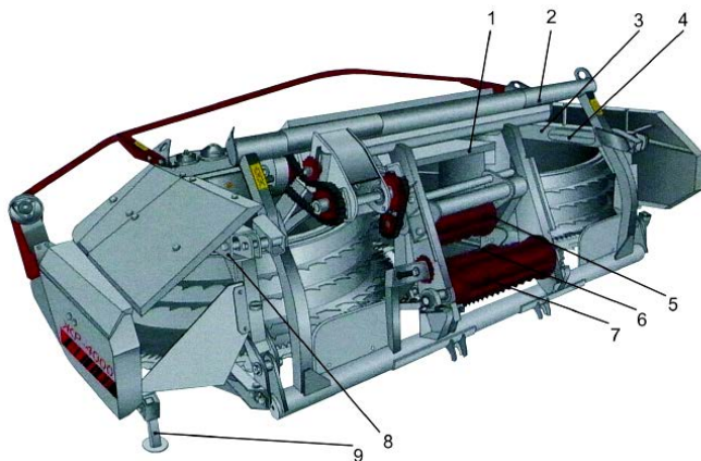
Рис. 4.5. Жатка роторная ЖР-4000 (вид сзади): 1 – приемная камера; 2 – проставка; 3, 8 – балки навески; 4 – блок пружин механизма уравнивания; 5 – бiter проставки верхний; 6 – валец жатки; 7 – бiter проставки нижний; 9 – стойка жатки
