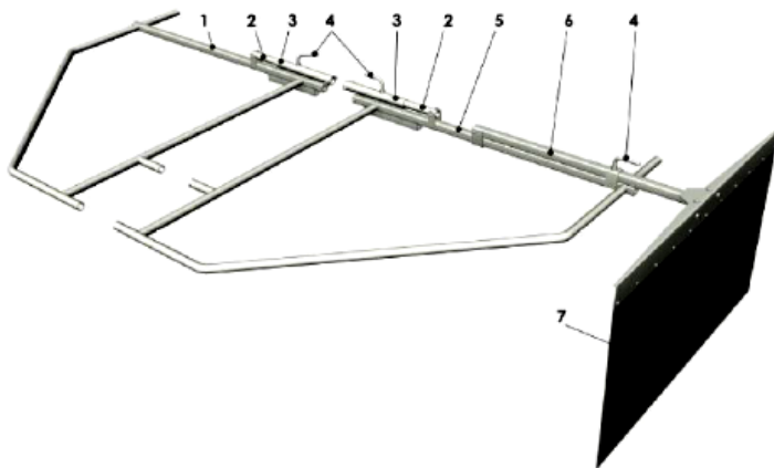
Рис. 2.13. Ограждения и отражатель: 1 – ограждение правое; 2 – распорки; 3 – фиксаторы; 4 – стопоры; 5 – ограждение левое; 6 – штанга; 7 – отражатель
