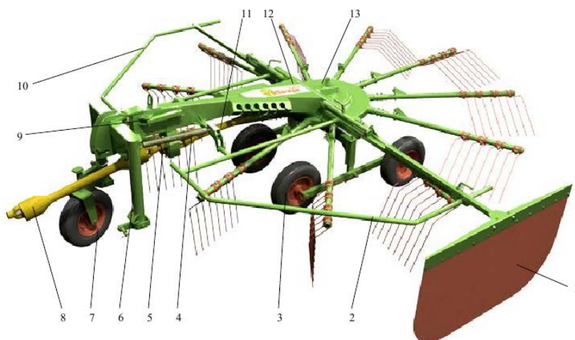
Рис. 2.6. Общий вид граблей: 1 – отражатель; 2 – ограждение левое; 3 – каретка; 4 – пружина; 5 – контрпривод; 6 – навеска; 7 – опорное колесо; 8, 11 – карданные валы; 9 – распорка транспортная; 10 – ограждение правое; 12 – рама; 13 – ротор
