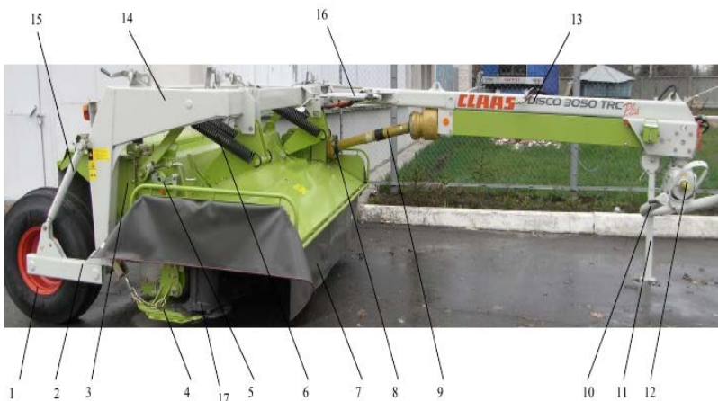
Рис. 1.3. Косилка роторная Disco 3050 TRC: 1 – колесо; 2 – держатель колеса; 3 – валкообразователь; 4 – косилочный брус; 5 – механизм регулировки высоты среза; 6 – пружины регулировки разгрузки косилочного бруса; 7 – защитный фартук; 8 – угловая передача; 9 – приводной вал; 10 – прицепная скоба; 11 – опорная стойка; 12 – двойная передача; 13 – дышло; 14 – рама; 15 – цилиндр подъема косилки; 16 – поворотный цилиндр; 17 – ротор
