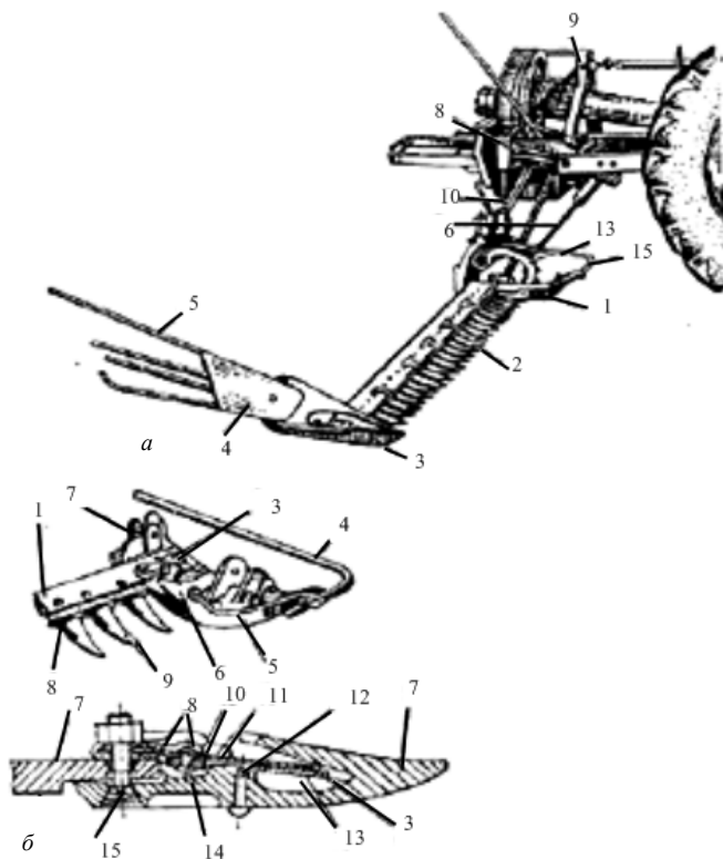
Рис. 1.1. Косилка КС-2,1: a – общий вид: 1, 3 – внутренний и наружный башмаки; 2 – режущий аппарат; 4 – полевая доска; 5 – прутки-стеблеотводы; 6 – шпренгель; 7 – тяговая штанга; 8 – рама; 9 – подвеска; 10 – главный шарнир; 11 – прут; б – режущий аппарат: 1 – пальцевый брус; 2 – полозок; 3, 6 – направляющие головки ножа; 4 – прут; 5 – внутренний башмак; 7 – палец; 8 – сегмент ножа; 9 – пластинка трения; 10 – спинка ножа; 11 – прижим; 12, 14 – заклепки; 13 – вкладыш; 15 – болт
