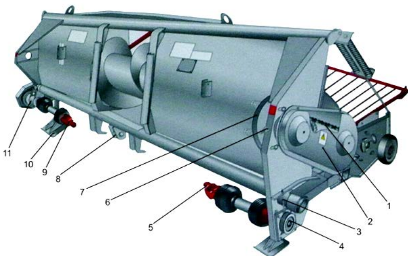
Рис. 4.19. Платформа-подборщик (вид сзади): 1 – цепь привода шнека; 2 – правый рычаг шнека; 3 – винт натяжной цепи привода верхнего вала; 4 – нижний вал; 5 – вал карданный привода шнека платформы; 6 – натяжной винт цепи привода шнека; 7 – устройство предохранительное шнека платформы; 8 – шарнир соединения платформы; 9 – вал карданный привода подборщика; 10 – левая опора установки платформы; 11 – контрпривод подборщика
