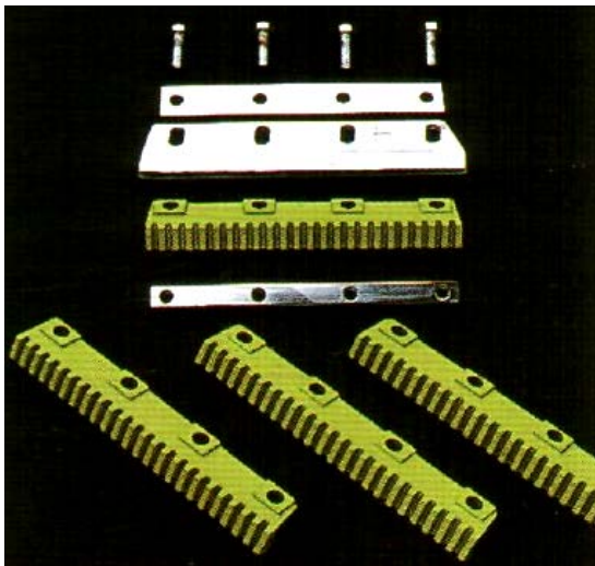
Рис. 4.38. Терочные доски с микроударными пластинами
