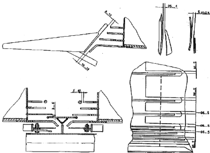
Рис. 4.9. Зазоры между приемной камерой и барабаном, барабаном и блоком делителей, барабаном и прутковым делителем
