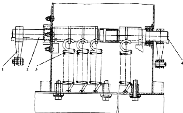
Рис. 4.24. Настройка положения вальцов питающего аппарата: 1 – рычаг; 2 – левый торсион; 3 – пружина; 4 – правый торсион
