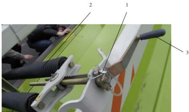
Рис. 1.4. Механизм разгрузки косилочного бруса: 1 – откидной штекер; 2 – пружина; 3 – ручка
