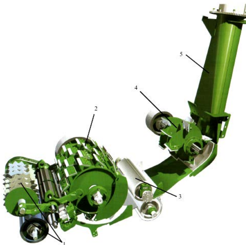
Рис. 4.47. Технологическая схема комбайна John Deere: 1 – подающие вальцы; 2 – измельчающий барабан; 3 – измельчитель зерна кукурузы; 4 – ускоритель; 5 – выгрузная труба
