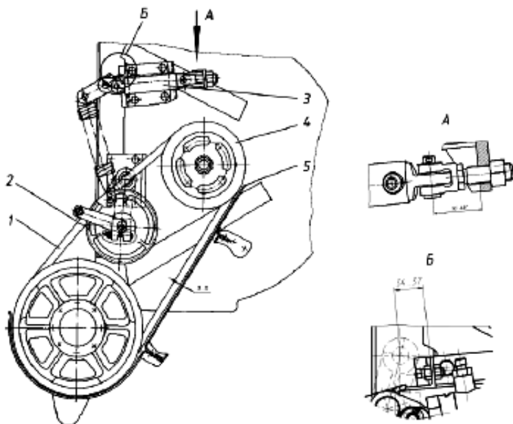
Рис. 4.25. Механизм включения леникса: 1 – ремень; 2 – натяжной шкив; 3 – гидроцилиндр; 4 – ведущий шкив; 5 – кожух
