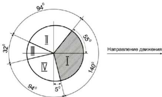
Рис. 2.9. Схема кольцевой направляющей дорожки: I – сектор, в котором граблины находятся в рабочем положении; II – сектор подъема граблин; III – сектор, в котором граблины находятся в поднятом положении; IV – сектор опускания граблин в рабочее положение
