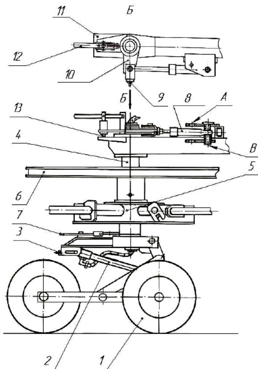
Рис. 2.3. Установка заднего ротора: 1 – ходовая система; 2, 8 – гидроцилиндры; 3 – регулируемый упор; 4 – ось; 5 – корпус ротора; 6 – шкив; 7 – рычаг с фиксатором; 9 – гайка регулировочная; 10 – рычаг поворота ходовой системы; 11 – сектор; 12 – рукоятка; 13 – фиксатор
