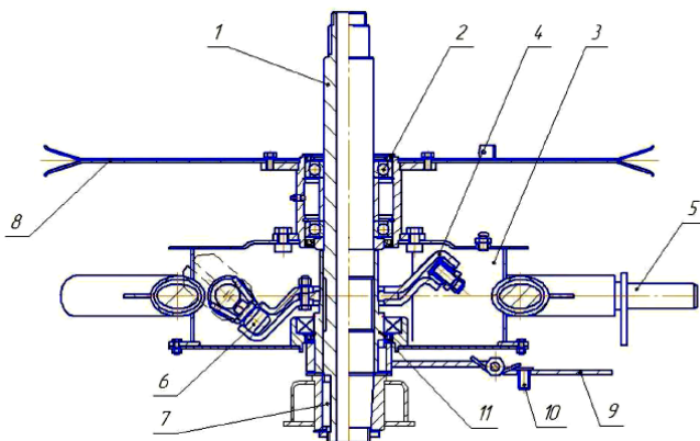
Рис. 2.4. Ротор: 1 – ось; 2 – подшипник; 3 – корпус; 4 – копир; 5 – ось граблины; 6 – кулачок с роликом; 7 – шпонка; 8 – шкив; 9 – рычаг; 10 – фиксатор; 11 – втулка
