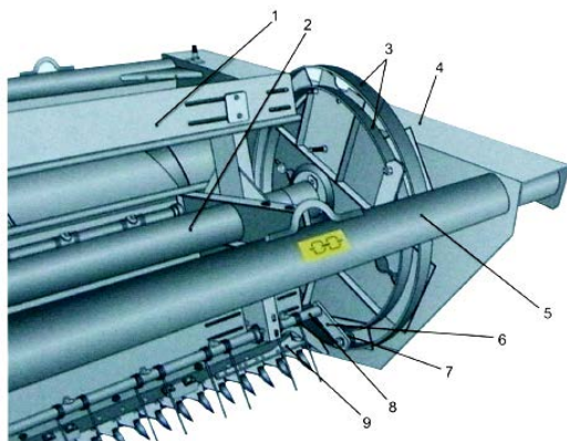
Рис. 4.13. Механизм копирования наклона граблей мотовила: 1 – лопасть мотовила; 2 – вал мотовила; 3 – направляющая дорожка механизма настройки угла наклона граблей мотовила; 4 – левая боковина жатки; 5 – передняя балка наклона массы; 6 – кронштейн ролика эксцентрикового механизма мотовила; 7 – ролик эксцентрикового механизма мотовила; 8 – труба граблей мотовила; 9 – нож режущего аппарата
