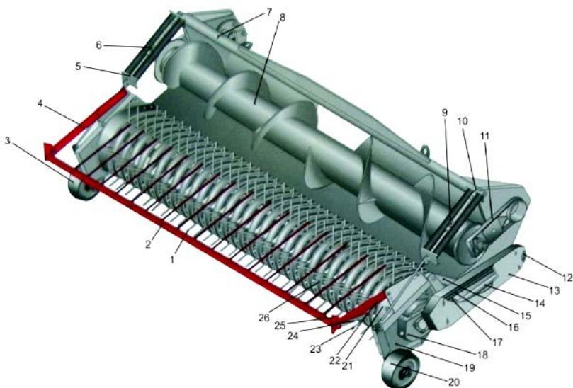
Рис. 4.17. Платформа-подборщик комбайна «Дон-680М»: 1 – палец прижима; 2 – труба прижима; 3 – правое опорное колесо; 4 – стойка прижима; 5, 10 – правый и левый блок пружин разгружающего устройства; 6, 9 – пальцы установки в транспортное положение; 7 – каркас; 8 – шнек платформы; 11 – левый рычаг шнека; 12 – шкив с муфтой обратного хода; 13 – защитный щиток; 14 – распорка натяжения ремней; 15 – рычаг крепления; 16 – ремни привода; 17 – шкив привода; 18 – редуктор привода; 19 – левая боковина; 20 – левое опорное колесо; 21 – скат боковой левый; 22 – левая стойка прижима; 23 – зубья пружинные подбирающего устройства; 24 – пружина натяжения прижима; 25 – кронштейн упора трубы прижима; 26 – скат подборщика
