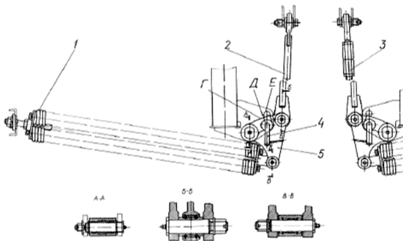
Рис. 4.15. Механизм уравнивания: 1 – блок пружин; 2 – подвеска левая; 3 – подвеска правая; 4 – штырь; 5 – рычаг; Г – упор; Д, Е – отверстия
