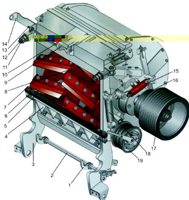
Рис. 4.27. Измельчающий аппарат: 1 – крюк навески питателя; 2 – рычаг навески; 3 – каркас измельчающего барабана; 4 – опора противорежущего бруса; 5 – брус противорежущий; 6 – болт крепления бруса; 7 – эксцентрик регулировки бруса; 8 – измельчающий барабан; 9 – конические шестерни подъема-опускания заточного бруса; 10 – крышка заточного устройства; 11 – стяжка крепления питателя; 12 – гайка стяжки; 13 – ось квадратная заточного устройства; 14 – кронштейн установки ключа; 15 – гидроцилиндр леникса питателя; 16 – шкив привода питателя; 17 – шкив привода измельчающего барабана; 18 – пружина леникса питателя; 19 – шкив леникса питателя
