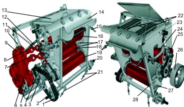
Рис. 4.21. Питающий аппарат комбайна «Дон-680М»: 1 – цепь двойная привода вала контрпривода жатки; 2 – вал контрпривода жатки; 3 – рычаг натяжного устройства цепи привода жатки; 4 – рычаг включателя муфты быстрого останова; 5 – опора редуктора питателя; 6 – механизм блокировки переключения длины резки; 7 – карданный вал привода малого верхнего вальца; 8 – карданный вал привода нижнего гладкого вальца; 9 – редуктор питателя; 10 – косынка крепления редуктора; 11 – растяжка регулируемая редуктора питателя; 12 – электромагнитная муфта быстрого останова; 13 – крышка механизма подпрессовки; 14 – захват питателя; 15, 21 – стяжные болты питателя и жатки; 16 – верхний большой валец; 17 – отсекатели; 18 – валец нижний средний; 19 – валец передний нижний (с металлодетектором); 20 – блок звездочек привода жатки; 22 – блоки пружин механизма подпрессовки вальцов; 23 – вал механизма подпрессовки; 24 – редуктор верхних вальцов; 25 – цепь привода среднего нижнего вальца; 26 – шкив контрпривода питателя; 27 – место регулировки положения датчика металлодетектора; 28 – рама
