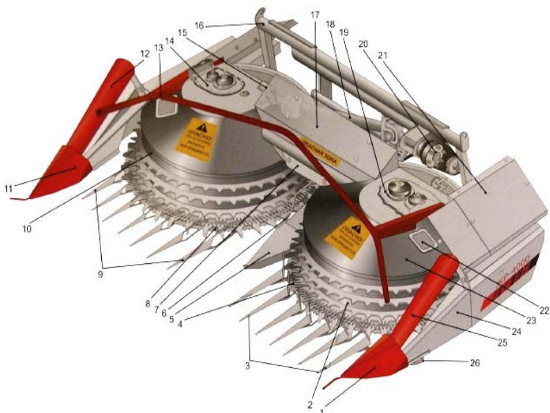
Рис. 4.3. Жатка роторная ЖР-4000: 1 – носок левого делителя; 2 – барабан левый; 3 – блок делителей левый; 4 – режущий аппарат левый; 5 – делитель средний; 6 – прижимной пруток среднего делителя; 7 – прижим массы; 8 – режущий аппарат правый; 9 – блок делителей правый; 10 – барабан правый; 11 – носок правого делителя; 12, 25 – активные делители; 13 – брус; 14 – угловой редуктор правый; 15 – цилиндрический редуктор; 16 – проставка; 17 – щиток защитный; 18 – вал карданный; 19 – угловой редуктор левый; 20 – муфта предохранительная; 21 – обшивка; 22 – крышка смотрового окна; 23 – кожух барабана; 24 – боковина делителя; 26 – подошва
