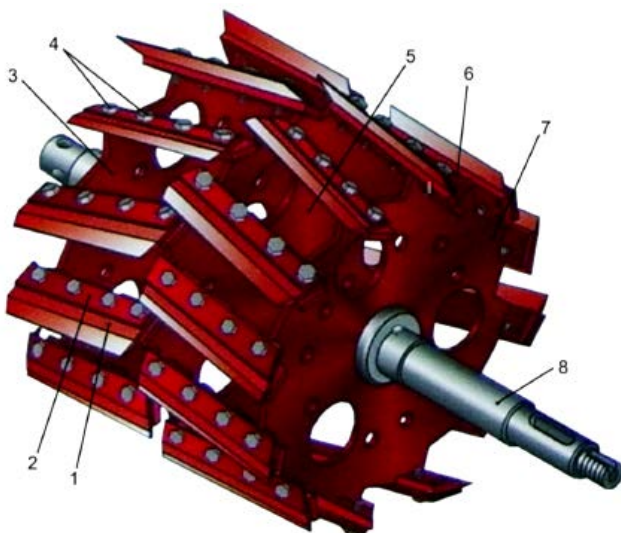
Рис. 4.28. Измельчающий барабан (шевронного типа): 1 – нож; 2 – прижим ножа; 3, 7 – диски крайние каркаса барабана; 4 – болты крепления ножей; 5 – диск средний каркаса барабана; 6 – опора ножа; 8 – вал барабана
