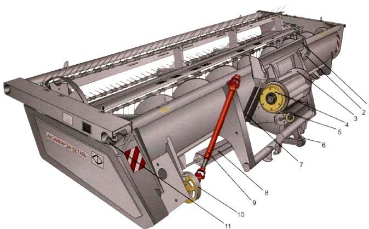
Рис. 4.11. Жатка травяная (вид сзади): 1 – проставка жатки; 2 – подвеска правая (регулируемая) механизма уравновешивания; 3 – битаер проставки; 4 – устройство предохранительное бitera проставки; 5 – звездочка натяжная цепи привода бitera; 6 – центральный шарнир; 7 – подвеска правая (нерегулируемая) механизма уравновешивания; 8 – блок пружин механизма уравновешивания; 9 – вал карданный привода жатки; 10 – шкив контрпривода и привода режущего аппарата; 11 – нож запасной
