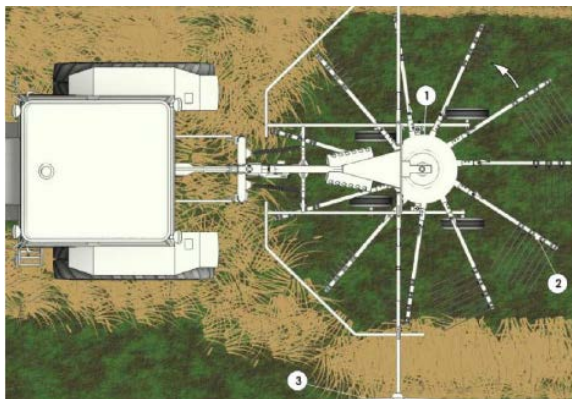
Рис. 2.7. Технологическая схема работы: 1 – ротор; 2 – граблины; 3 – отражатель
