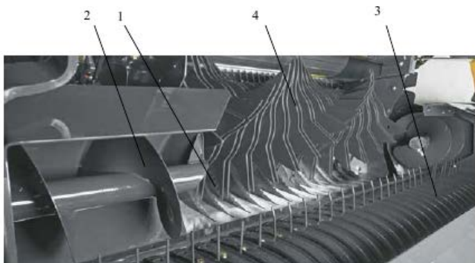
Рис. 3.3. Захватывающий ротор: 1 – нож; 2 – шнек; 3 – подборщик; 4 – ротор
