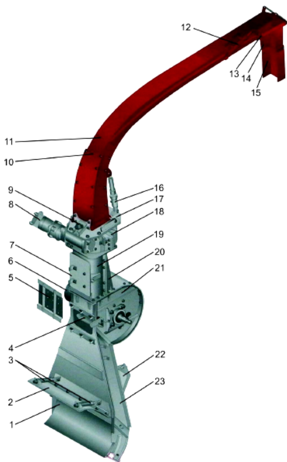
Рис. 4.30. Транспортирующее устройство: 1 – вставка (направитель потока массы); 2 – крышка измельчающего аппарата; 3 – пружины прижимные; 4 – лопасть ротора ускорителя массы; 5 – крышка ротора ускорителя; 6 – шкив привода ротора ускорителя; 7 – защитный щиток; 8 – гидромотор привода поворотного устройства силосопровода; 9 – болт откидной; 10 – накладка силосопровода (сменная); 11 – силосопровод; 12 – гидроцилиндр поворота козырька силосопровода; 13 – рычаг поворота козырька; 14 – козырек силосопровода; 15 – надставка козырька; 16 – гидроцилиндр подъема силосопровода; 17 – опора силосопровода; 18 – поворотное устройство силосопровода; 19 – переходник; 20 – сектор; 21 – корпус ускорителя; 22 – крышка смотрового люка; 23 – конфузор
