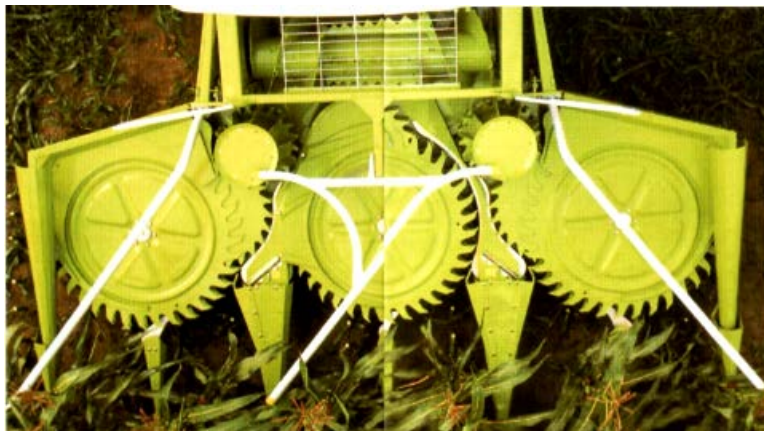
Рис. 4.45. Захватывающие диски
