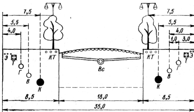
Рис. 4.12. Вариант размещения подземных сетей с двух сторон улицы: К – канализация; В – водопровод; Г – газопровод низкого давления; Т – телефонный кабель; Э – электрокабель; КТ – кабель троллейбуса; Вс – водосток
