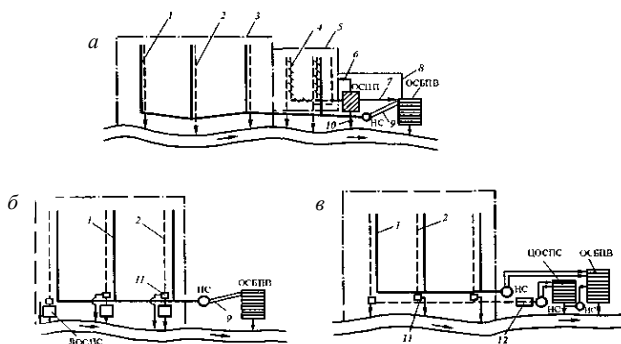
Рис. 3.2. Схемы полной отдельной системы водоотведения: а – без очистки поверхностного стока; б и в – с очисткой поверхностного стока соответственно на локальных и на централизованных очистных сооружениях; ОСБПВ – очистные сооружения бытовых и производственных вод; ОСПП – очистные сооружения промышленного предприятия; ЛОСПС – локальные очистные сооружения поверхностного стока; ЦОСПС – централизованные очистные сооружения поверхностного стока;
