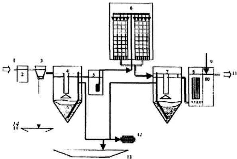
Рис. 6.21. Технологическая схема очистки сточных вод небольшого населенного пункта на биофильтрах с плоскостной загрузкой пропускной способностью 1000–10000 м 3 /сут:
