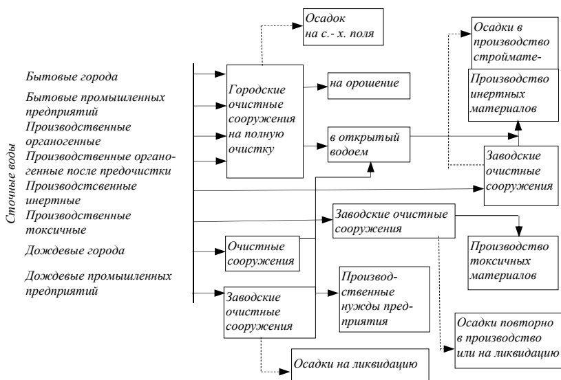
Рис. 3.6. Граф возможных вариантов водоотведения и рационального использования очищенных сточных вод при полной раздельной системе
