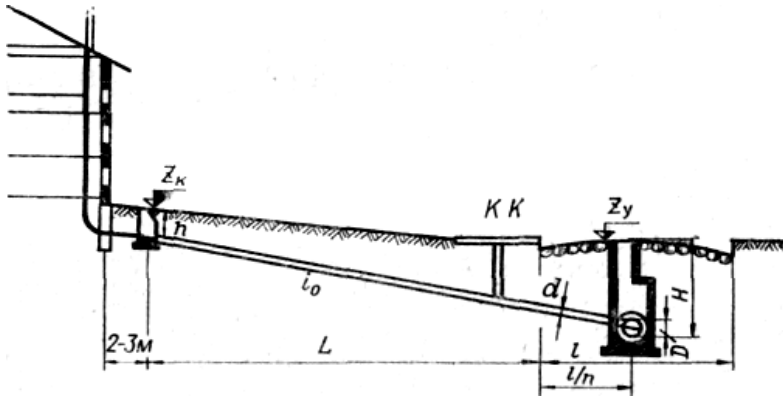
Рис. 4.10. Схема определения начальной глубины заложения уличной сети:
