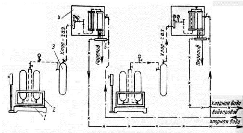
Рис. 6.23. Технологическая схема хлораторной производительностью до 5 кг/ч: 1 – весы; 2 – стойки с баллонами; 3 – грязеуловитель; 4 – хлоратор; 5 – эжектор
