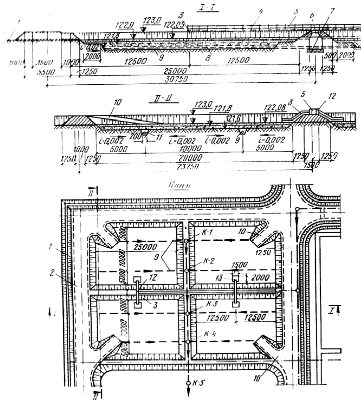
Рис. 6.13. Иловые площадки:
