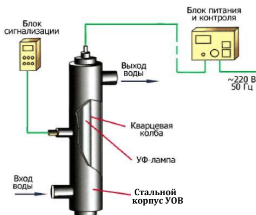
Рис. 6.24. Принципиальная схема ультрафиолетовой установки для обеззараживания воды
