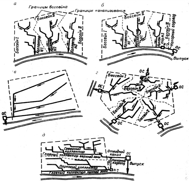
Рис. 4.5. Схемы водоотводящей сети: а – перпендикулярная; б – пересеченная; в – параллельная; г – децентрализованная радиальная; д – зонная; ОС – очистные сооружения; НС – насосная станция
