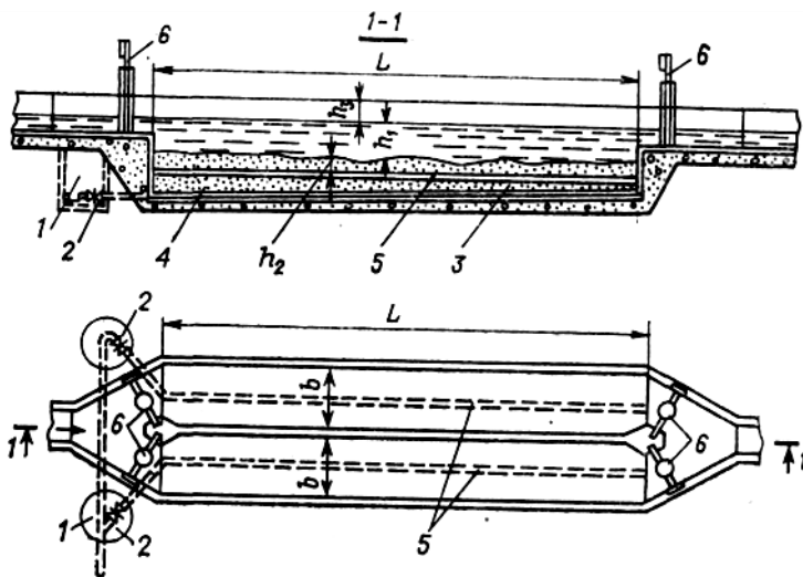
Рис. 6.6. Горизонтальная песколовка с прямолинейным движением сточных вод: 1 – колодец; 2 – задвижка; 3 – осадок; 4 – слой гравия; 5 – дренажная труба; 6 – шиберы
