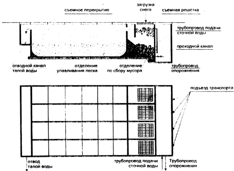
Рис. 4.30. Снегоплавная камера с улавливанием песка и крупных включений
