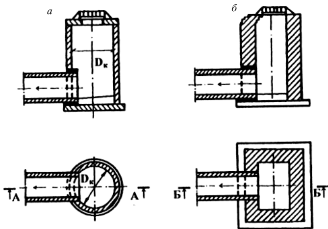
Рис. 4.31. Дождеприемники: а – круглые железобетонные; б – прямоугольные кирпичные
