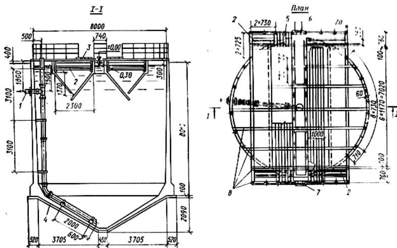
Рис. 6.12. Одиночный двухъярусный отстойник:
