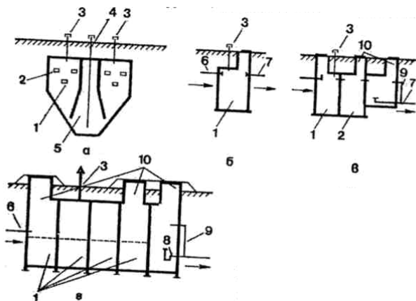
Рис. 6.14. Септики:
