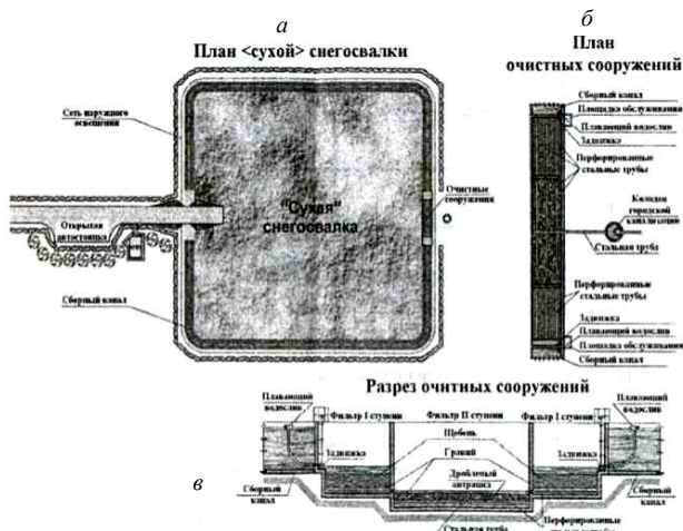
Рис. 4.29 «Сухая» снегосвалка: a – план «сухой» снегосвалки; б – план очистных сооружений; в – разрез очистных сооружений
