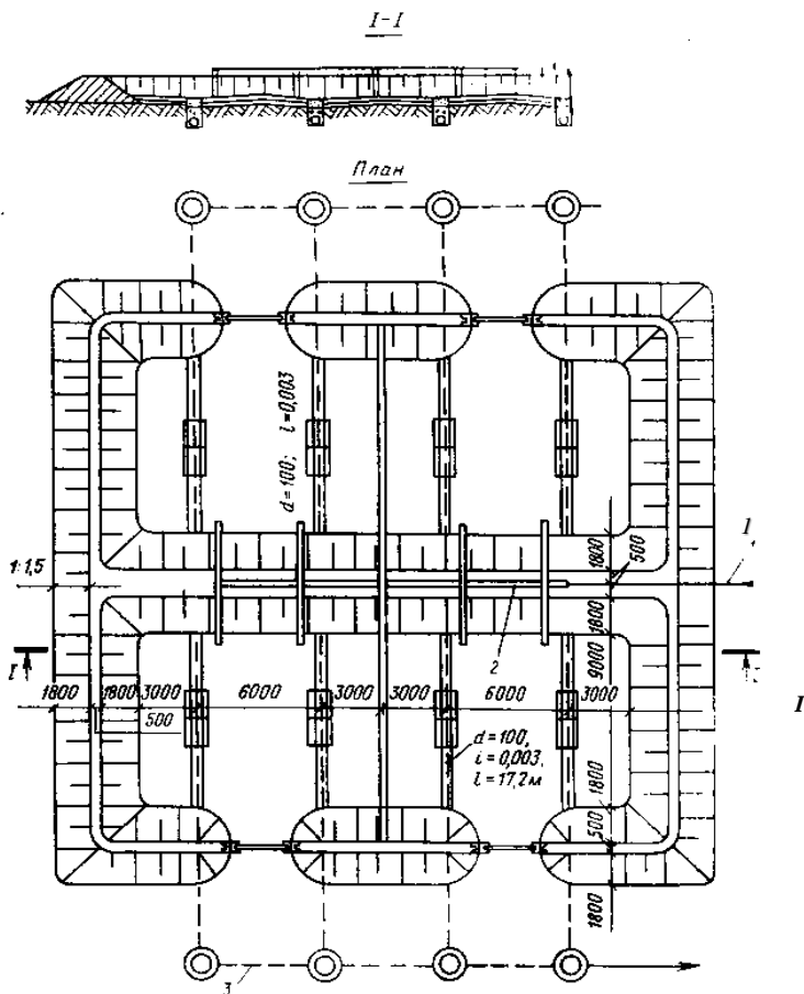
Рис. 6.7. Песковая площадка: 1 – пескопровод; 2 – разводящий лоток; 3 – трубопровод для отвода дренажной воды
