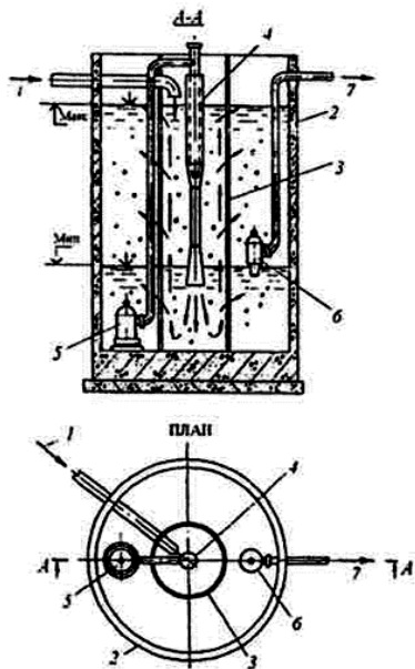
Рис. 6.20. Установка «Контакт»: 1 – подача сточной жидкости; 2 – емкость аэротенка; 3 – центральная цилиндрическая сетка; 4 – эжекторный аэратор; 5 – циркулярный насос; 6 – насос для откачки очищенных сточных вод; 7 – выпуск очищенной воды
