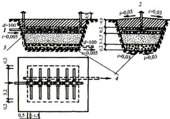
Рис. 6.18. Песчано-гравийный фильтр:
