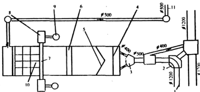
Рис. 4.27. Очистные сооружения камерного типа: 1 – подводный коллектор; 2 – разделительная камера; 3 – вход осветляемой воды; 4 – переливная стенка; 5 – решетка; 6 – плавающий понтон; 7 – сборник нефтепродуктов; 8 – нефтесепараторная камера; 9 – слив воды; 10 – фильтры доочистки; 11 – отвод очищенной воды
