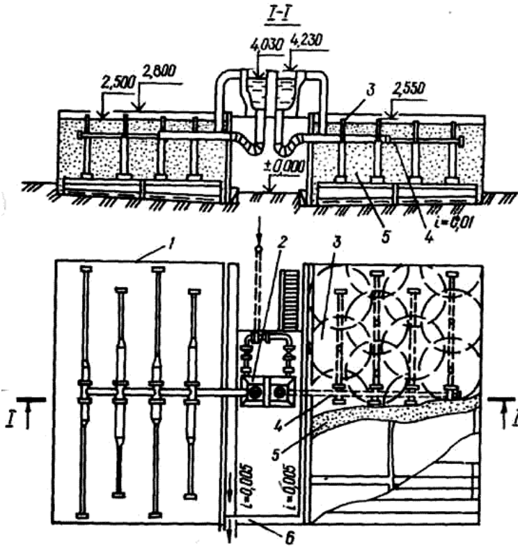
Рис. 6.9. Биофильтр: 1 – секция биофильтра; 2 – дозирующий бак; 3 – спринклер для орошения поверхности биофильтра; 4 – распределительный трубопровод; 5 – загрузка фильтра (фильтрующий материал); 6 – отвод очищенной сточной воды
