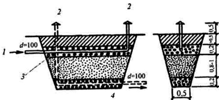
Рис. 6.17. Фильтрующая траншея:
