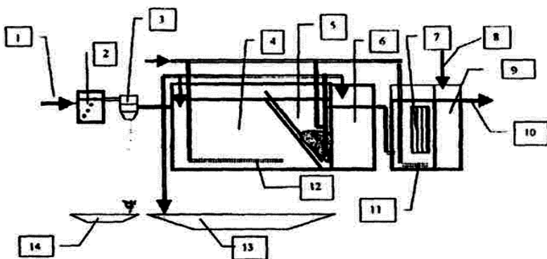
Рис. 6.22. Технологическая схема очистки сточных вод пропускной способностью 100–1000 м 3 /сут:
