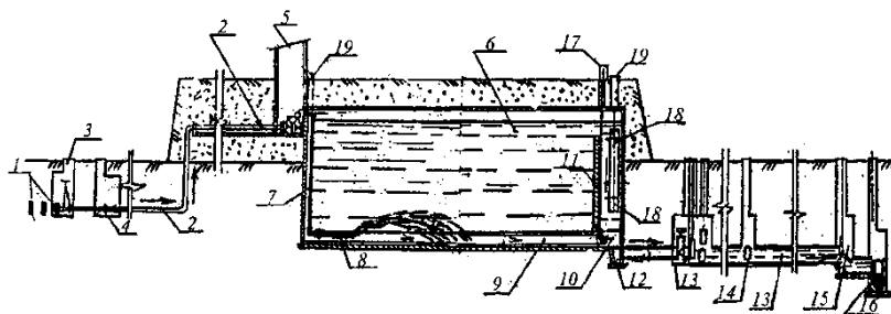
Рис. 5.7. Принципиальная высотная схема расположения APP по отношению к подводящему каналу НС: 1 – напорные водоводы от НС; 2 – трубопровод, подающий воду в галерею задвижек; 3 – колодец с задвижками; 4 – колодец с расходомером; 5 – галерея задвижек с регулирующими устройствами; 6 – аварийно-регулирующий резервуар; 7 – подающая в APP труба; 8 – эжектор с коническим насадком на подводящей к APP трубе; 9 – лотковая часть днища APP; 10 – водосборный канал; 11 – поперечная перегородка с водопропускным проемом; 12 – приямок опорожнения APP; 13 – труба опорожнения APP с запорно-регулирующими устройствами; 14 – канал опорожнения APP с колодцами на присоединении от смежных секций APP; 15 – водоизмерительный пост на канале опорожнения APP; 16 – колодец; 17 – фильтр-поглотитель; 18 – переливная труба APP; 19 – лазы в APP
