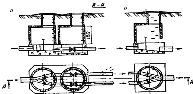
Рис. 4.14. Конструкция верхней (а) и нижней (б) камер дюкера
