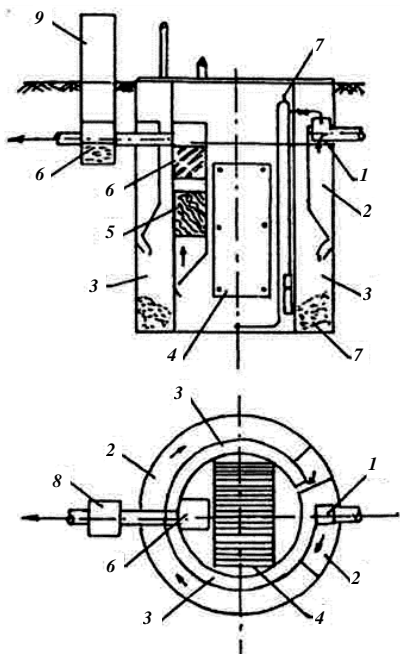
Рис. 6.19. Компактный блок очистных сооружений (КБС): 1 – решетка; 2 – остойный желоб; 3 – сбраживатель; 4 – аэротенк с плоскостным инертным наполнителем; 5 – осветлитель с тонкослойным отстаиванием; 6 – высокопористый фильтр; 7 – погружной насос с эжектором; 8 – контактный резервуар; 9 – шкаф системы КИПиА и обеззараживания
