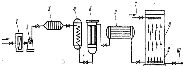
Рис. 6.25. Схема озонаторной установки:
