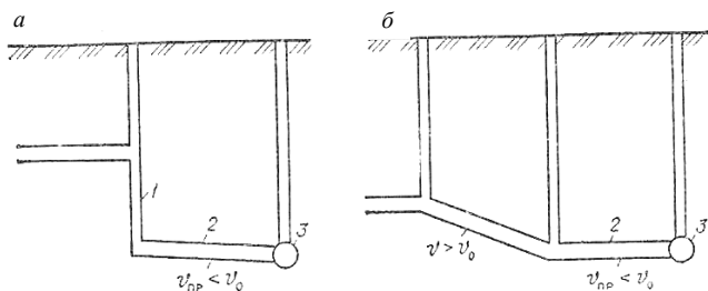
Рис. 4.21. Продольные профили боковых веток с перепадным колодцем (а) и участок с повышенным уклоном (б)
