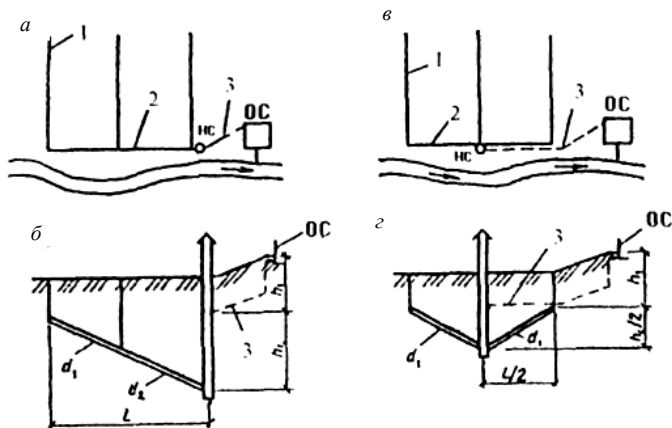
Рис. 5.2. Схемы водоотведения города с одной насосной станцией (а, в) и продольные профили главных коллекторов (б, з): 1 – коллекторы; 2 – главные коллекторы; 3 – напорные трубопроводы
