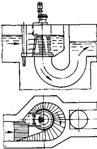
Рис. 6.5. Схема установки решетки-дробилки РД-600
