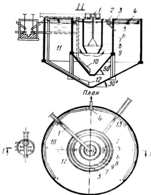
Рис. 6.11. Осветлитель-перегниватель:
