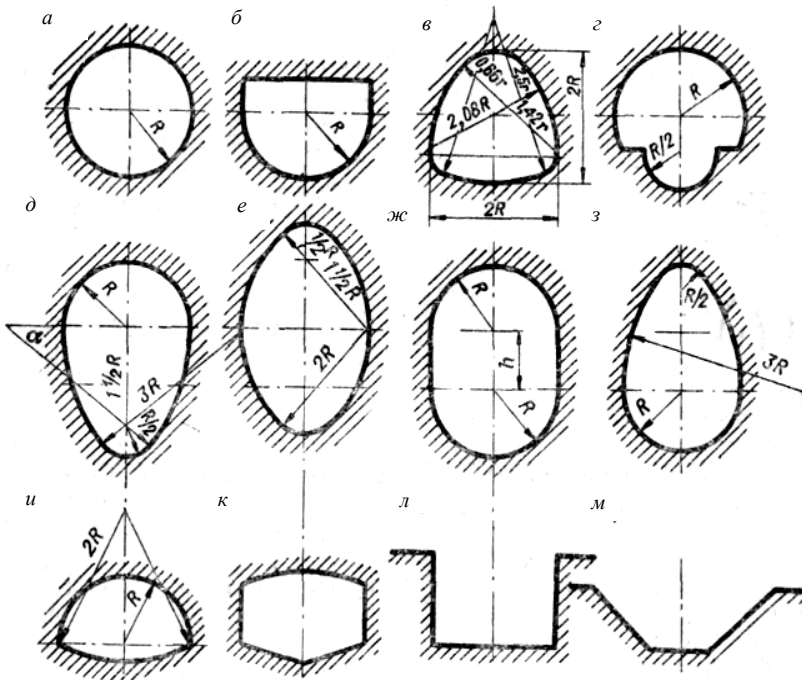
Рис. 4.2. Формы поперечного сечения водоотводящих труб, коллекторов и каналов: a – круглое; б – полукруглое; в – шатровое; г – банкетное; д – яйцевидное (овоидальное); е – эллиптическое; ж – полукруглое с прямыми вставками; з – яйцевидное перевернутое; и – лотковое; к – пятиугольное; л – прямоугольное; м – трапециевидное
