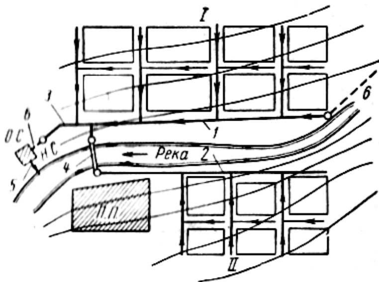
Рис. 4.4. Общая схема водоотведения населенного места: I, II – бассейны водоотведения; 1, 2 – главные коллекторы; 3 – отводящий главный загородный коллектор; 4 – дюкер; 5 – выпуск очищенных вод; б – напорный трубопровод; НС – насосная станция; ОС – очистные сооружения; ПП – промышленное предприятие
