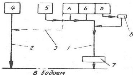
Рис. 4.19. Схема раздельной системы водоотведения с местными очистными установками: А, Б, В – цехи (производственные воды); 1 – сеть бытовых и загрязненных производственных сточных вод; 2 – сеть дождевых вод; 3 – выпуск условно чистых производственных вод; 4 – дождевые воды; 5 – бытовые воды; 6 – местные очистные установки; 7 – очистная станция
