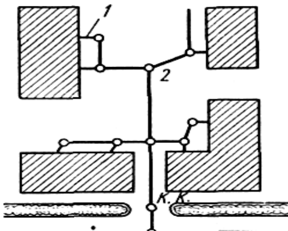
Рис. 4.9. Схема дворовой водоотводящей сети: 1 – выпуск из здания; 2 – смотровой колодец; К. К. – контрольный колодец
