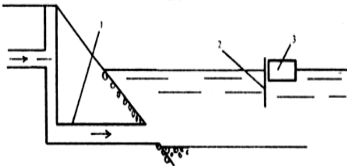
Рис. 4.25. Схема щитового заграждения: 1 – береговой выпуск дождевого коллектора; 2 – полупогружная перегородка; 3 – понтоны
