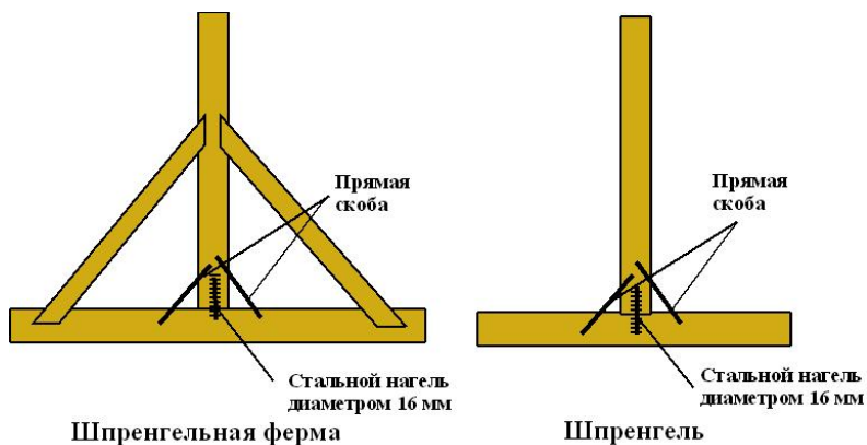
Рис. 102. Виды шпренгелей
