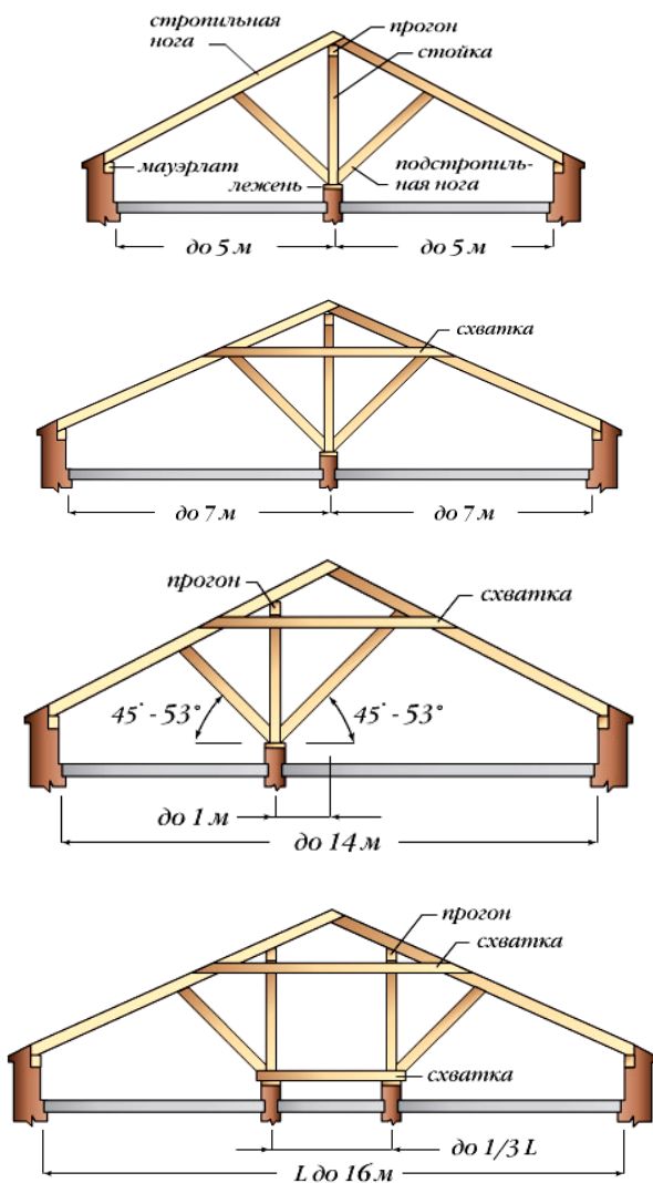
Рис. 93. Стропильные системы двухскатных крыш
