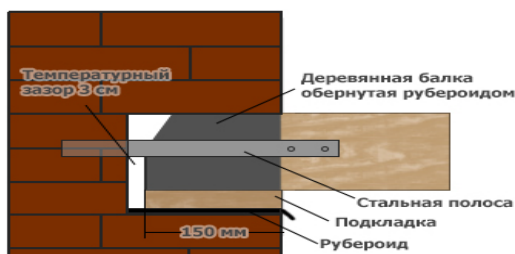
Рис. 63. Опирание деревянной балки на наружную стену
