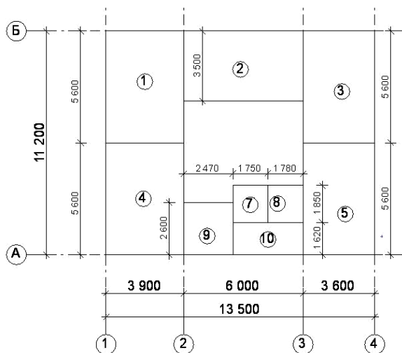
Рис. 12. Расстояние между осями «3» и «4» и параметры помещений 3, 5
