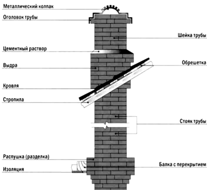
Рис. 23. Основные части дымовой трубы
