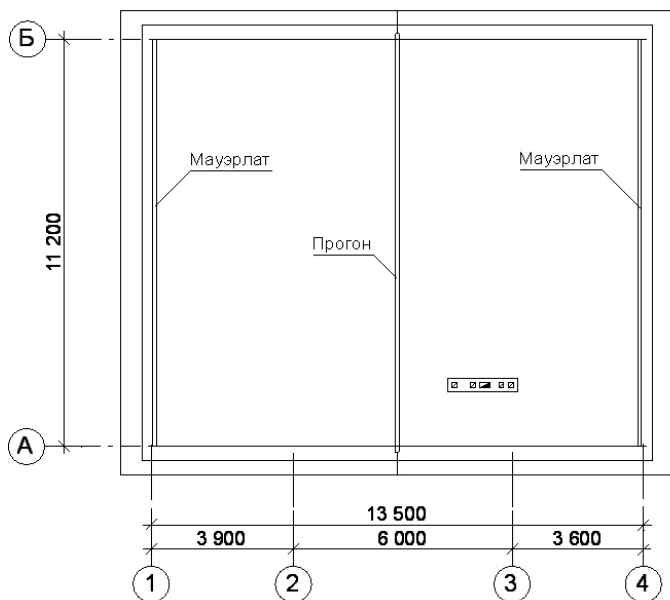
Рис. 145. Расположение мауэрлатов и прогона стропильной системы
