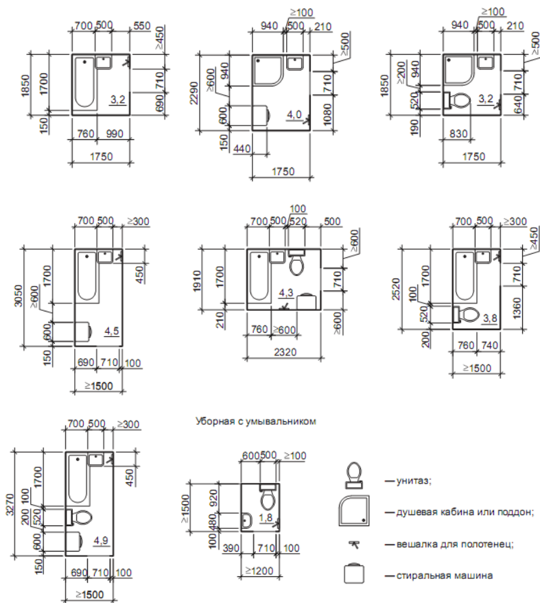
Рис. 1. Планировочные схемы санузлов и размеры санитарного оборудования
