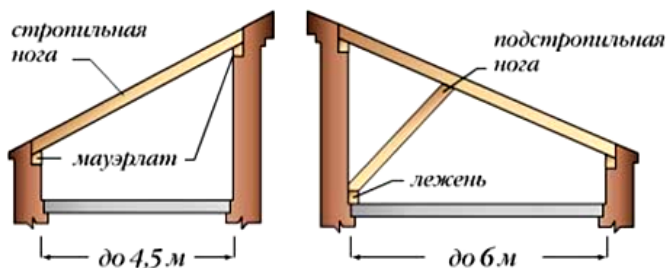
Рис. 90. Стропильная система односкатной крыши (однопролетные здания)
