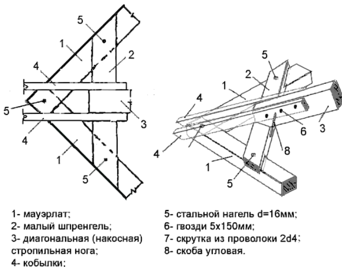
Рис. 154. Опорный узел крепления на мауэрлат диагональной стропильной ноги
