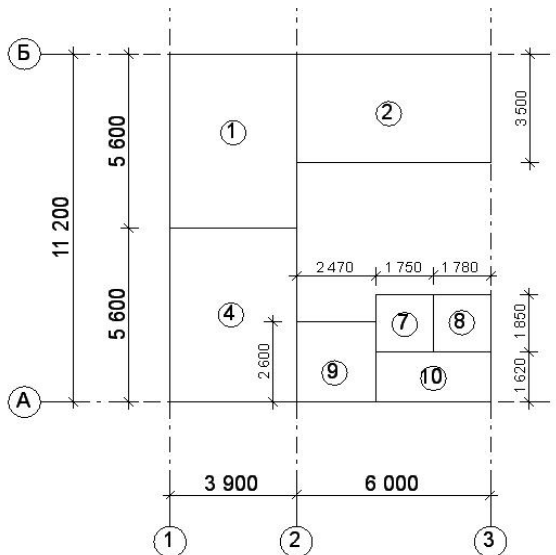
Рис. 11. Расстояние между осями «2» и «3» и параметры помещений 2, 7, 8, 9, 10
