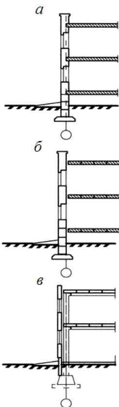
Рис. 4. Типы стен: a – несущая стена; б – самонесущая стена; в – ненесущая стена
