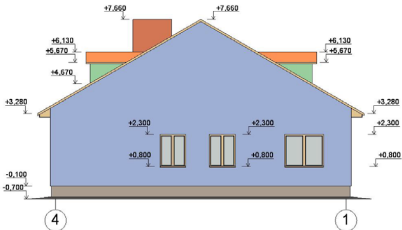
Рис. 181. Фасад 4–1
