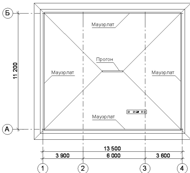
Рис. 149. Расположение мауэрлатов и прогона стропильной системы
