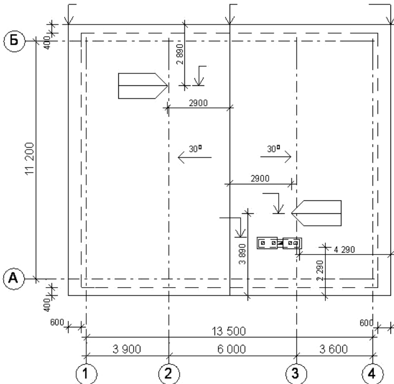
Рис. 135. План кровли двухскатной крыши (вариант 2)
