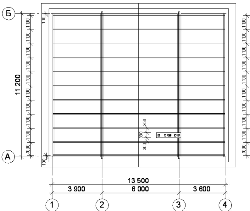
Рис. 141. Расположение рядовых стропил на плане
