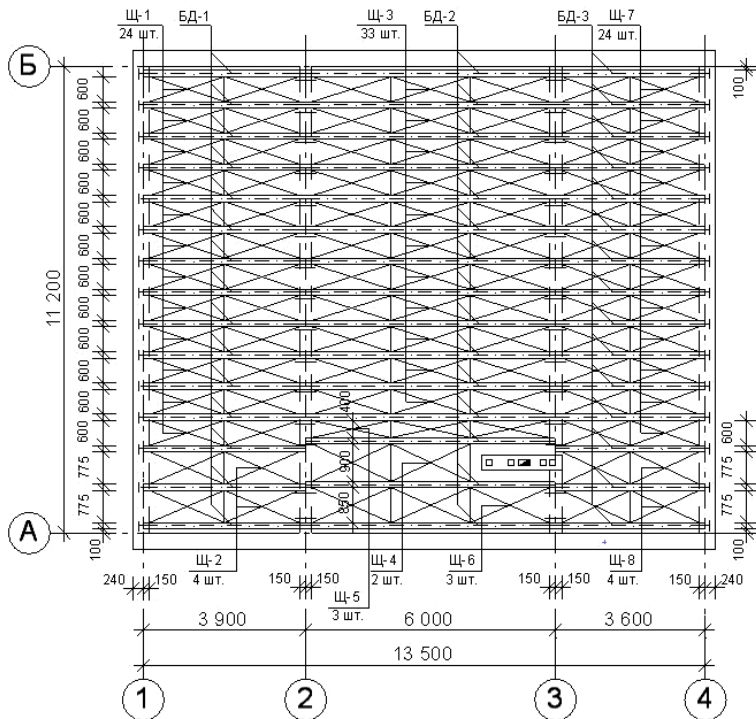
Рис. 69. Перекрытие по деревянным балкам
