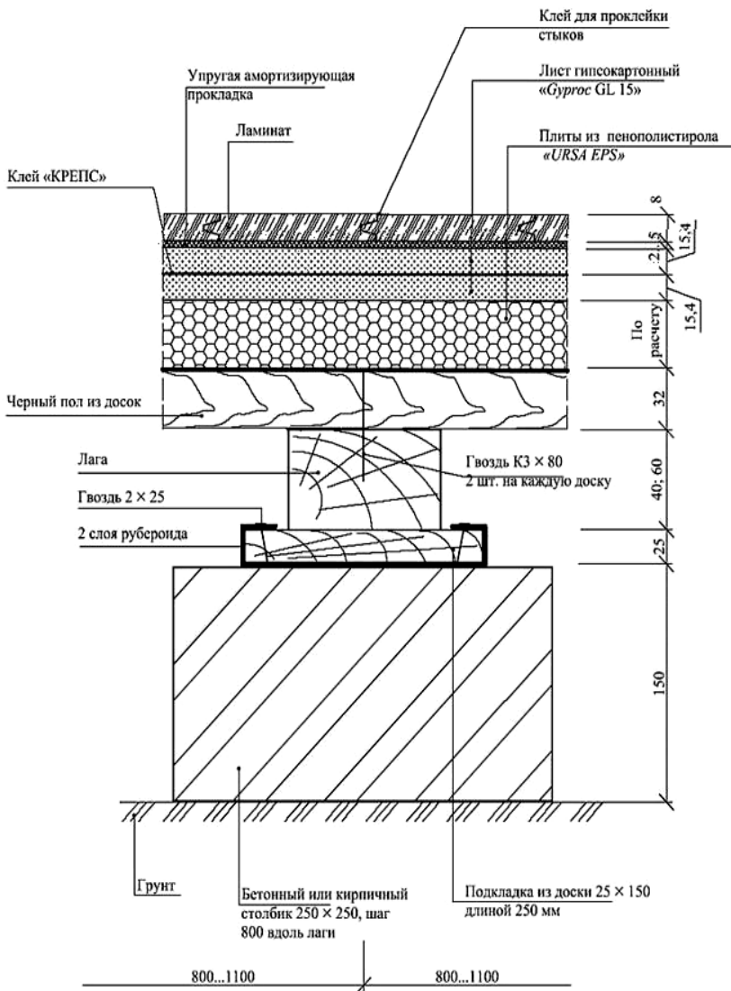
Рис. 172. Пол на столбиках с покрытием из ламината
