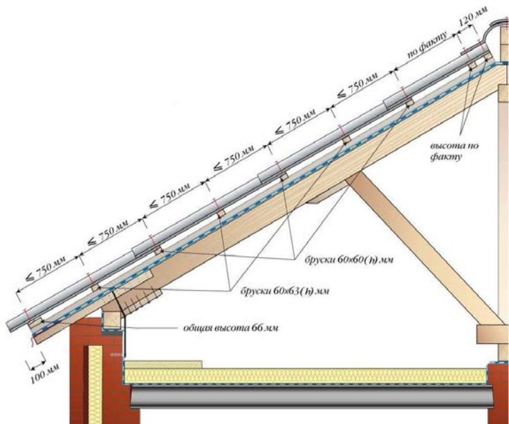
Рис. 120. Шаг обрешетки под шифер
