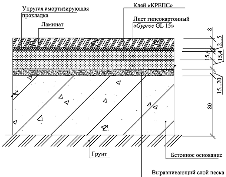
Рис. 170. Пол на бетонном основании с покрытием из ламината
