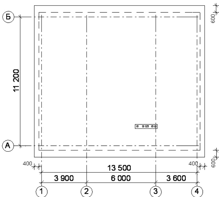
Рис. 131. Положение карнизного и фронтонного свесов
