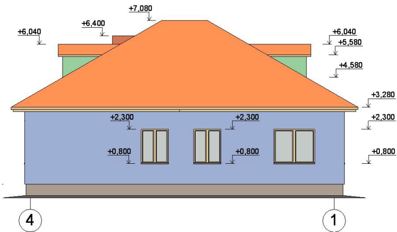
Рис. 185. Фасад 4–1
