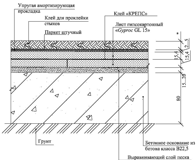
Рис. 168. Пол на бетонном основании с покрытием из паркетной доски
