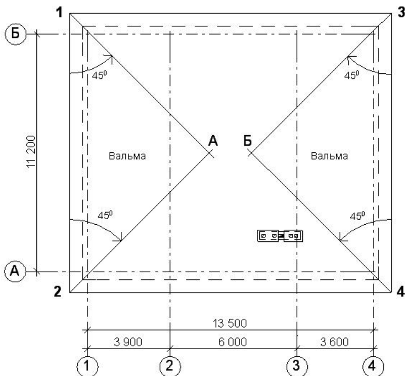
Рис. 137. Положение вальм на плане кровли
