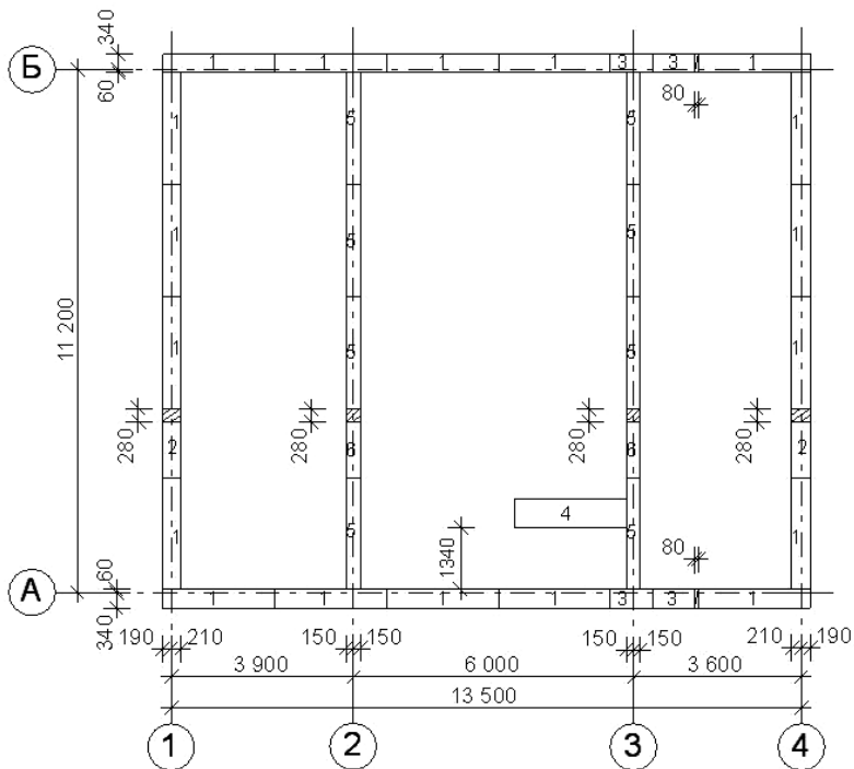
Рис. 45. Раскладка 1-го ряда фундаментных блоков
