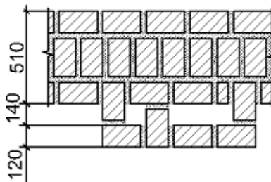
Рис. 19. Устройство вентиляционных и дымовых каналов в наружной стене
