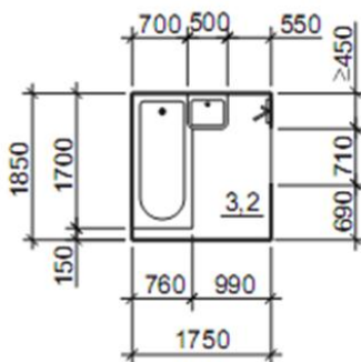
Рис. 10. Параметры помещения 7
