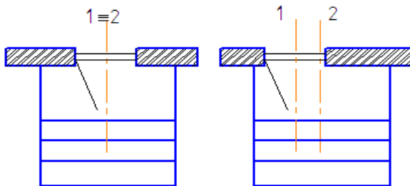
Рис. 158. Входная площадка перед наружной дверью: 1 – ось двери; 2 – ось крыльца
