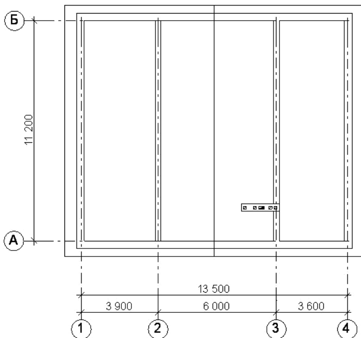
Рис. 139. Наружные и внутренние стены, контур кровли
