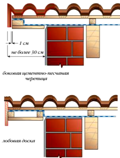
Рис. 114. Варианты оформления фронтового свеса крыши с покрытием из цементно-песчаной черепицы
