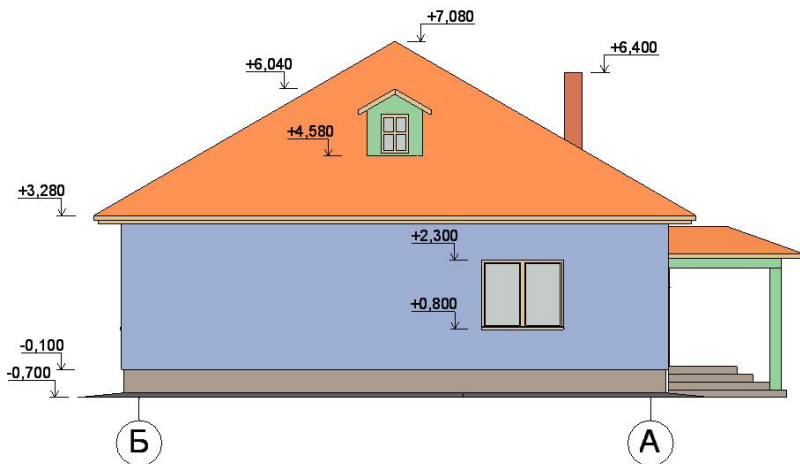
Рис. 187. Фасад Б–А
