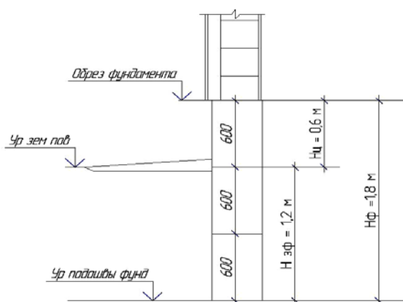
Рис. 40. Основные размеры фундамента
