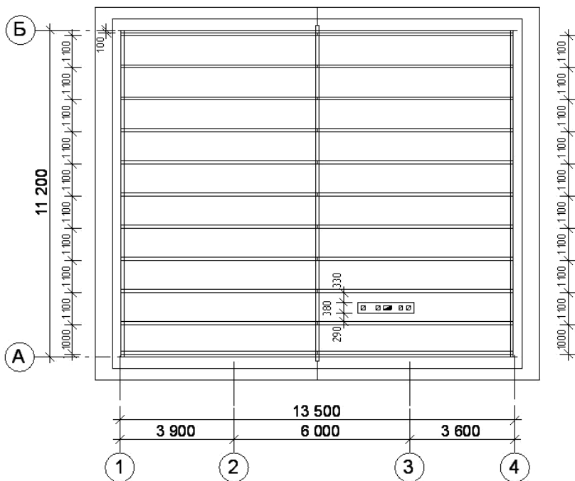
Рис. 146. Расположение рядовых стропил на плане
