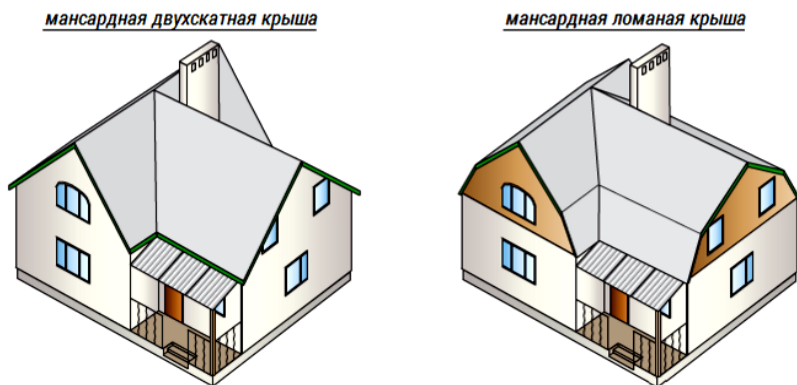
Рис. 86. Виды скатных крыш (мансардная)
