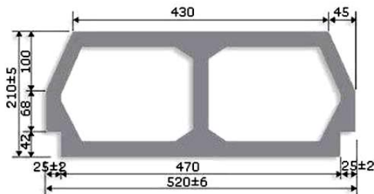
Рис. 55. Элемент сборно-монолитного перекрытия
