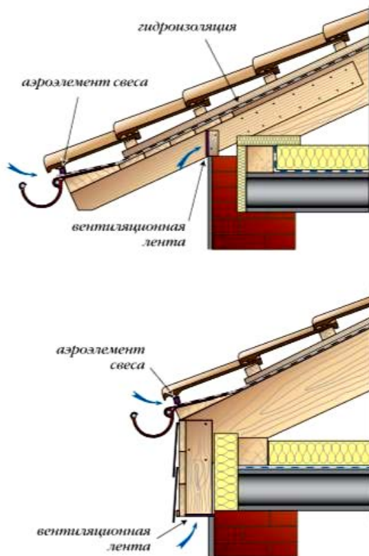
Рис. 113. Варианты устройства карнизного свеса крыши с покрытием из цементно-песчаной черепицы
