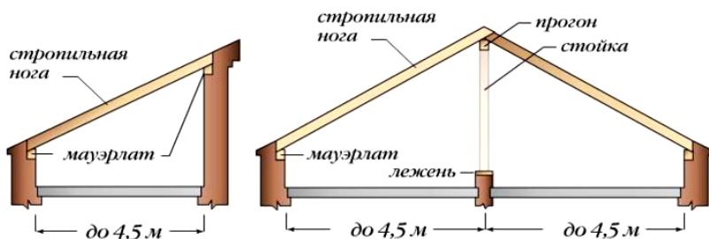
Рис. 98. Наслонные стропильные системы без подкосов
