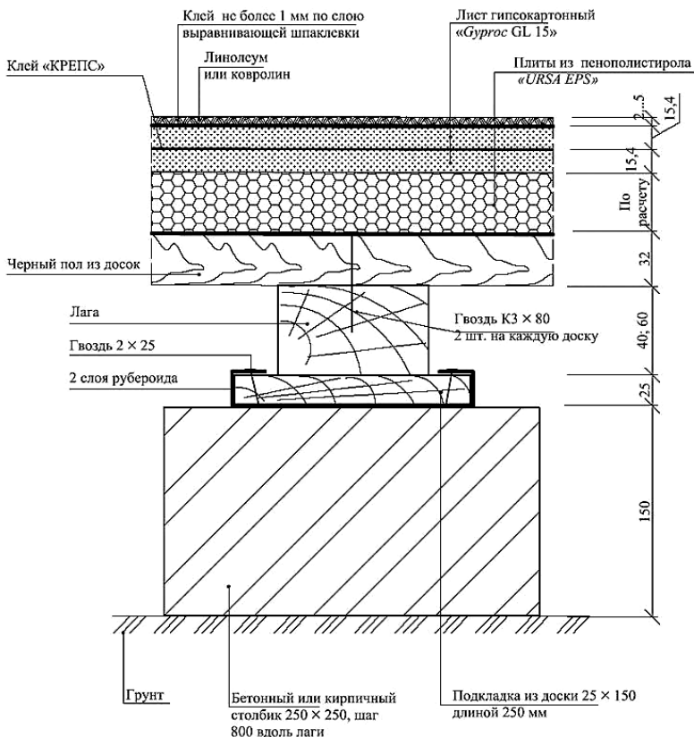
Рис. 166. Пол на столбиках с покрытием из линолеума
