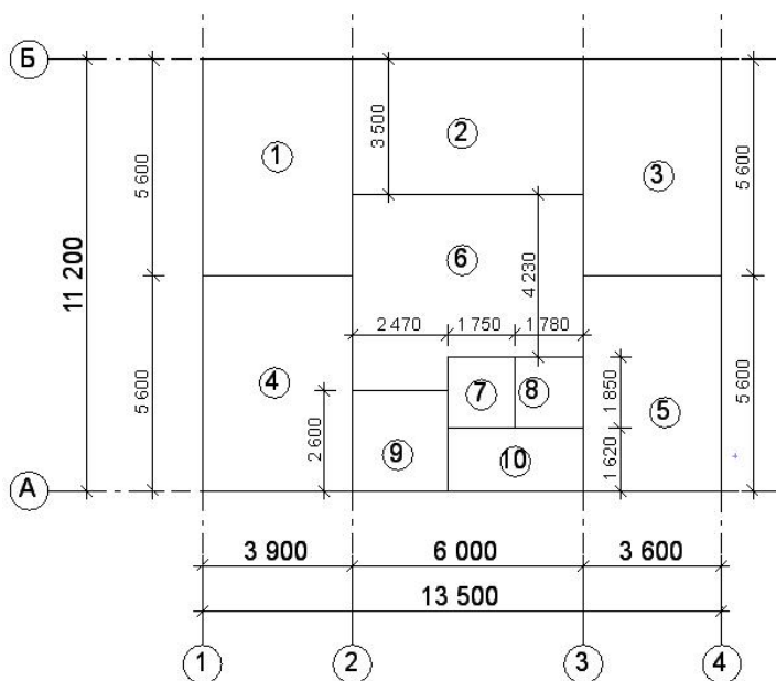
Рис. 13. Эскиз с назначенными размерами помещений
