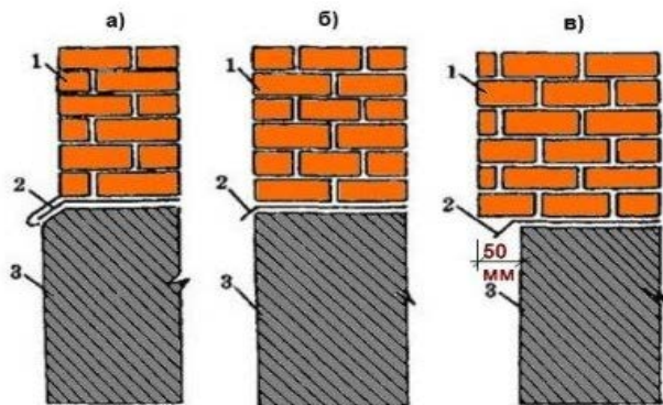
Рис. 41. Виды цоколя: а – выступающий цоколь; б – цоколь в одной плоскости со стеной; в – западающий цоколь; 1 – стена; 2 – гидроизоляция; 3 – надземная часть фундамента
