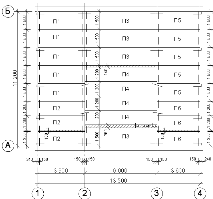
Рис. 62. Сборное железобетонное перекрытие
