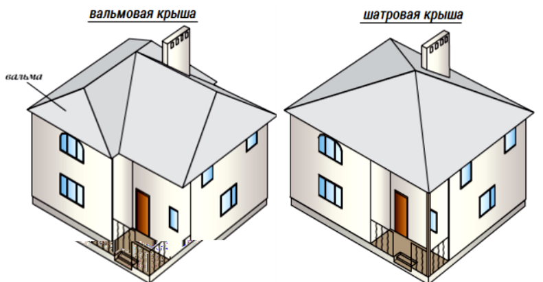
Рис. 85. Виды скатных крыш (вальмовая, шатровая)
