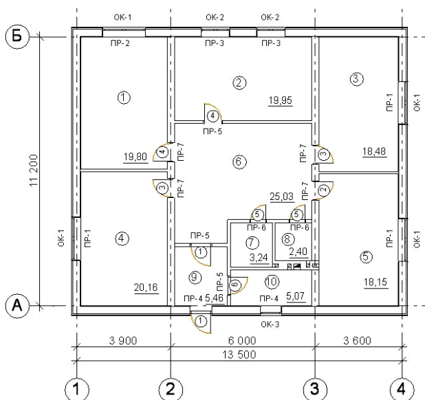
Рис. 129. План жилого дома
