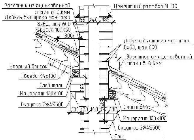
Рис. 156. Пропуск вентиляционного стояка через стропильную систему
