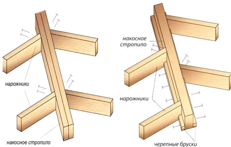
Рис. 155. Способы крепления нарожников к диагональной стропильной ноге
