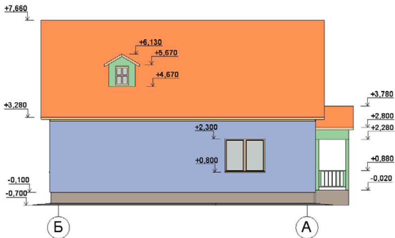
Рис. 183. Фасад Б-А
