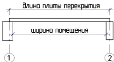
Рис. 8. Уменьшение площади помещения за счет величины опирания элементов перекрытия
