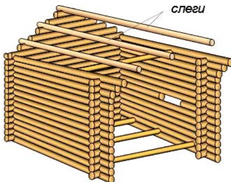
Рис. 89. Бесстропильная система
