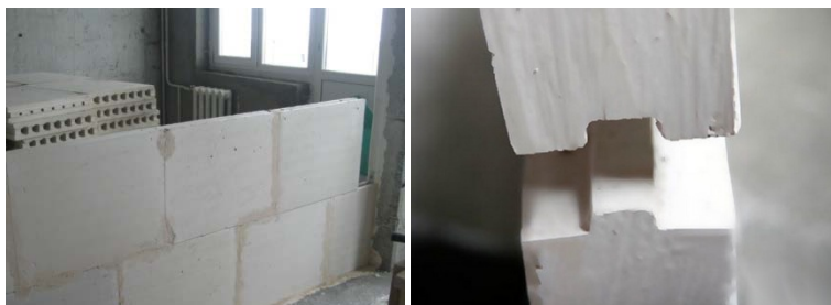
Рис. 25. Межкомнатные перегородки из пазогребневых гипсовых плит
