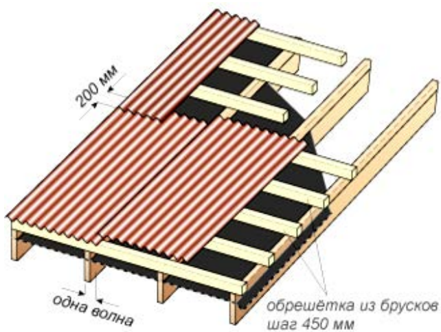
Рис. 123. Обрешетка под еврошифер с уклоном ската от 10 до 15°
