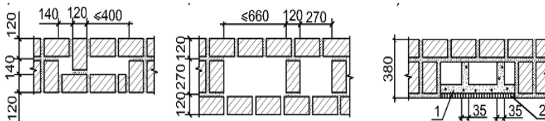
Рис. 18. Размеры вентиляционных и дымовых каналов в кирпичных стенах: 1 – гипсшлаковые блоки; 2 – штукатурка
