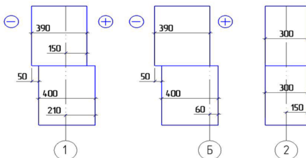
Рис. 42. Схемы к определению привязки фундамента
