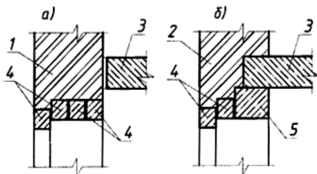
Рис. 82. Устройство проемов в каменных стенах с применением сборных железобетонных пере­мычек:
