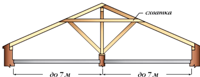
Рис. 99. Наслонные стропильные системы с подкосами и схваткой
