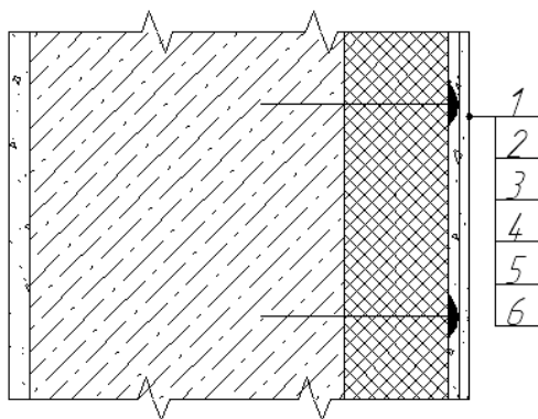
Рис. 16. Конструкция наружной стены жилого дома
