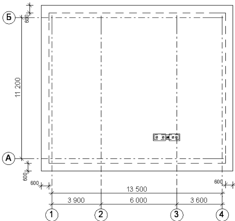
Рис. 136. Контур крыши с шириной свесов
