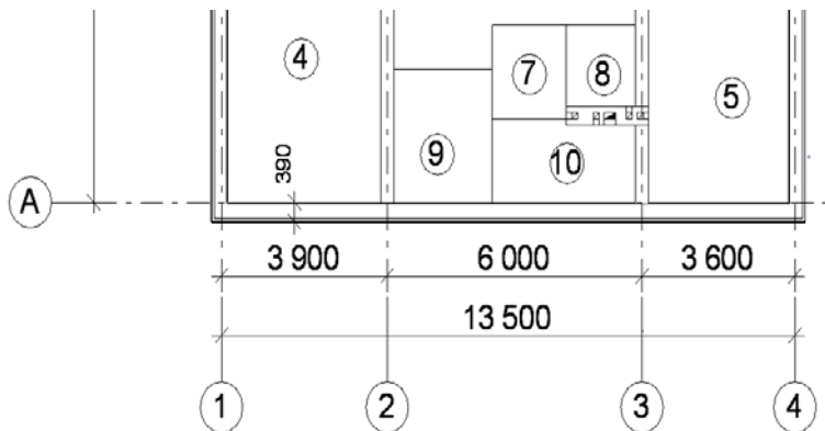
Рис. 33. Расположение вентиляционного стояка
