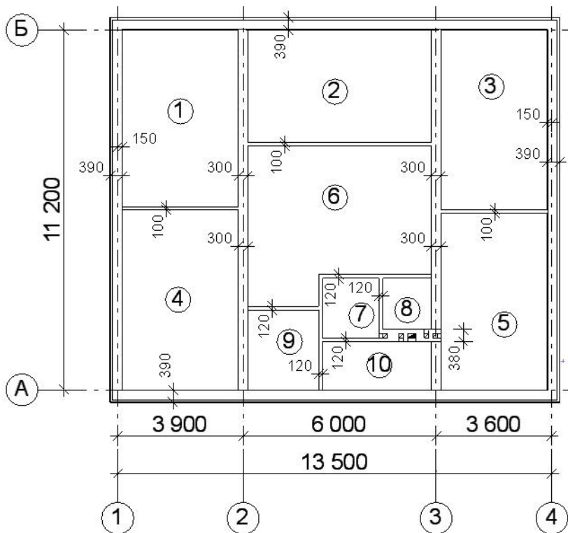
Рис. 35. Расположение межкомнатных перегородок
