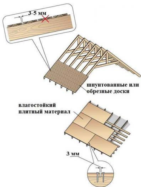
Рис. 117. Варианты устройства сплошной обрешетки под мягкую черепицу
