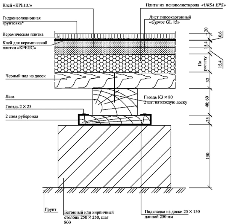
Рис. 173. Пол на столбиках с покрытием из керамической плитки
