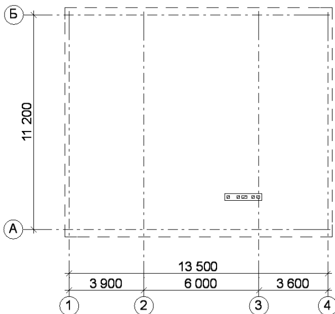
Рис. 130. Разбивочные оси с наружным контуром наружных стен
