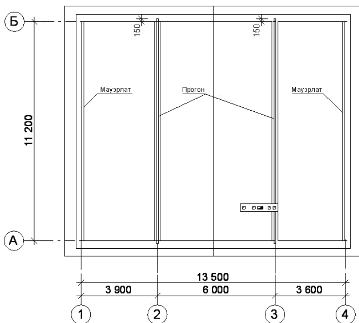
Рис. 140. Расположение мауэрлатов и прогонов стропильной системы
