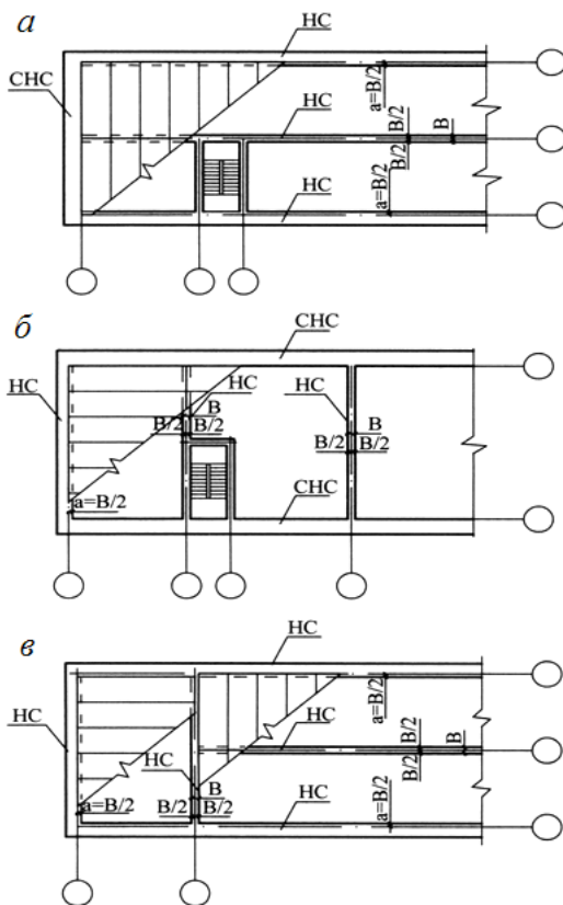
Рис. 5. Конструктивные схемы зданий: a – с продольными несущими стенами; б – с поперечными несущими стенами; в – с продольными и поперечными несущими стенами
