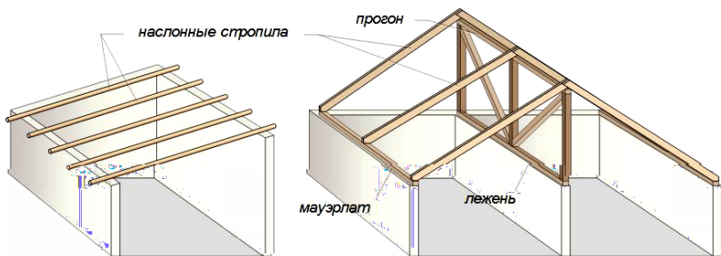
Рис. 87. Система наслонных стропил
