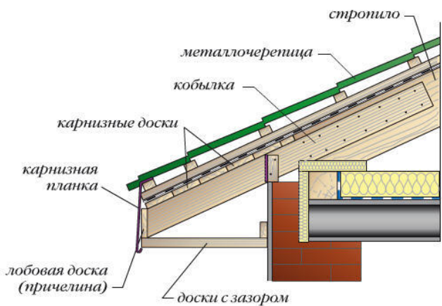
Рис. 106. Вариант устройства карнизного свеса крыши с покрытием из металлочерепицы
