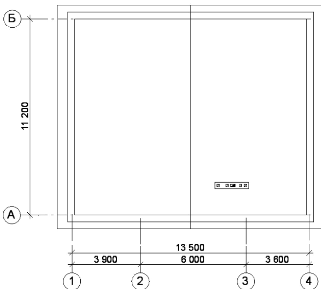
Рис. 144. Наружные стены, контур кровли
