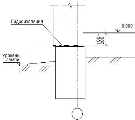
Рис. 161. Расстояние от пола первого этажа до обреза фундамента
