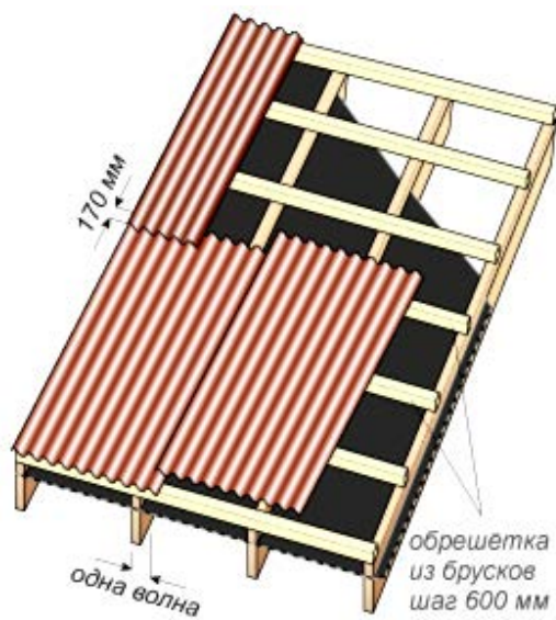
Рис. 124. Обрешетка под еврошифер с уклоном ската более 15°
