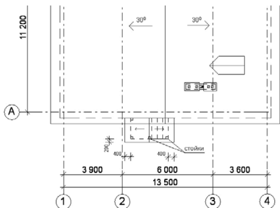
Рис. 165. Крыша над крыльцом с боковым расположением ступеней
