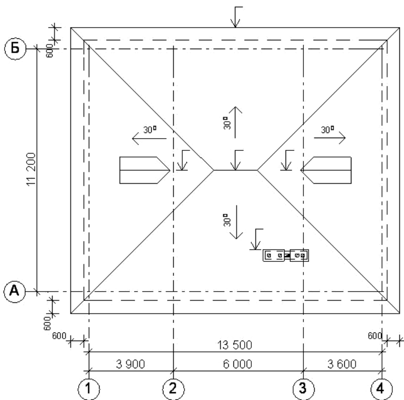
Рис. 138. План кровли вальмовой крыши
