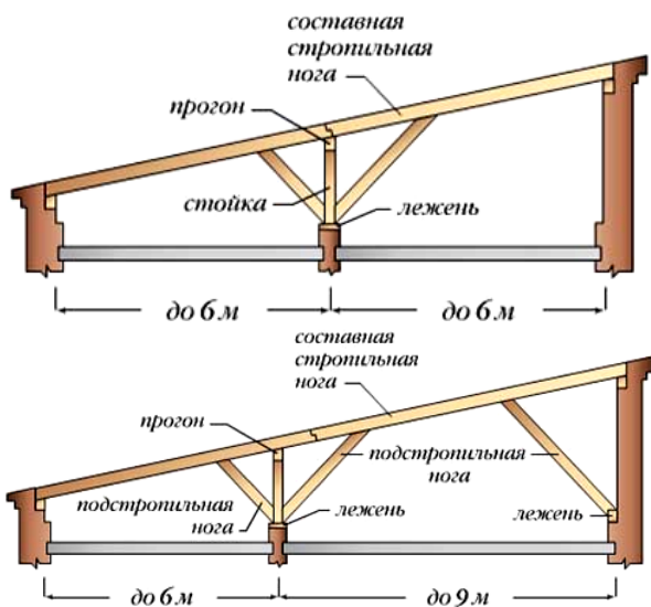
Рис. 91. Стропильная система односкатной крыши (двухпролетные здания)
