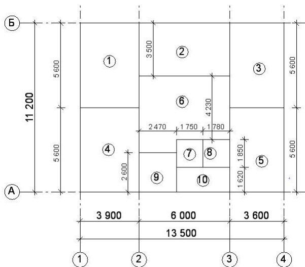
Рис. 29. Эскиз дома с разбивочными осями
