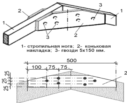
Рис. 142. Коньковая накладка
