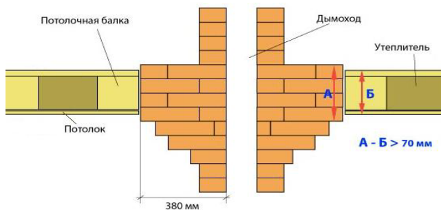
Рис. 68. Кирпичная разделка дымового канала
