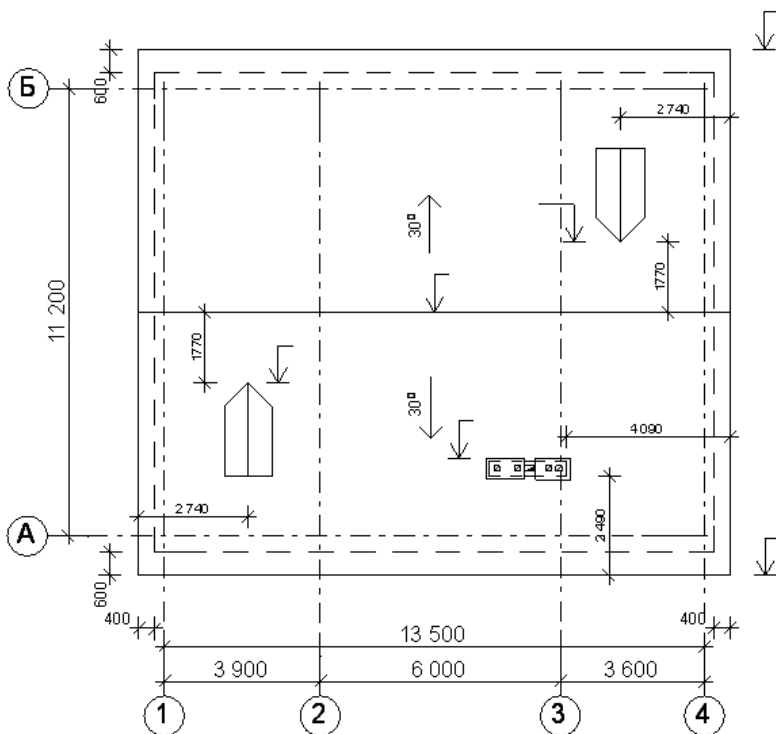
Рис. 134. План кровли двухскатной крыши
