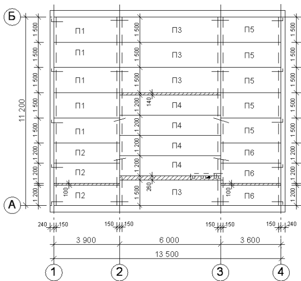
Рис. 176. Пример оформления плана сборного железобетонного перекрытия
