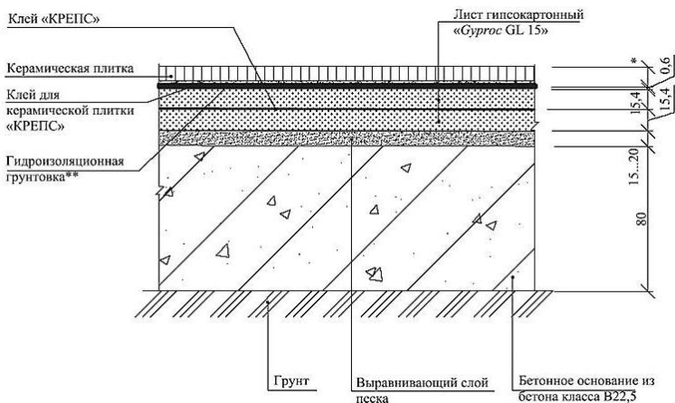
Рис. 171. Пол на бетонном основании с покрытием из керамической плитки
