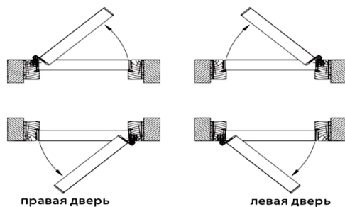
Рис. 77. Направления открывания дверей
