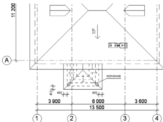
Рис. 164. Крыша над крыльцом с трехсторонним расположением ступеней
