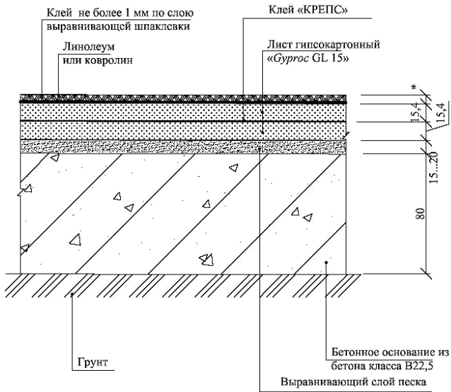
Рис. 167. Пол на бетонном основании с покрытием из линолеума
