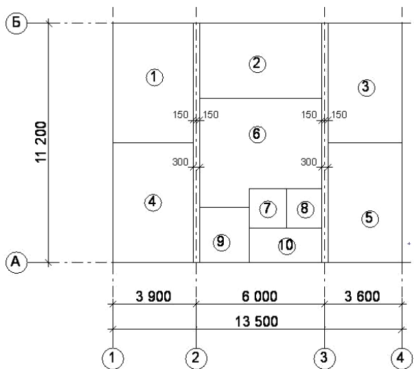
Рис. 30. Расположение и привязка внутренних стен
