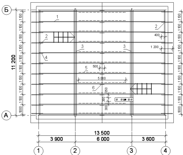
Рис. 143. План стропильной системы двухскатной крыши: 1 – стропильная нога; 2 – мауэрлат; 3 – прогон; 4 – кобылка; 5 – затяжка; 6 – накладка
