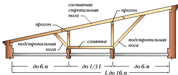
Рис. 92. Стропильная система односкатной крыши (трехпролетные здания)
