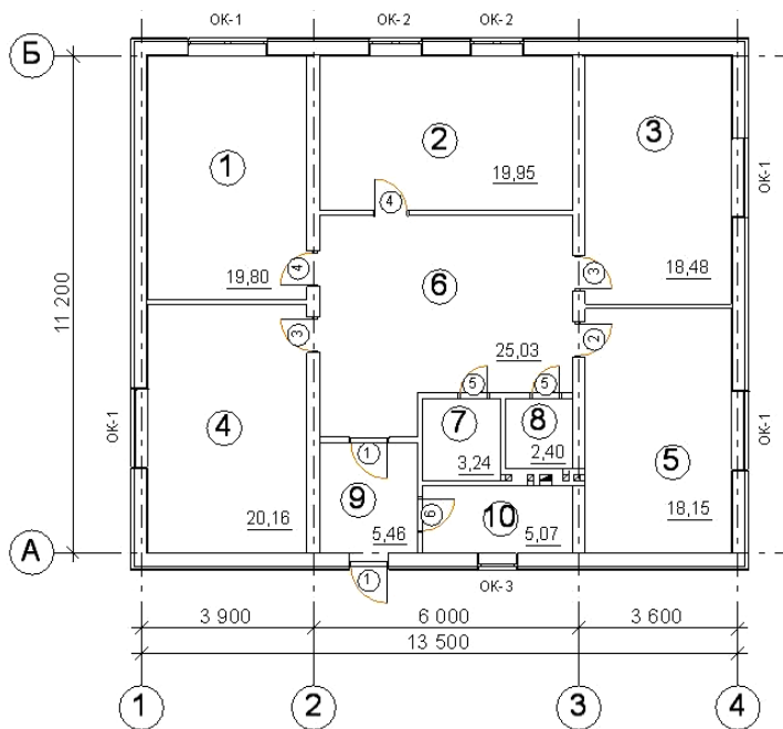
Рис. 78. План жилого дома с дверными проемами
