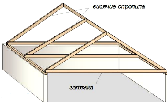
Рис. 88. Система висячих стропил
