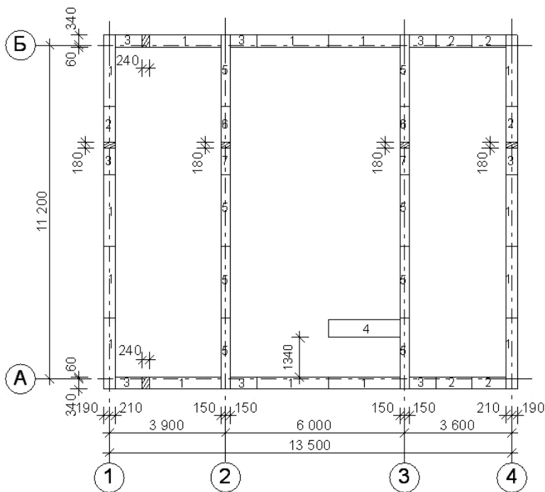
Рис. 47. Раскладка 2-го ряда фундаментных блоков
