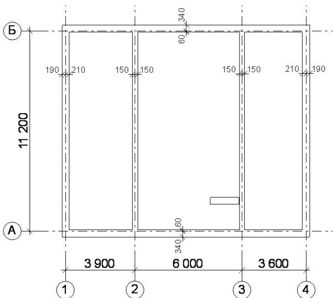
Рис. 44. План ленточного фундамента
