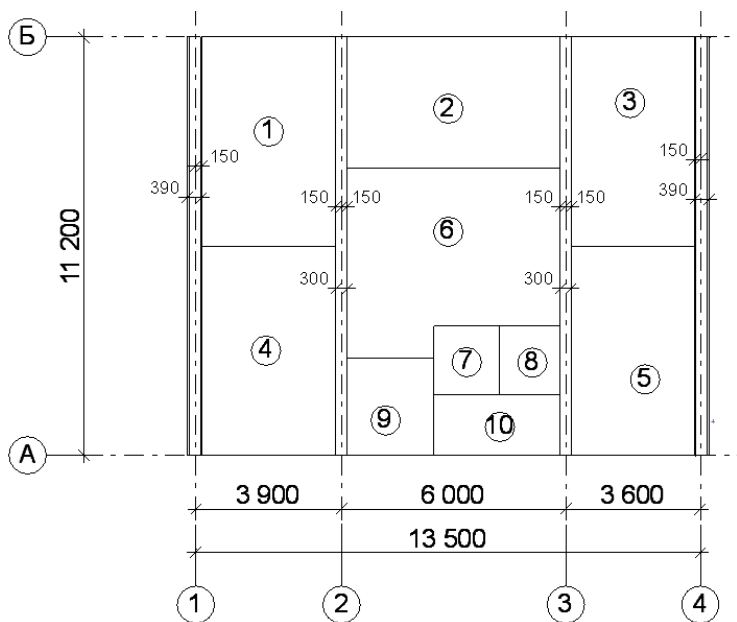
Рис. 31. Расположение и привязка наружных несущих стен
