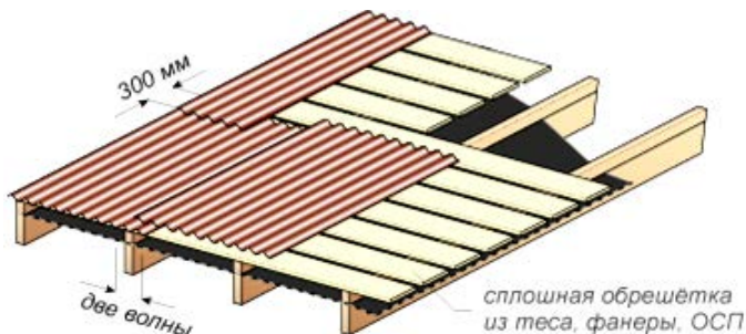
Рис. 122. Сплошная обрешетка под еврошифер с уклоном ската от 5 до 10°
