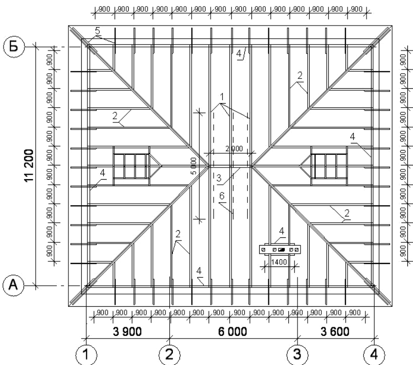
Рис. 178. Пример оформления плана стропильной системы
