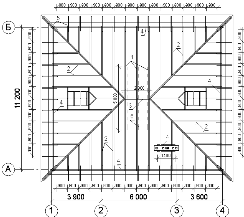
Рис. 157. План стропильной системы вальмовой крыши:
