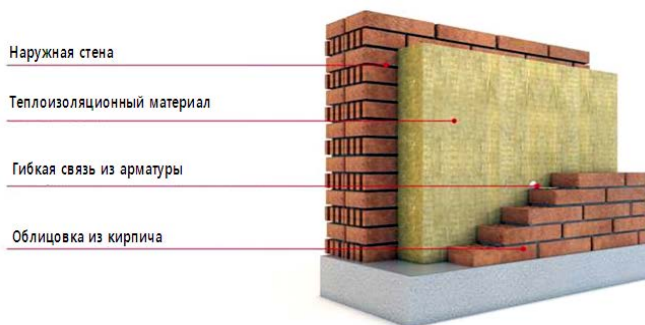
Рис. 14. Конструкция наружной стены с облицовкой кирпичом
