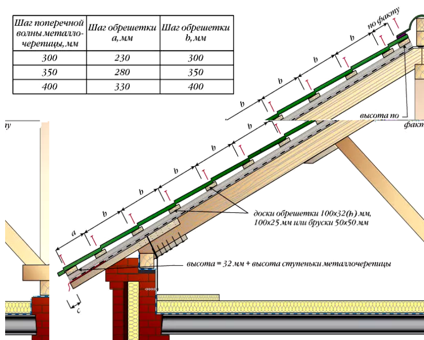
Рис. 105. Расчет шага обрешетки под кровлю из металлочерепицы
