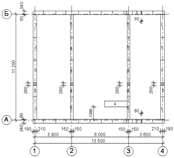
Рис. 177. Пример оформления плана фундамента
