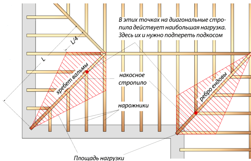
Рис. 101. Место установки дополнительных опор под диагональные стропила
