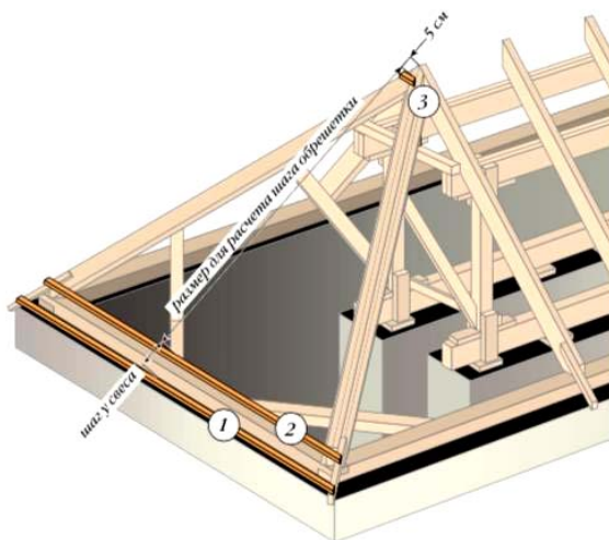
Рис. 112. Расчет шага обрешетки на вальмовой крыше
