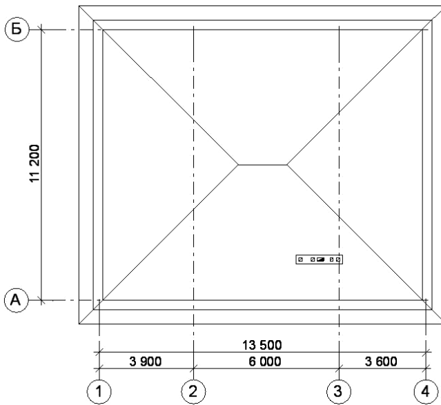
Рис. 148. Наружные стены, контур кровли
