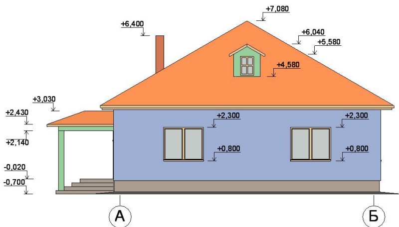
Рис. 186. Фасад А–Б
