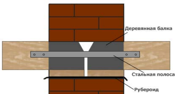
Рис. 64. Опирание деревянных балок на внутреннюю стену
