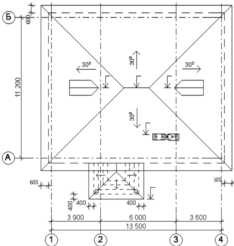
Рис. 179. Пример оформления плана кровли
