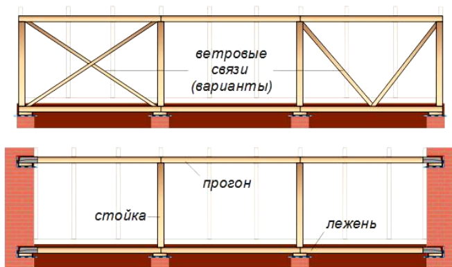
Рис. 97. Варианты подстропильных конструкций
