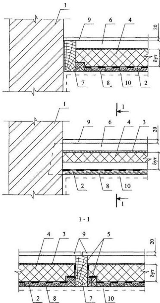
Рис. 66. Элементы чердачного перекрытия по деревянным балкам: 1 – наружная стена; 2 – пароизоляция; 3 – армофол тип С, Пенофол 2000 С-03 с перфорацией; 4 – минераловатные плиты; 5 – деревянные бруски; 6 – замкнутая воздушная прослойка; 7 – деревянная балка перекрытия; 8 – деревянный щит; 9 – цементно-стружечная плита d = 20 мм; 10 – штукатурка
