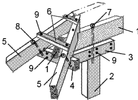
Рис. 151. Опорный узел крепления диагональных стропильных ног на коньковый прогон без опоры на подкосы для вальмового ската: 1 – прогон; 2 – стойка под прогон; 3 – боковые накладки; 4 – торцевая накладка; 5 – диагональные стропильные ноги; 6 – ригель обрешетки; 7 – стальной штырь d = 10 \dots 12 мм; 8 – болт М16; 9 – гвозди
