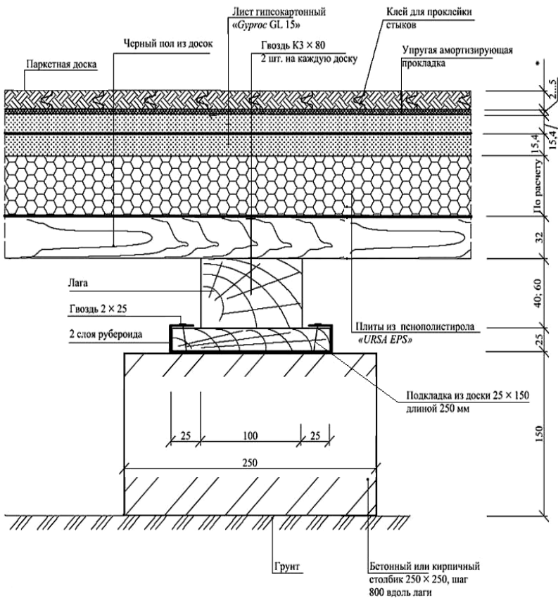
Рис. 169. Пол на столбиках с покрытием из паркетной доски
