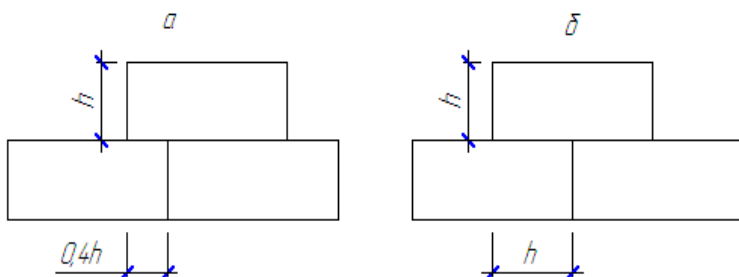
Рис. 46. Минимальная глубина перевязки вертикальных швов фундаментных стеновых блоков: a – при малосжимаемых грунтах; б – при сильносжимаемых грунтах
