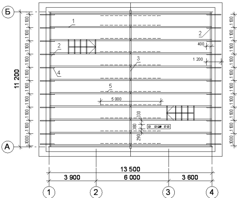
Рис. 147. План стропильной системы двухскатной крыши:
