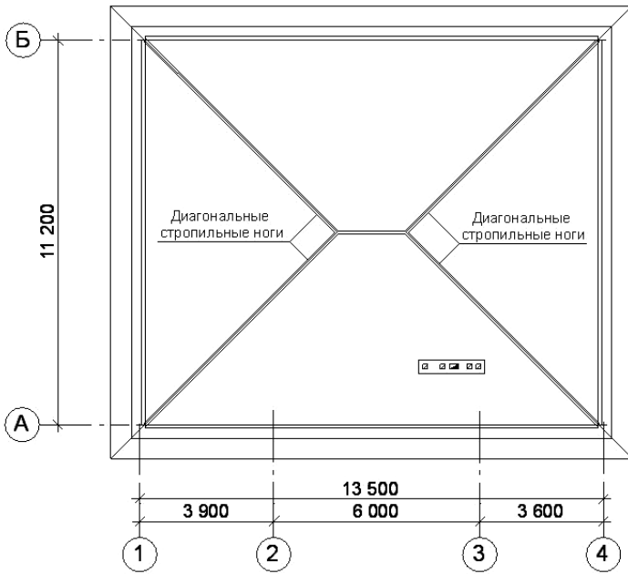
Рис. 150. Расположение диагональных стропильных ног на плане
