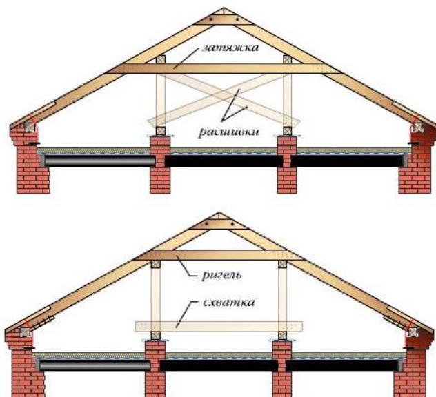
Рис. 100. Стропильная система для зданий с двумя внутренними несущими стенами
