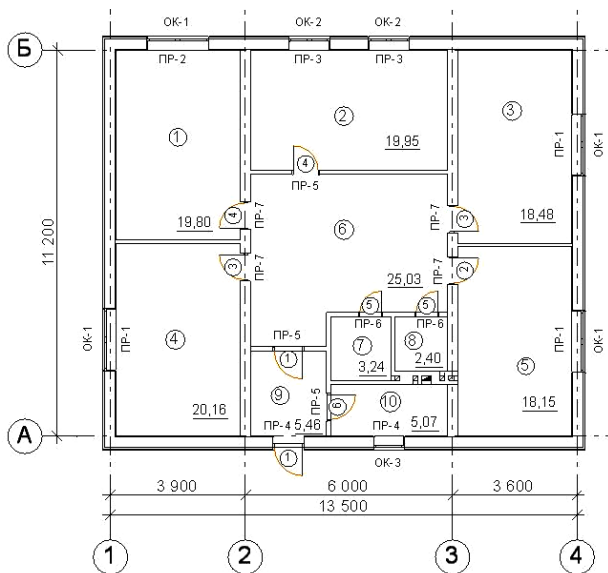
Рис. 81. Обозначение проемов на плане
