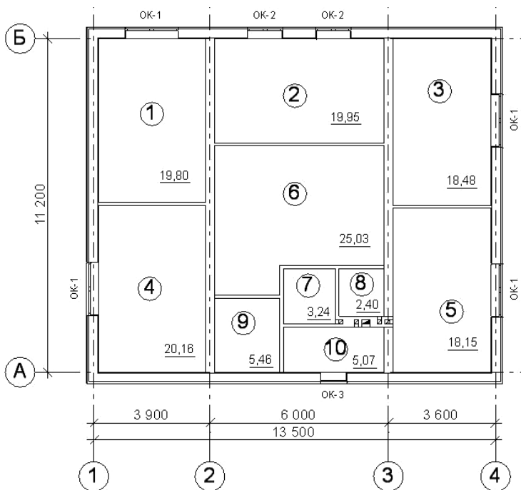
Рис. 76. План жилого дома с оконными проемами
