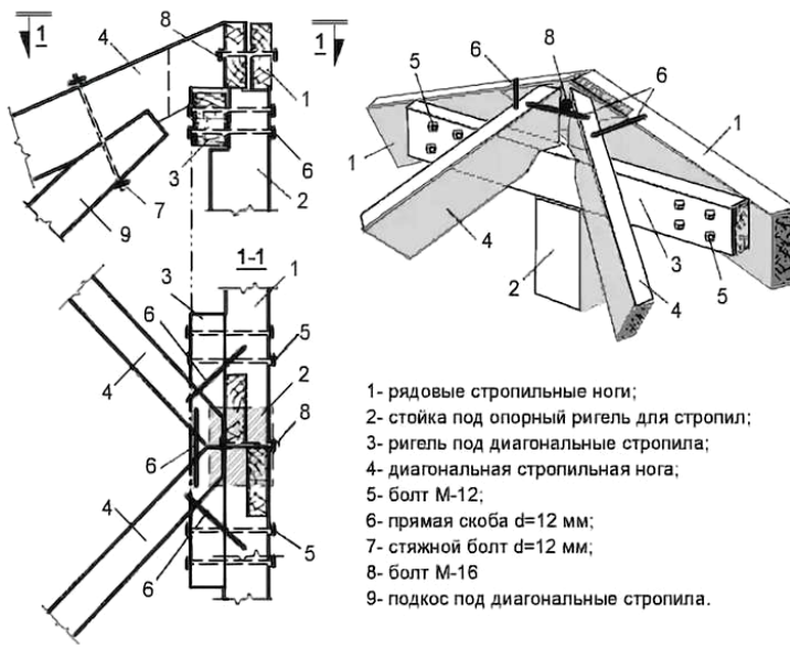
Рис. 153. Опорный узел крепления диагональных стропильных ног на ригель и боковые подкосы при отсутствии конькового прогона
