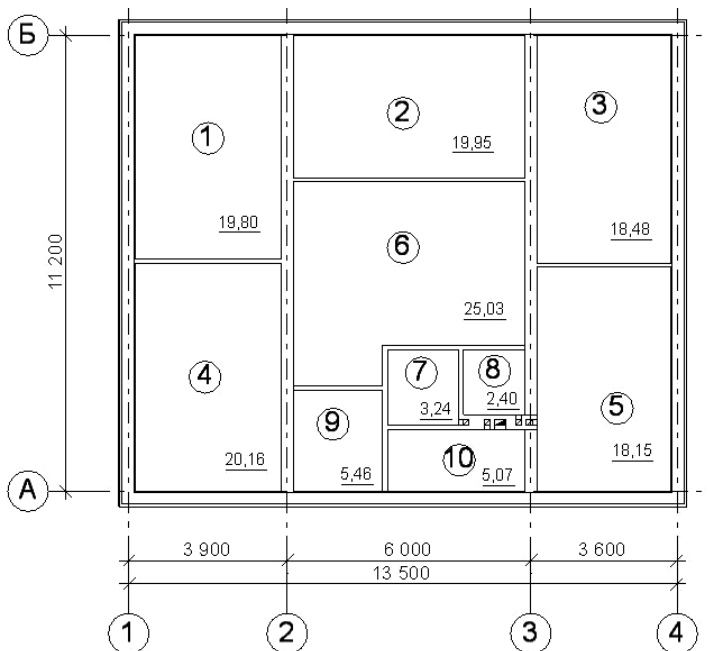
Рис. 72. План проектируемого дома:
