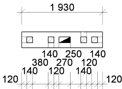
Рис. 34. Параметры вентиляционного стояка жилого дома
