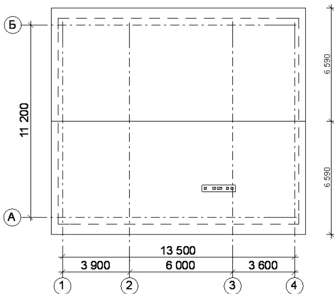
Рис. 133. Положение конька крыши
