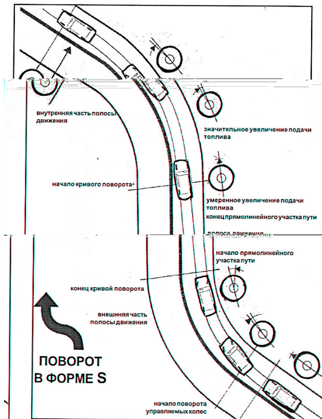
Рис. 6.23. Поворот в форме S
