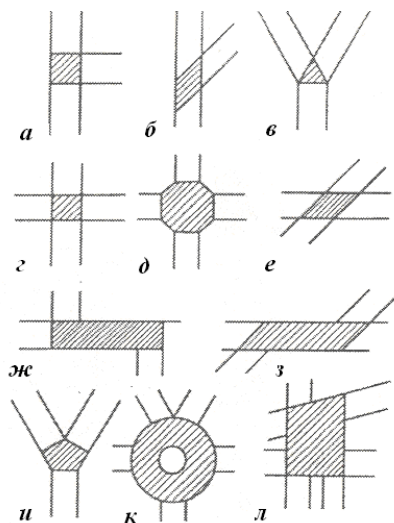
Рис. 2.5. Формы пересечения дорог
