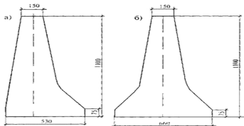
Рис. 2.18. Ограждение железобетонное парапетного типа: а – в одностороннем (блок Бс-0) б – в двустороннем исполнении (блок Бс-Д)
