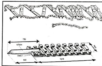
Рис. 6.10. Цепи с косым расположением траков
