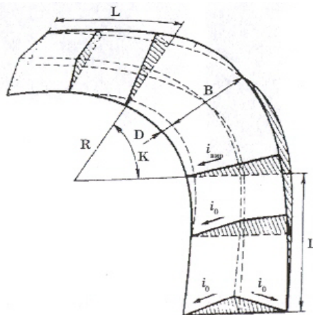
Рис. 2.1. Схема виража: i_{\text{вир}} и i_0 – поперечные уклоны соответственно на вираже и на переходной кривой; L – участок отгона виража и переходная кривая; D – уширение; K – круговая кривая; B – ширина проезжей части; R – радиус круговой кривой
