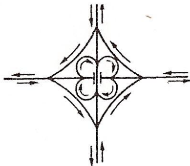
Рис. 2.13. Схема пересечения в разных уровнях по типу «клеверный лист»
