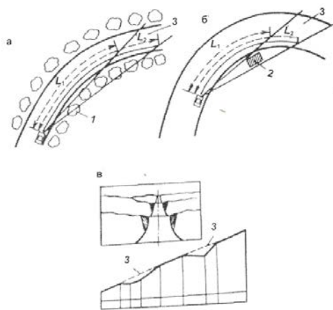
Рис. 6.3. Схемы ограничения обзорности: а – неправильное расположение посадок; б – неправильное расположение павильона на автобусной остановке; в – устройство частых переломов в продольном профиле (вид дороги в плане и профиле); 1 – посадки; 2 – павильон; 3 – зоны отсутствия обзорности; L 1 и L 2 – фактическое и необходимое расстояние обзорности соответственно
