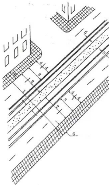
Рис. 2.4. Элементы улицы: 1 – общая ширина улицы; 2 – проезжая часть; 3 – проезжая часть для транспортных средств; 4 – полоса движения; 5 – трамвайный путь; 6 – тротуар; 7 – разделительная полоса
