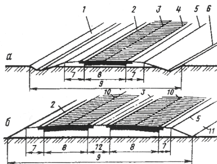
Рис. 2.2. Элементы поперечного профиля дороги: а – с одной проезжей частью; б – с двумя проезжими частями и разделительной полосой; 1 – внешний откос канавы; 2 – укрепленная полоса обочины; 3 – ось дороги; 4 – кромка проезжей части; 5 – бровка земляного полотна; 6 – внутренний откос; 7 – обочина; 8 – проезжая часть; 9 – земляное полотно; 10 – ось проезжей части; 11 – откос насыпи; 12 – разделительная полоса
