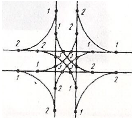
Рис. 2.6. Конфликтные точки на пересечениях дорог в одном уровне: 1 – разделение транспортных потоков; 2 – слияние транспортных потоков; 3 – пересечение транспортных потоков
