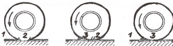
Рис. 6.24. Этапы возникновения аквапланирования: 1 – пленка воды на покрытии; 2 – зона контакта между шиной и покрытием; 3 – водяной клин
