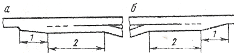
Рис. 2.15. Схема переходно-скоростных полос: а – торможения; б – разгона; 1 – отгон переходно-скоростной полосы; 2 – длина полосы для разгона и торможения
