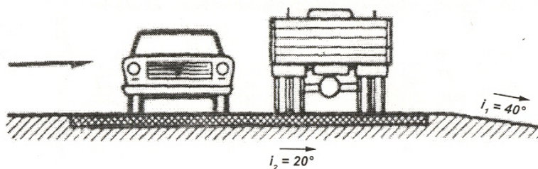
Рис. 6.25. Направление наиболее вероятного смещения транспортного средства при заносе на проезжей части с односкатным профилем: i_1 – поперечный уклон обочины; i_2 – поперечный уклон проезжей части
