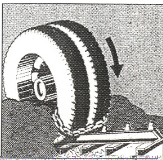
Рис. 6.15. Рейковый мат с клином
