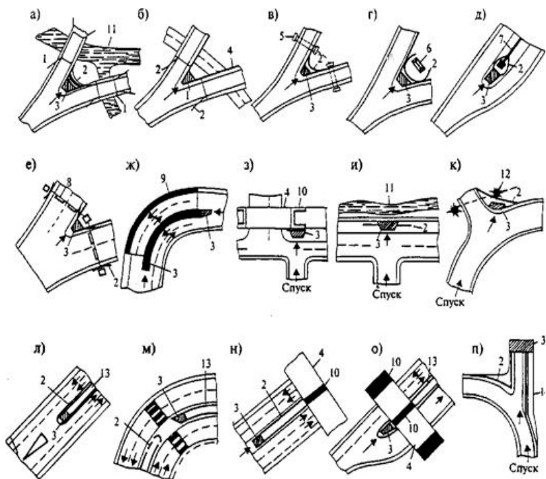
Рис. 2.20. Размещение ограждений первой группы у препятствий и на опасных участках дорог: 1 – мост; 2 – направляющие ограждения; 3 – останавливающие ограждения; 4 – путепровод; 5 – водопропускная труба; 6 – здание; 7 – подпорная стенка; 8 – рамная опора информационно-указательных знаков; 9 – тоннель, селепровод или снегозащитная галерея; 10 – опора путепровода; 11 – река; 12 – опора высоковольтных линий электропередачи; 13 – разделительная полоса; 14 – противоаварийный съезд
