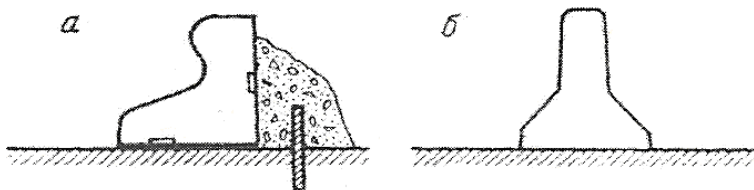
Рис. 2.22. Профили высоких бетонных ограждений: a – «Триэф»; б – «Нью-Джерси»
