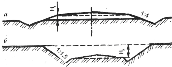
Рис. 2.3. Поперечные профили насыпи (а) и выемки (б): H_1 – высота насыпи; H_2 – глубина выемки
