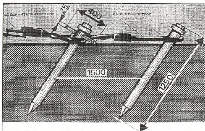
Рис. 6.16. Упоры для вытаскивания транспортного средства
