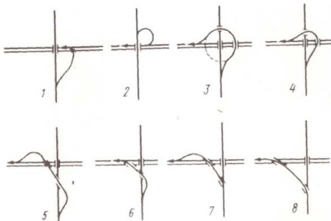
Рис. 2.8. Типы левоповоротных съездов на транспортных развязках: 1 – съезд на неполных развязках; 2 – петлевой съезд на развязках типа «клеверный лист»; 3, 4 – съезды с использованием распределительного кольца; 5, 6 – полупрямые съезды; 7, 8 – прямые съезды
