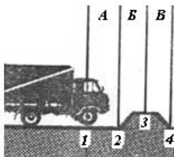
Рис. 6.4. Схема преодоления препятствия в виде возвышения над поверхностью дороги
