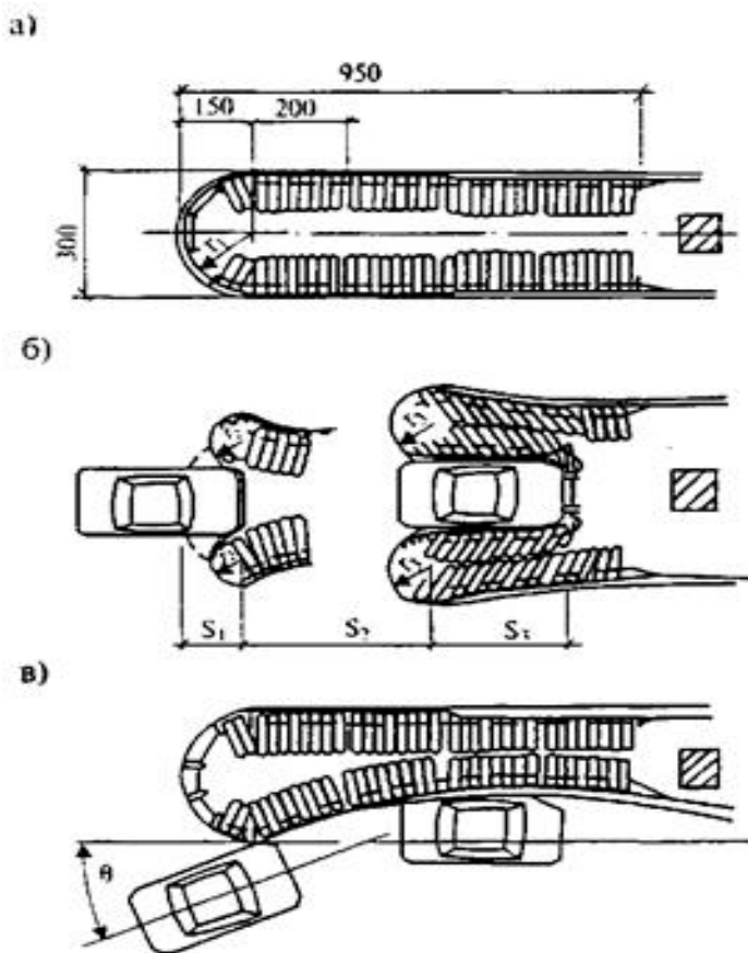
Рис. 2.19. Схема устройства и работы фронтально-бокового ограждения 211ДО-Н при фронтальном и боковом наездах: а – схема устройства ограждения; б – характер деформации ограждения при фронтальном наезде; в – то же при боковом
