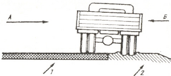
Рис. 6.26. Направление возможного заноса при резком увеличении скорости ( A ) и резком торможении ( B ): 1 – покрытие; 2 – обочина
