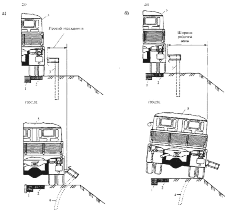
Рис. 2.21. Динамический прогиб ограждения: 1 – проезжая часть; 2 – краевая полоса; 3 – недеформированное ограждение; 4 – деформированное ограждение; 5 – автомобиль
