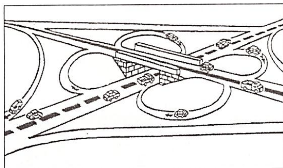
Рис. 2.12. Пересечение типа «клеверный лист»
