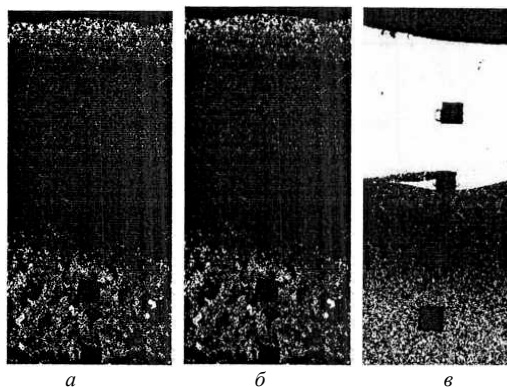
Рис. 3. Фотографии микроструктуры различных покрытий после МЭУ и лазерной обработки: a – Fe-Ti ( \times 50 ); б – Fe-5%V ( \times 50 ); в – ФБХ-6-2 ( \times 50 )
