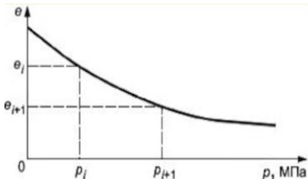
Рис. 2. Компрессионная кривая биогенного грунта
