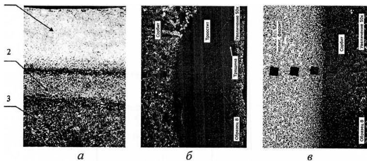
Рис. 2. Фотографии микроструктур покрытий из композиционного ферромагнитного порошка Fe-Ti: a – структурное строение покрытия после МЭУ; б – после МЭУ между зонами структурного строения ( \times 50 ); в – после МЭУ и лазерной обработки между зонами структурного строения ( \times 50 ); 1 – покрытие; 2 – зона термического влияния; 3 – основной материал
