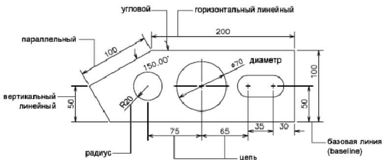
Рис. 7.18. Примеры размеров
