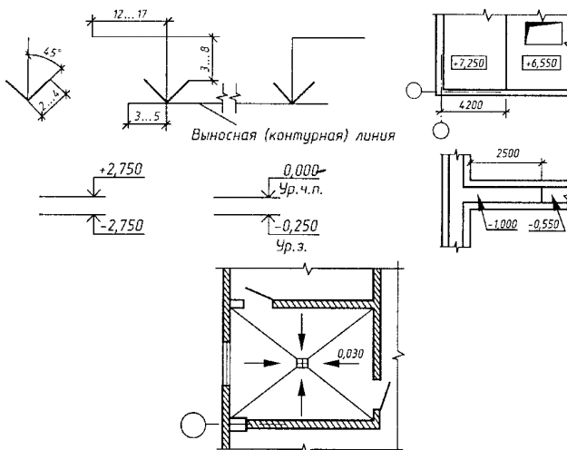
Рис. 6.10. Высотные отметки
