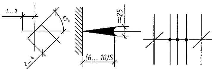
Рис. 6.6. Ограничение размерных линий засечкой, стрелкой
