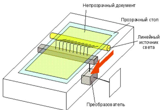
Рис. 7.79. Планшетный сканер
