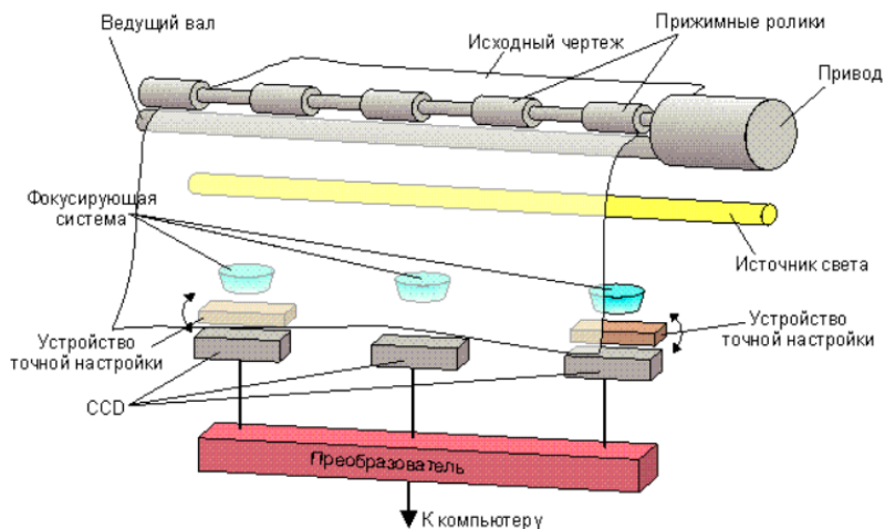
Рис. 7.77. Рулонный сканер
