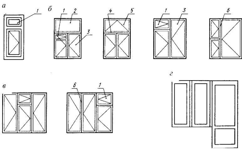
Рис. 5.3. Типы окон: а – одностворчатое; б – двухстворчатые; в – трехстворчатые ( 1 – форточка; 2 – глухая фрамуга; 3 – вертикальная створка переплета; 4 – средник; 5 – открывающаяся фрамуга; 6 – импост); г – с балконной дверью
