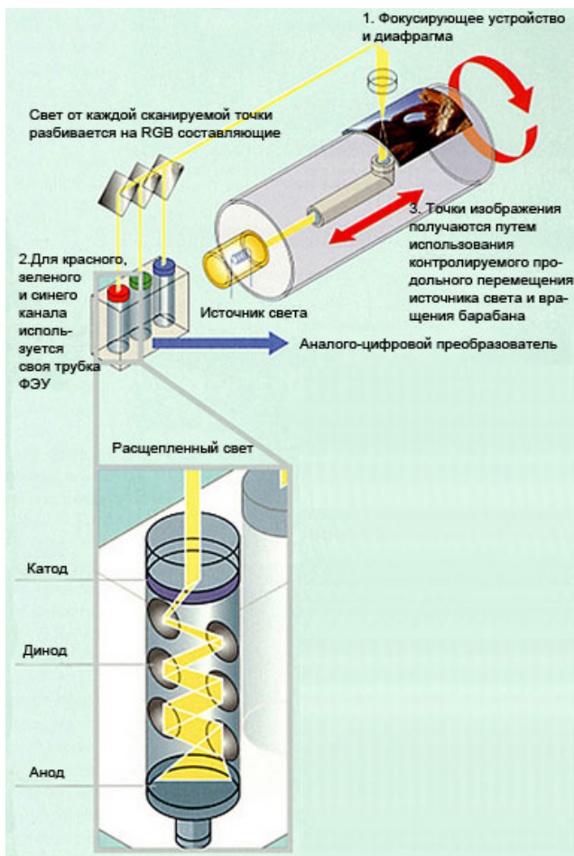
Рис. 7.81. Устройство барабанного сканера
