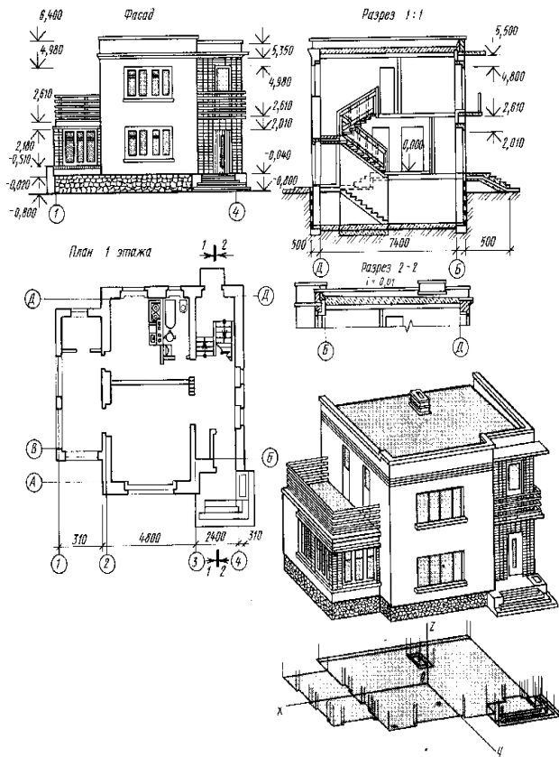
Рис. 6.1. Разрезы здания
