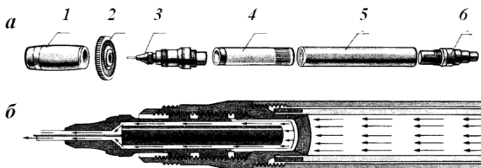
Рис. 1.2. Рапидограф:
