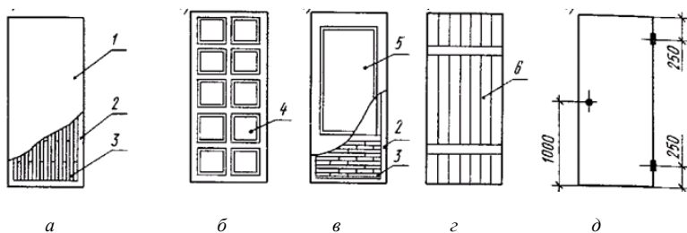
Рис. 5.5. Типы деревянных полотен:
