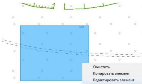
Рис. 7.29. Контекстовое меню
