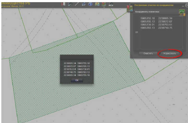
Рис. 7.65. Функция «Нарисовать»
