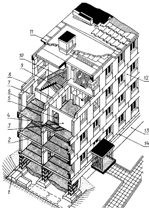
Рис. 6.2. Конструктивные элементы зданий:
