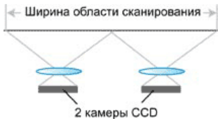
Рис. 7.76. Расположение CCD-камер
