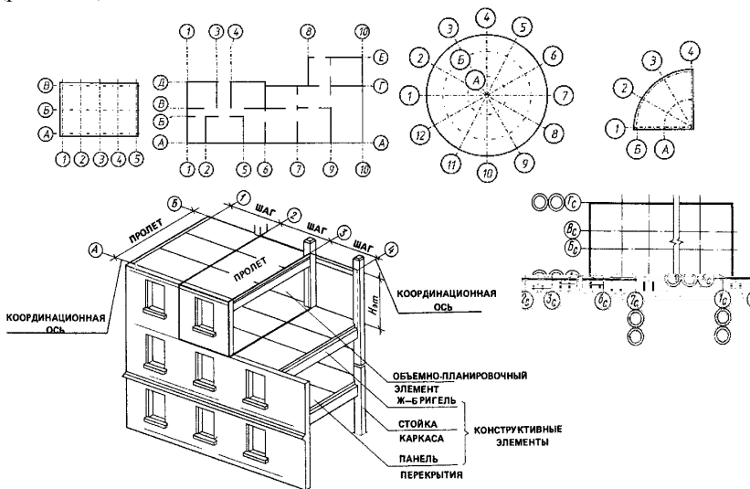
Рис. 6.19. Сетка координационных осей несущих конструкций здания
