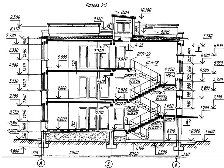
Рис. 6.12. Конструктивный разрез жилого дома по лестничной клетке
