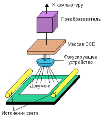
Рис. 7.80. Проекционный сканер
