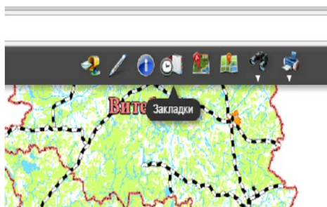
Рис. 7.62. Инструмент «Закладки»
