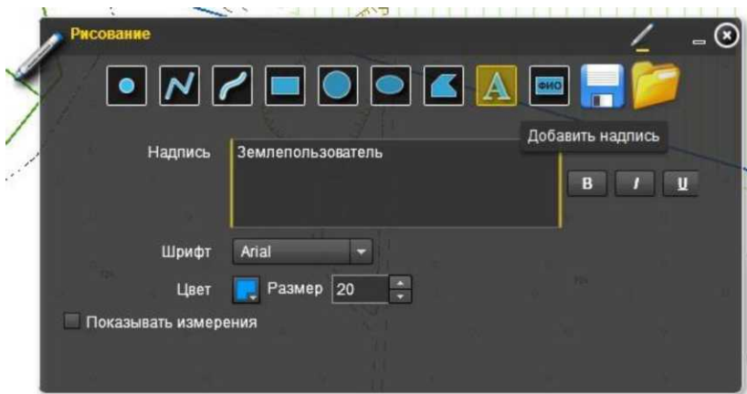
Рис. 7.33. Диалоговое окно
