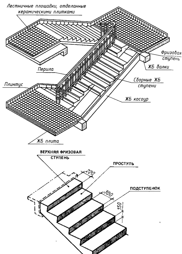
Рис. 5.7. Конструктивные элементы лестниц
