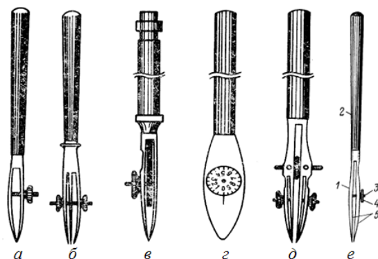
Рис. 1.3. Рейсфедеры:
