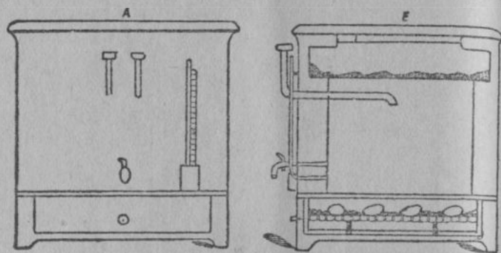
Рис. 90. Гидроинкубатор Ариу и Рулье. А — вид спереди. В — продольный разрез.
