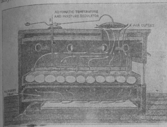
Рис. 97б. Одно из отделений инкубатора Ньютона-Гигант с отдельным регулятором теплоты.
