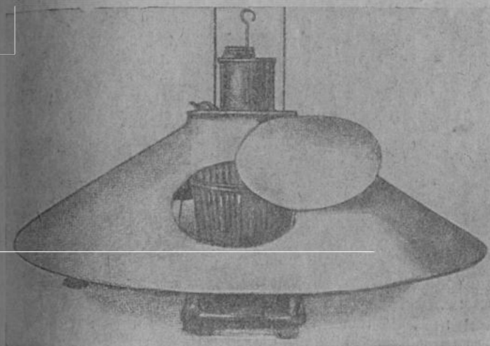
Рис. 107. Американский брудер с угольной печкой на 300 цыплят.
