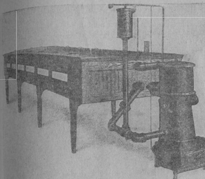
Рис. 95. Одиночный инкубатор Ньютон-Гигант на 1.800 яиц.
