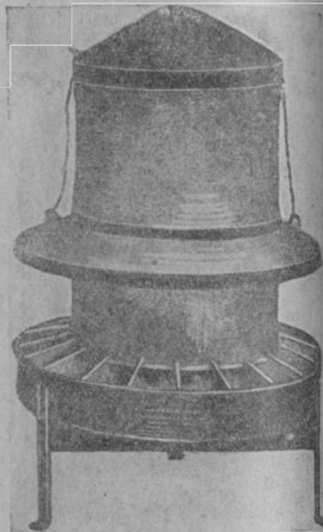
Рис. 131. Круглая автоматическая металлическая кормушка для зерна.
