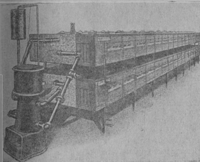
Рис. 96. Двойной инкубатор Ньютон-Гигант на 9.600 яиц.
