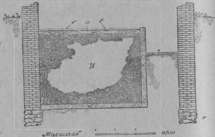
Рис. 195. Цистерна для хранения яиц в известковой воде в разрезе. Ц — цистерна, заполненная яйцами; б — бетонные пол и стенки; в — слой известковой воды поверх яиц; л — ледок; п — пол прохода вдоль цистерн.
