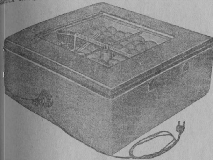
Рис. 91. Электрический инкубатор.
