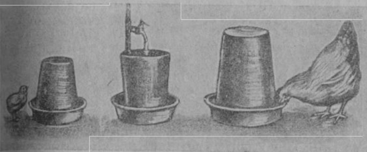
Рис. 133. Сифонные цинковые или оцинкованные поилки.
