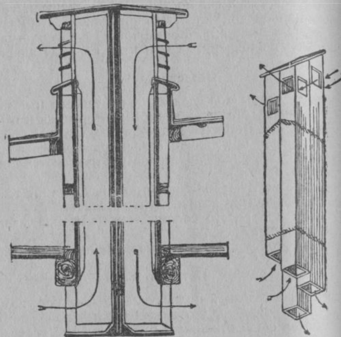
Рис. 150. Вытяжная труба по Муиру.
