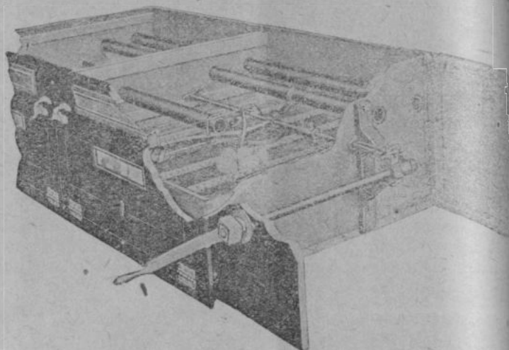
Рис. 102. Система рычагов для переворачивания яиц в инкубаторах Джемсвей.
