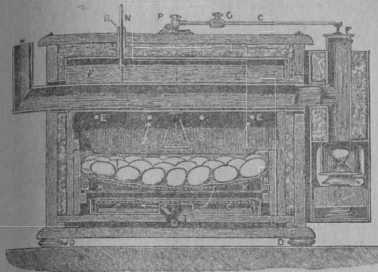
Рис. 88. Инкубатор Хирсона в разрезе.
