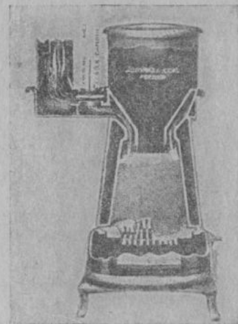
Рис. 97а. Печь при инкубаторе Ньютона-Гиганта с автоматической подачей угля.
