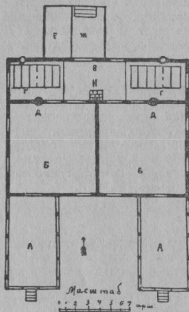
Рис. 151. План большого двойного зимнего курятника О. М. Орловой. А—стеклянный балкон. Б—выгульная. В—спальня. Г—нашесты. Д—печь. Е—прихожая. Ж—крытый навес и ход наверх. З—кладовая. И—кирпичная основа для печки. К—вентилятор.
