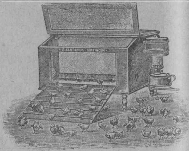
Рис. 105. Искусственная матка Сарториуса.
