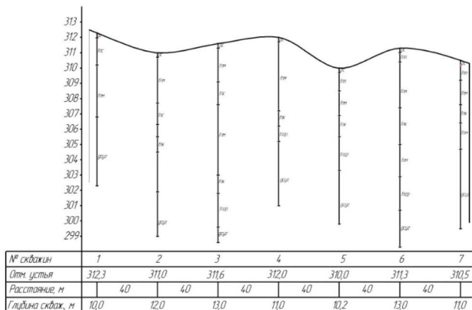
Рис. 6.5. Результаты распределения грунтов по скважинам
