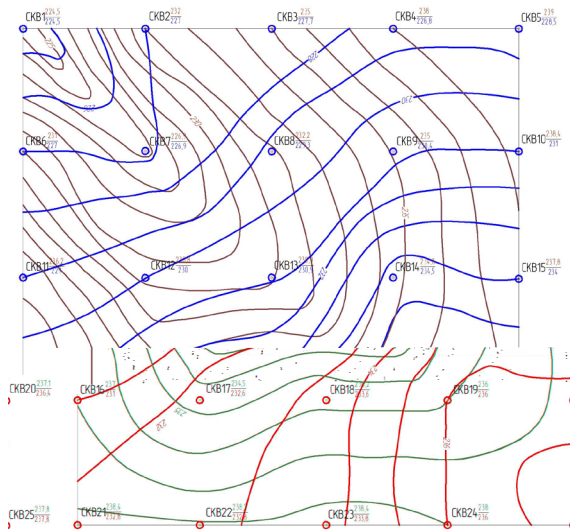
Рис. 5.5. Карта гидроизогипс, совмещенная с горизонталями
