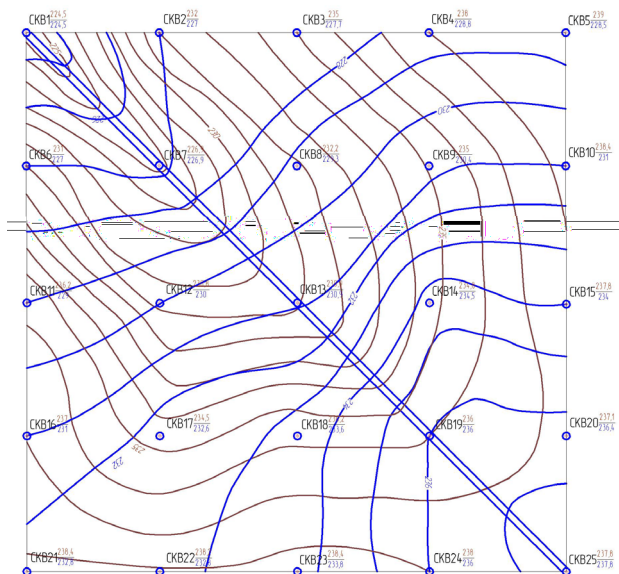
Рис. 5.6. Русло канала
