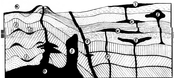
Рис. 2.1. Формы залегания магматических горных пород: а – батолит; б – шток; в – лополит; з – лакколлит; д – факолит; е – магматические жилы (дайки); ж – силлы; з – покров; и – вулканический конус; к – лавовый поток
