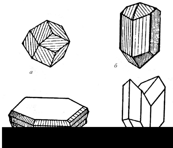
Рис. 1.4. Формы кристаллов минералов: а – изометрическая (магнетит); б – вытянутая в одном направлении (антимонит); в – вытянутая в двух направлениях (хлорит); г – двойник кристаллов гипса
