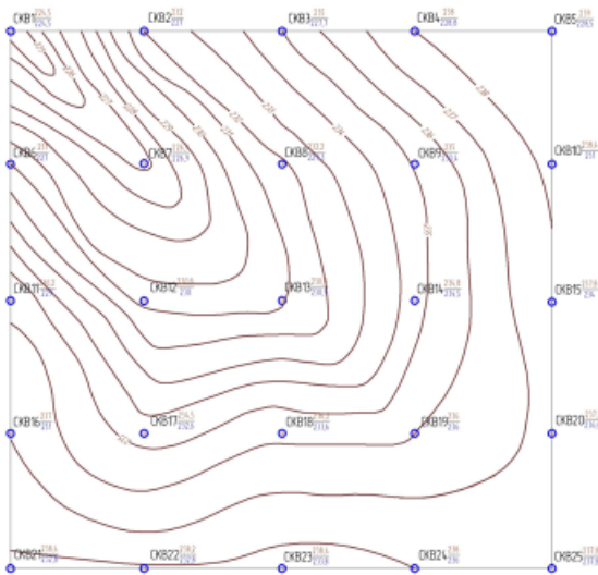
Рис. 5.4. Карта горизонталей
