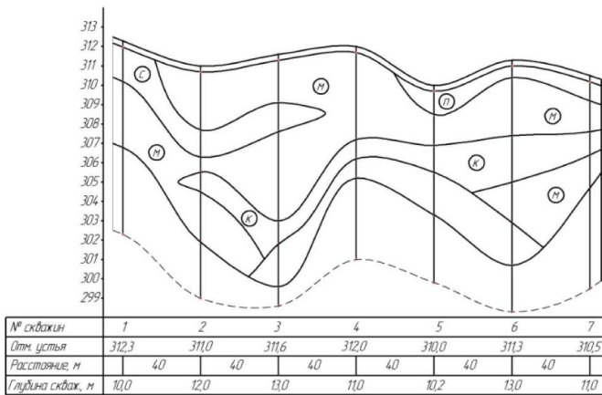
Рис. 6.6. Геолого-литологический разрез
