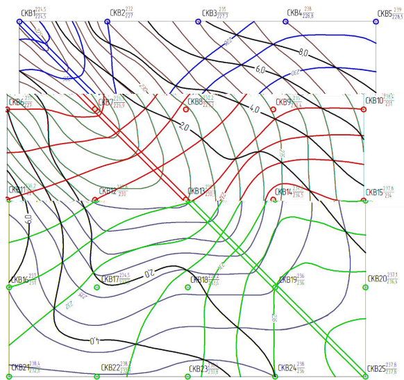
Рис. 5.7. Линии тока воды (гидроизобаты)
