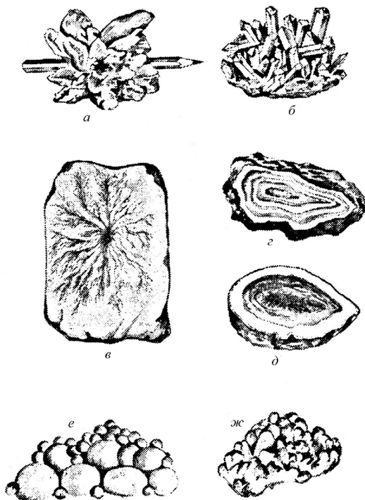
Рис. 1.5. Формы нахождения минералов в природе: а, б – друзы кристаллов гипса и кварца; в – дендрит марганцевых соединений на известняке; г – секреция; д – жеода; е – шаровидные конкреции; ж – почковидные натечные формы
