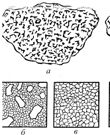
Рис. 2.2. Структура интрузивных пород: а – пегматитовая; б – полнокристаллическая, неравномерно-зернистая (порфировидная); в – полнокристаллическая, равномерно-зернистая
