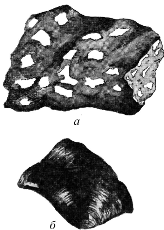
Рис. 2.3. Структура эффузивных пород: а – неполнокристаллическая (порфировая); б – некристаллическая (стекловатая)
