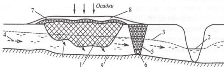
Рис. 8.1. Схема эколого-экономической безопасности на свалках: 1 – локальный объект-загрязнитель; 2 – водный объект; 3 – УГВ; 4 – фильтрационный поток; 5 – дренажно-аккумулирующая система; 6 – дрена; 7 – защитный слой мелиоранта-сорбента; 8 – плодородный слой; 9 – водоупор
