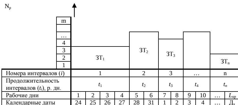
Рис. 18. Форма графика поставки трудовых ресурсов на объект строительства
