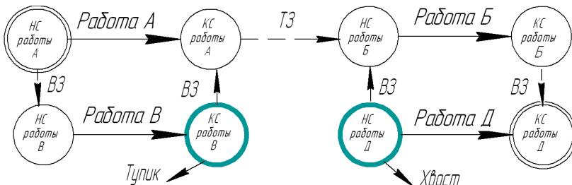
Рис. 10. Правило недопустимости «тупиков» и «хвостов»
