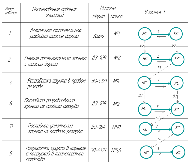
Рис. 13. Фрагмент табл. 14 по вертикальной увязке «полузависимых» работ на участке 1 проектной трассы дороги (вариант задания № 11)
