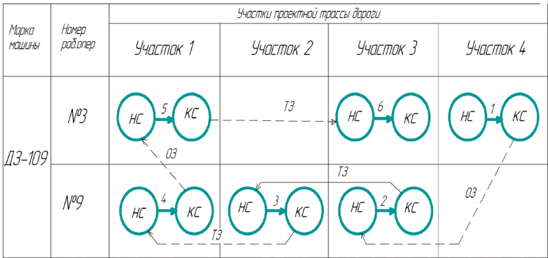
Рис. 12. Фрагмент табл. 14 по горизонтальной увязке «зависимых» работ для бульдозера Б-10МБ № 3 (вариант задания № 11)
