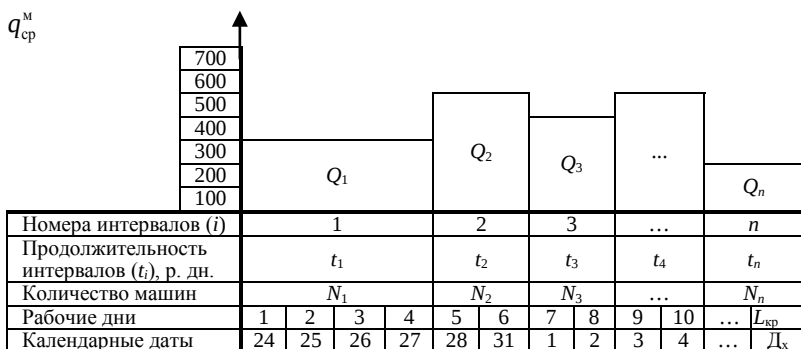
Рис. 20. Форма графика поставки ТСМ на объект строительства
