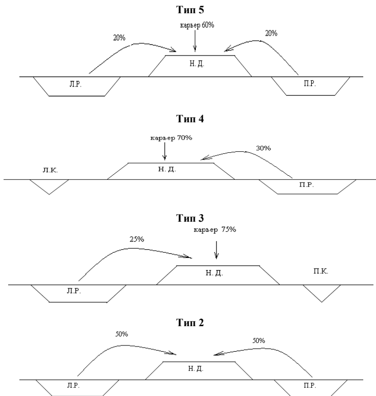
Рис. 2. Типы поперечных сечений насыпи земполотна автодороги
