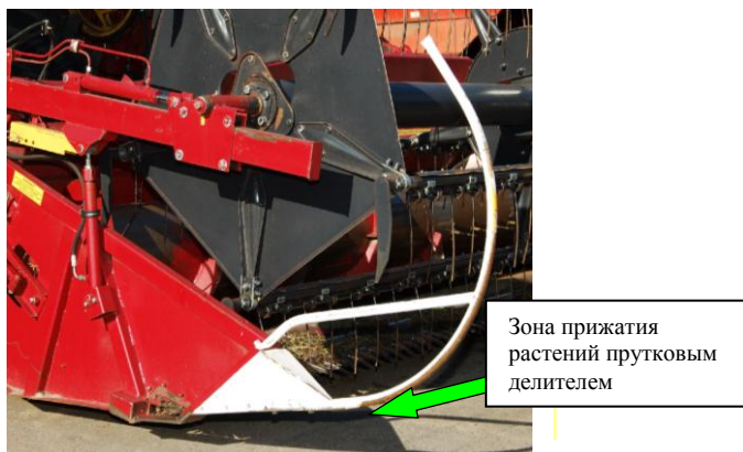
Рис. 4.4. Конструкция делителя комбайнов «ПАЛЕССЕ GS»
