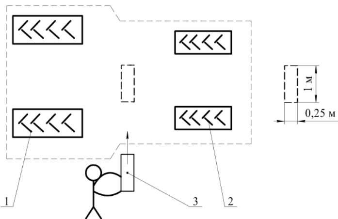
Рис. 7.7. Схема расположения лотка при определении потерь зерна: 1 – передние колеса; 2 – задние колеса; 3 – лоток (1,0×0,25 м)
