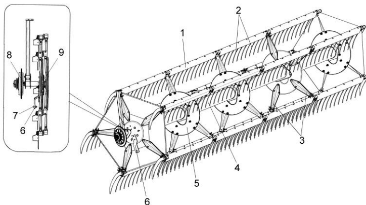
Рис. 4.3. Мотовило:
