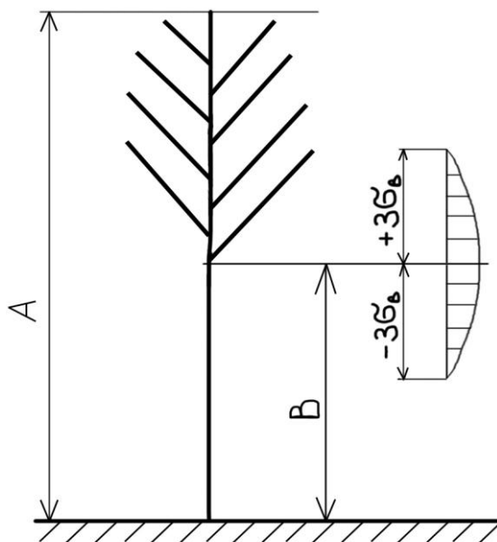
Рис. 3.2. Схема растения крестоцветных культур с характерными параметрами
