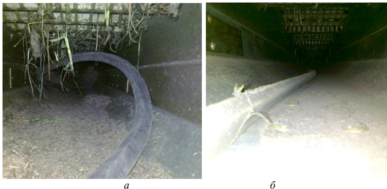
Рис. 6.3. Устранение забиваний клавиш посредством установки дополнительного ремня внутри клавиш: а – ремень установлен в забитую клавишу; б – очищенная клавиша при использовании ремня
