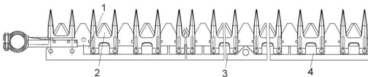
Рис. 4.9. Режущий аппарат: 1, 3, 4 – пластины трения; 2 – сегмент
