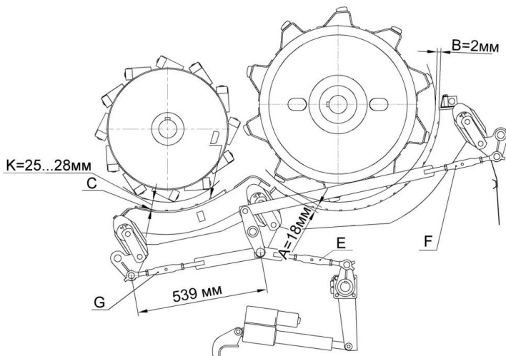
Рис. 5.2. Зазоры и установочная длина регулируемых тяг в механизмах молотильного аппарата
