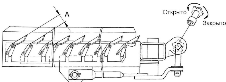
Рис. 6.5. Регулировка открытия жалюзи решет: А – положение жалюзи решет
