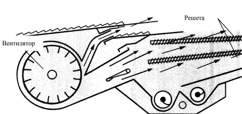
Рис. 6.2. Общее устройство очистки комбайна
