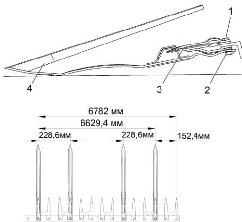
Рис. 4.10. Установка стеблеподъемника: 1 – болт крепления стеблеподъемника; 2 – гайка крепления стеблеподъемника; 3 – палец режущего аппарата; 4 – стеблеподъемник
