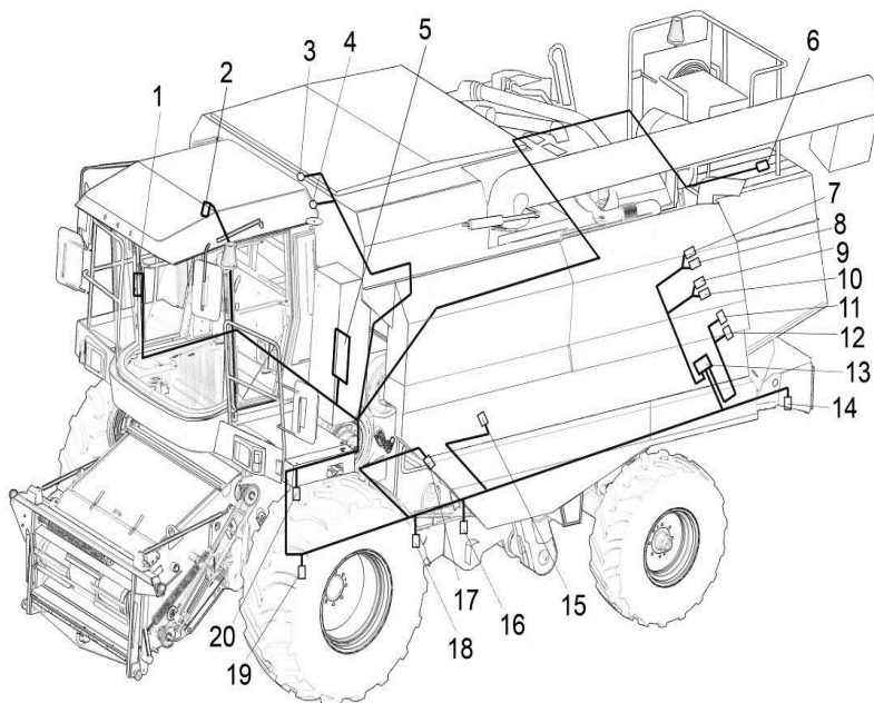
Рис. 7.2. Автоматическая система контроля комбайна (АСК):
