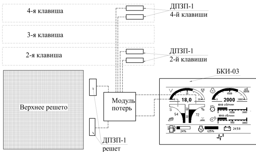
Рис. 7.5. Схема работы устройства для определения потерь зерна
