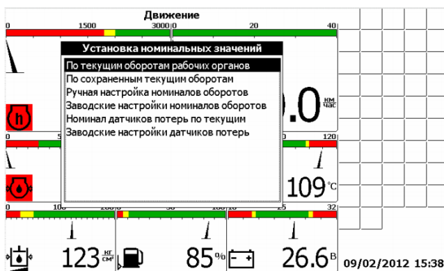
Рис. 7.10. Индикация меню «Установка номинальных значений»
