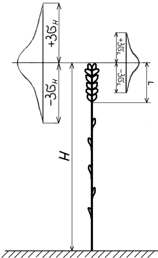
Рис. 3.1. Схема растения зерновой культуры с характерными параметрами высоты H и длины колоса L с учетом изменчивости параметров по средним квадратическим отклонениям \sigma
