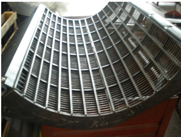
Рис. 5.4. Экспериментальное подбарабанье с дифференцированной рабочей поверхностью
