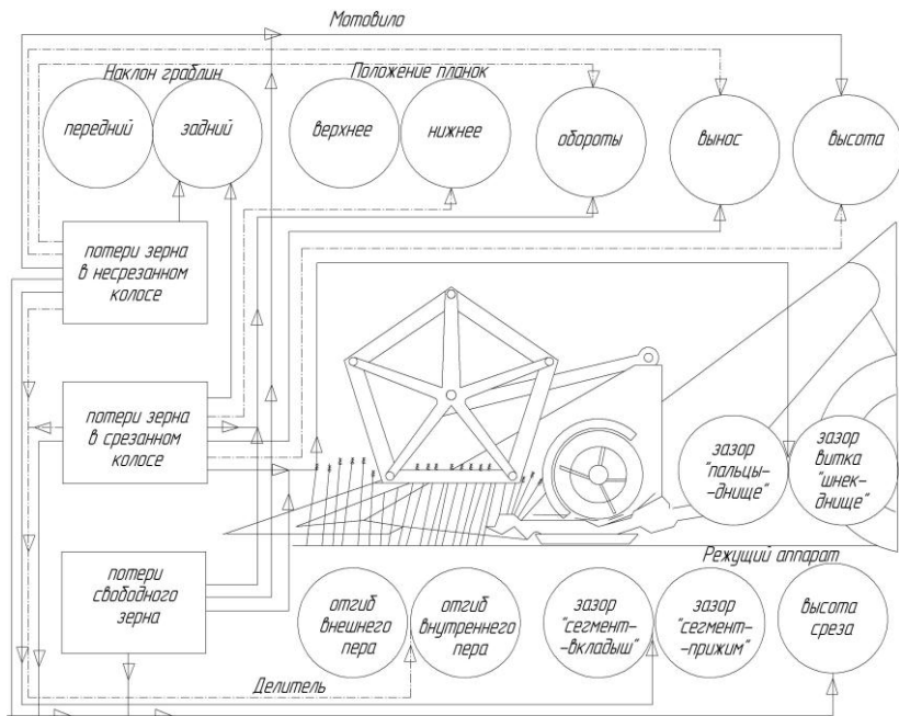
Рис. 4.1. Причины потерь зерна за жаткой и способы их устранения
