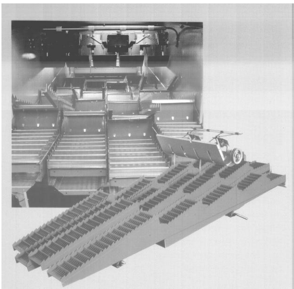
Рис. 6.1. Устройство клавишного соломотряса с активатором
