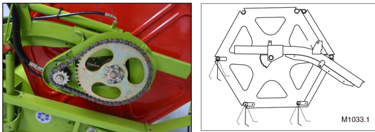
Рис. 4.13. Механизм установки мотовила на изогнутых направляющих
