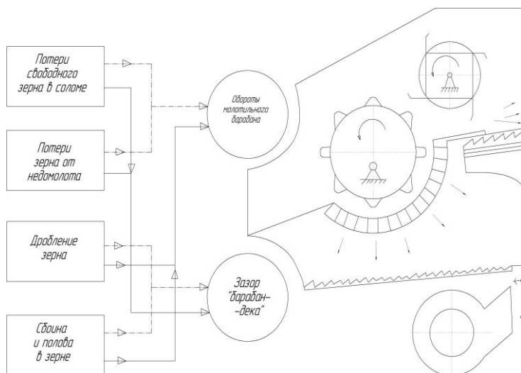
Рис. 5.1. Недостатки в работе молотильного аппарата и их причины
