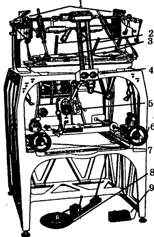
Рис. 3. Стереопроектор СПР-2.
