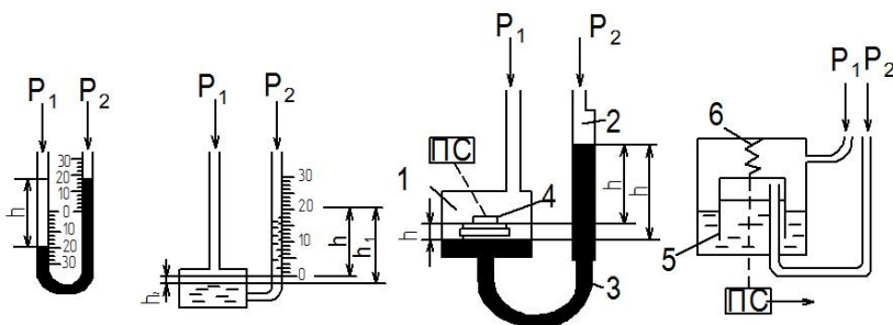
Рис. 1.10. Жидкостные манометры: а – U-образный (двухтрубный); б – чашечный (однотрубный); в – поплавковый; г – колокольный
