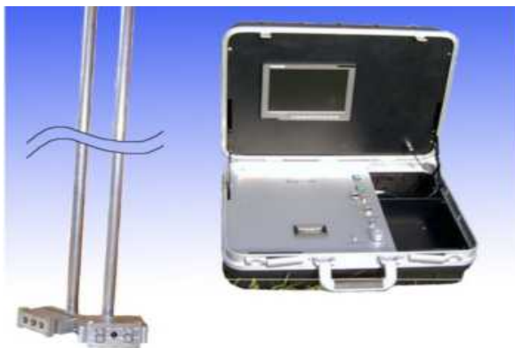
Рис. 8.5. Модификация комплекта средств диагностики КСД-160У
