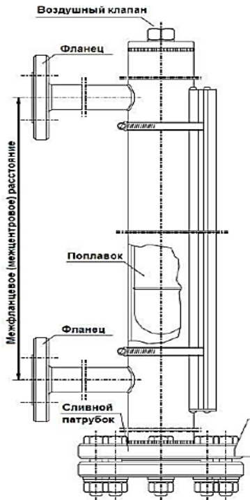
Рис. 1.28. Устройство байпасного поплавкового магнитного уровнемера
