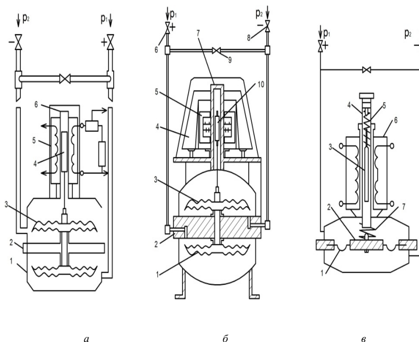
Рис. 1.14. Конструкция дифманометров мембранных: а – тип ДМ; 1, 3 – мембранные коробки; 2 – основание; 4 – сердечник; 5 – дифференциально-трансформаторный преобразователь; 6 – немагнитная разделительная трубка; б – тип ДМЭ (или ДМЭР): 1, 3 – мембранные коробки; 2 – основание; 4 – полупроводниковый усилитель; 5 – передающий преобразователь с магнитной компенсацией; 6, 8 – запорные вентили; 9 – регулирующий вентиль; 10 – магнитный плунжер; в – тип ДМИ: 1 – вялая (неметаллическая) мембрана; 2 – жесткий центр; 3 – сердечник; 4 – разделительная трубка; 5 – винтовая цилиндрическая пружина; 6 – дифференциально-трансформаторный преобразователь; 7 – дополнительная пружина
