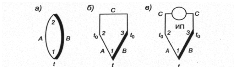
Рис. 1.24. Термоэлектрические цепи термоэлектрических термометров:
