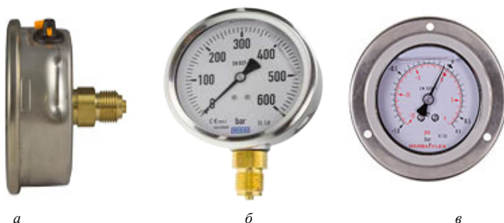
Рис. 1.12. Манометры: а – с осевым (тыловым) подключением; б – с радиальным подключением; в – с креплением переднего кольца
