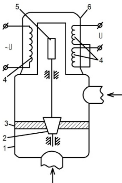
Рис. 1.17. Ротаметр с дифференциально-трансформаторным преобразователем:
