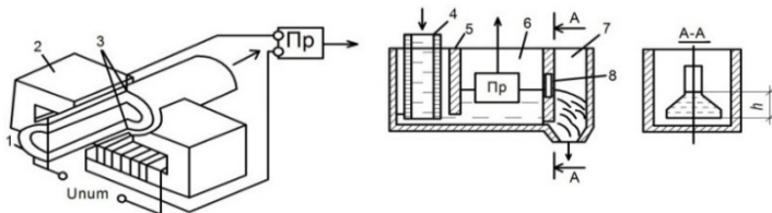
Рис. 1.16. Расходомеры жидкостей и пульп: а – электромагнитный; б – переменного уровня (щелевой)
