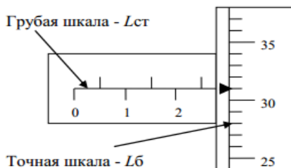
Рис. 1.9. Шкалы микрометра
