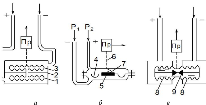
Рис. 1.13. Дифференциальные манометры с упругими чувствительными элементами (деформационные): а – мембранный; б – с вялой мембраной; в – сильфонный
