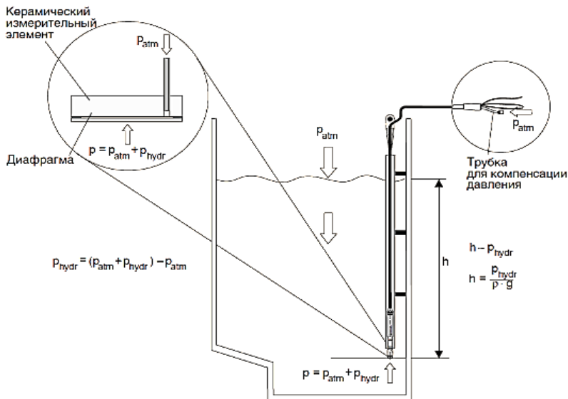
Рис. 1.27. Принцип работы гидростатического уровнемера
