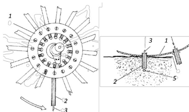
Рис. 3. Схема высева семян рабочими органами машины Spapperi SMP: 1 – высевающее колесо; 2 – высевающие трубки; 3 – очищающие спицы; 4 – кулачок; 5 – семена
