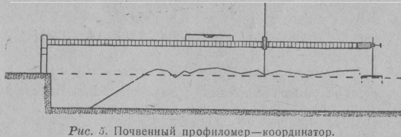
Рис. 5. Почвенный профиломер—координатор.
