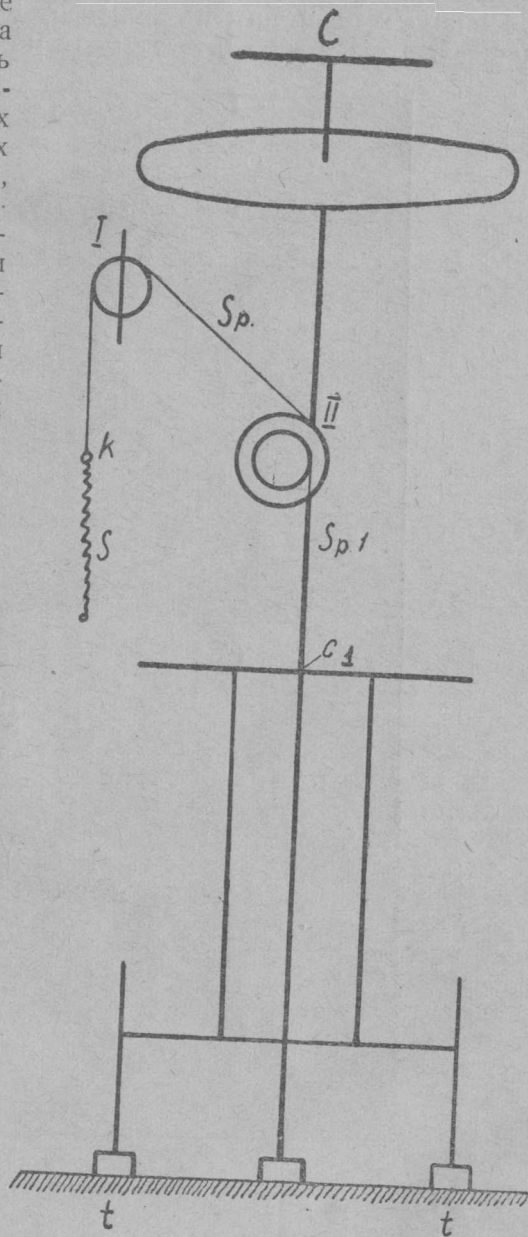
Рис. 7. Схема передач.
