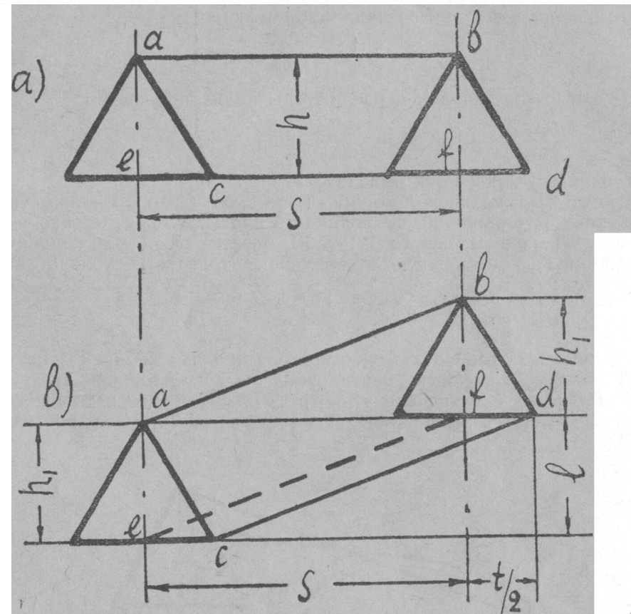
Фиг. 3. Площади, перекрываемые лезвием фиктивного и реального клинка.
