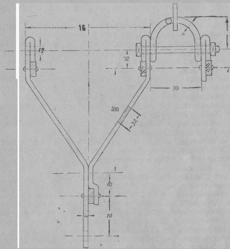
Фиг. 6. Звено бороны Вермке WE.
