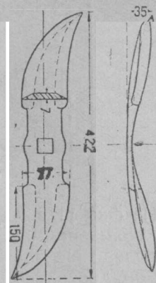
Фиг. 12. Нож культиватора „Ганкмо“.
