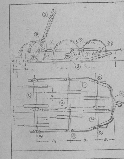
Рис. 1. Две проекции конного пружинного культиватора
