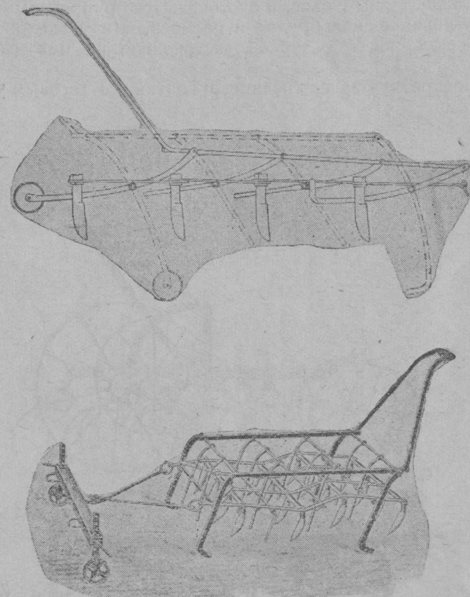
Фиг. 7. Культиватор „Аурас“
