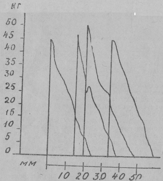
Рис. 9. Диаграмма Bodendruckdynamometer'a
