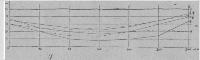
Рис. 11. Траектории концов зубьев при изменении нагрузки; к табл. № 1.
