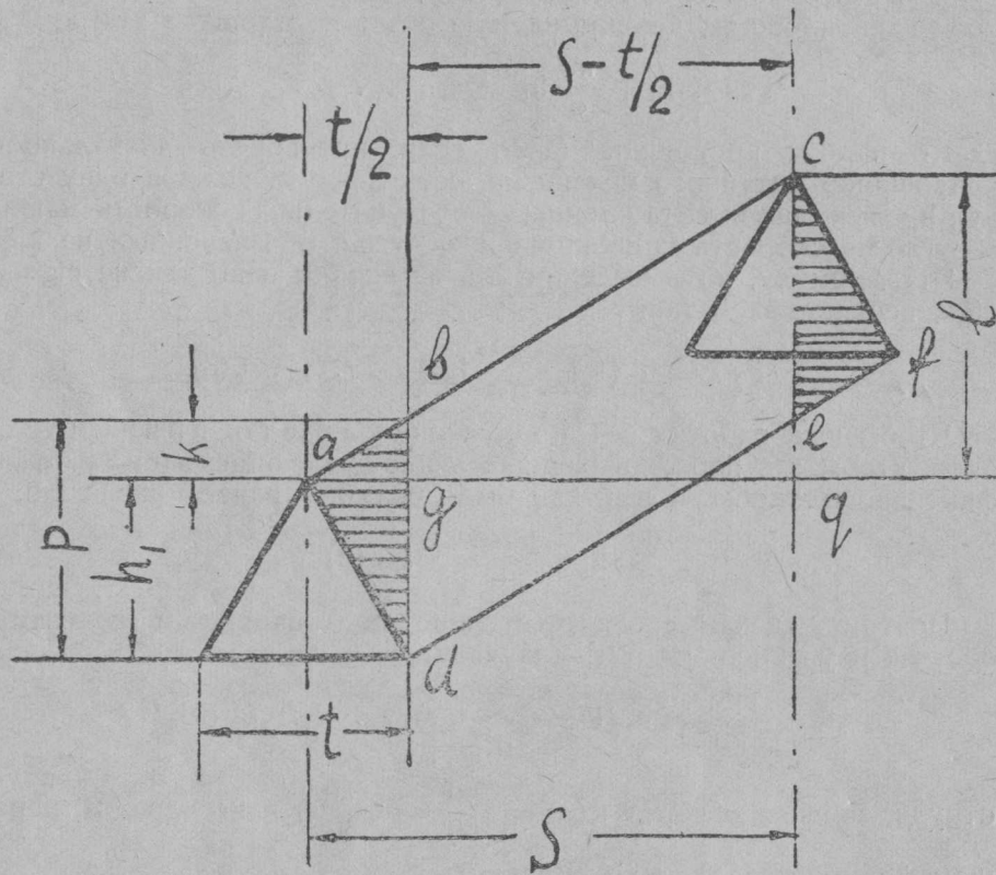
Фиг. 5. Определение площади перекрытия лезвием.
