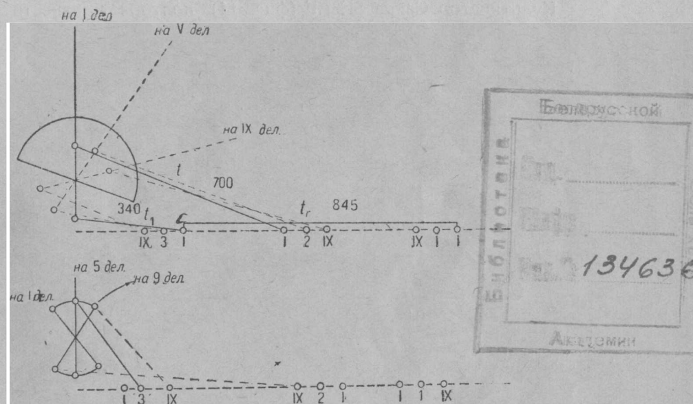
Фиг. 13. Схема рычажного механизма культиватора „Ганкмо“
