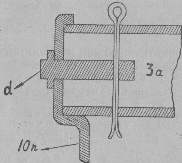
Рис. 2. Крепление подшинника поперечного бруска
