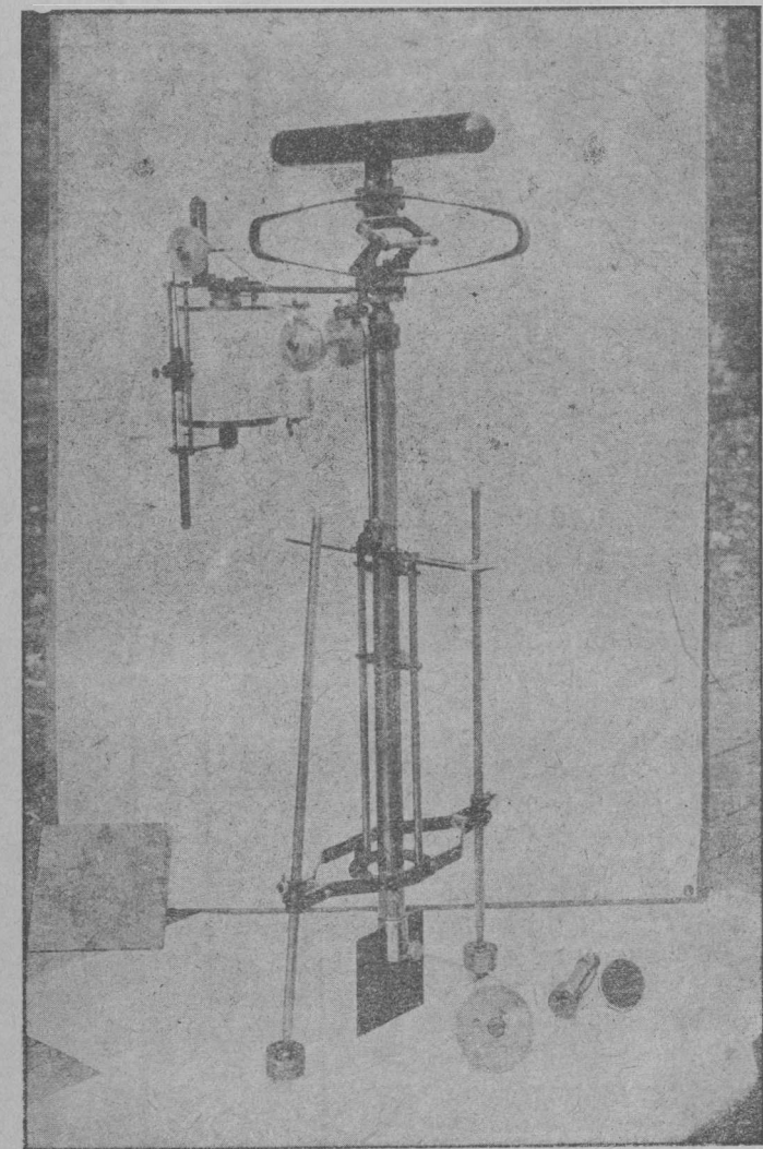
Рис. 6. Bodendruckdynamometer.
