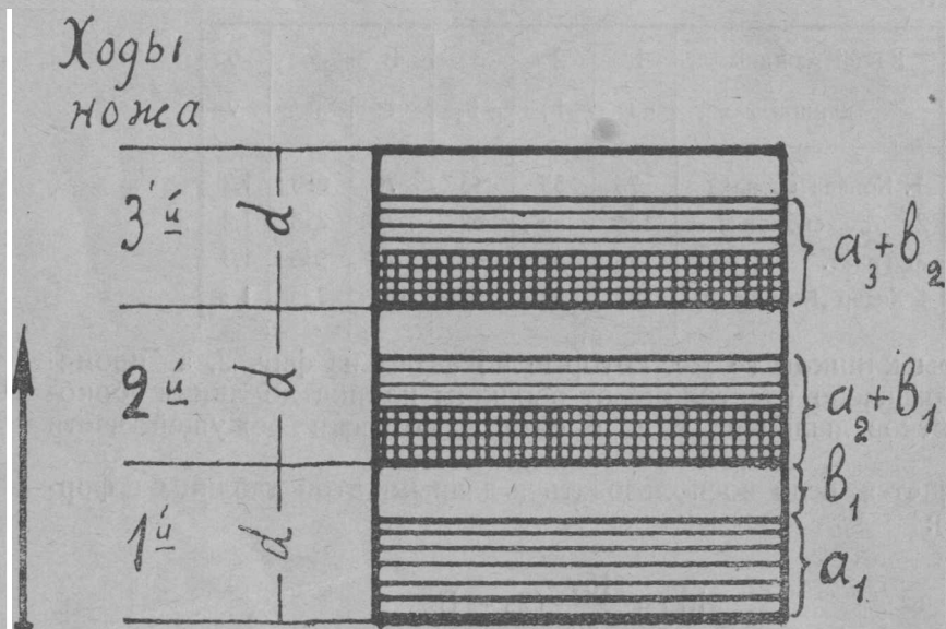
Фиг. 7. Перемещение стеблей с одной полосы резания в другую.
