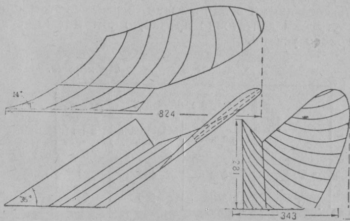
Фиг. 17. Рабочая поверхность корпуса плуга П7П12 в трех проекциях.
