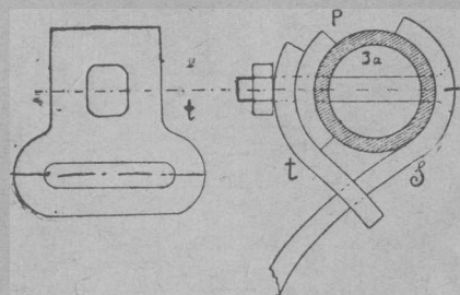
Рис. 3. Укрепление зубьев
