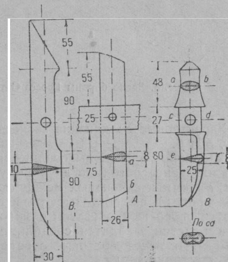
Фиг. 4. Зубья луговых борон.
