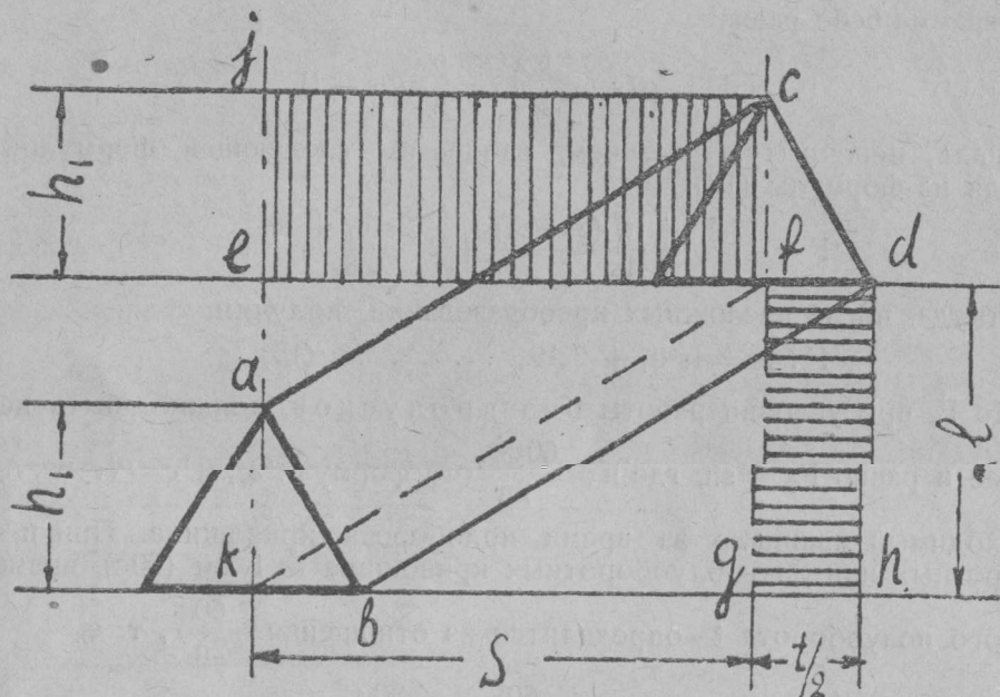
Фиг. 6. Определение площади перекрытия лезвием с разложением ее на две площади.
