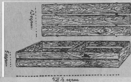
Рис. 6. Ящик для упаковки яиц.
