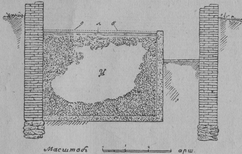
Рис. 4. Цистерна для хранения яиц в известковой воде в разрезе. Ц—цистерна, заполненная яйцами; б—бетонные пол и стенки; б—бетонная стенка соседней цистерны; в—слой известковой воды поверх яиц; л—ледок; п—пол прохода вдоль цистерн.
