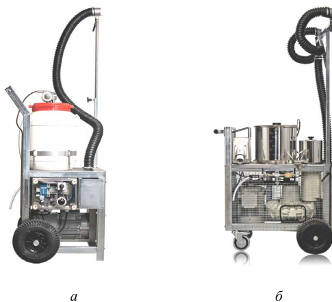
Рис. 7. Аэрозольные генераторы ультрамалого объема: а – ИГЕБА U 5 E; б – ИГЕБА U 15 E
