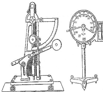
Рис. 30. Динамометр ДШМ-3М ( ) для определения крепости шерсти и торсионные весы ( )
