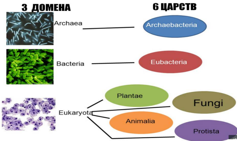
Рис. 1.3. Соотношение таксономических рангов: доменов и царств
