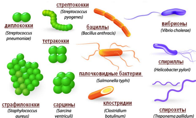
Рис. 1.30. Основные морфологические группы бактерий
