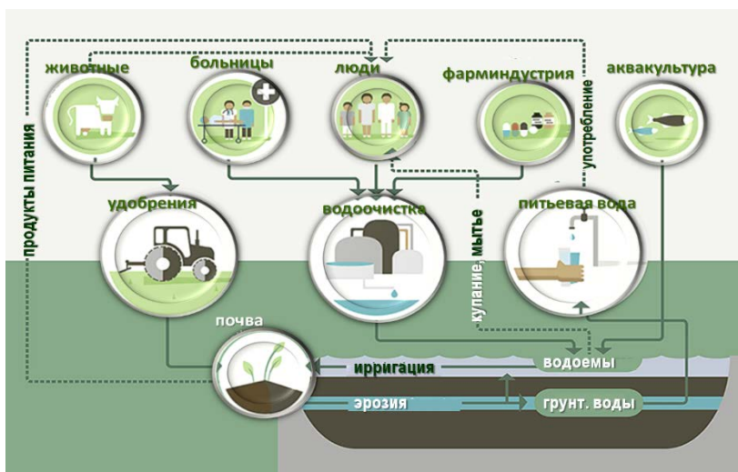
Рис. 1.63. Круговорот воды и пути распространения микроорганизмов в природе
