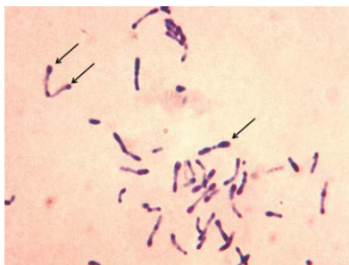
Рис. 1.23. Морфология Corynebacterium diphtheriae
