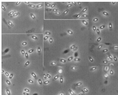
Рис. 1.41. Споры Bacillus anthracis
