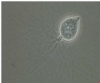
Рис. 1.5. Хитридомицет Obelidium micronatum в процессе дифференцировки в спорангий, из которого высвободятся зооспоры
