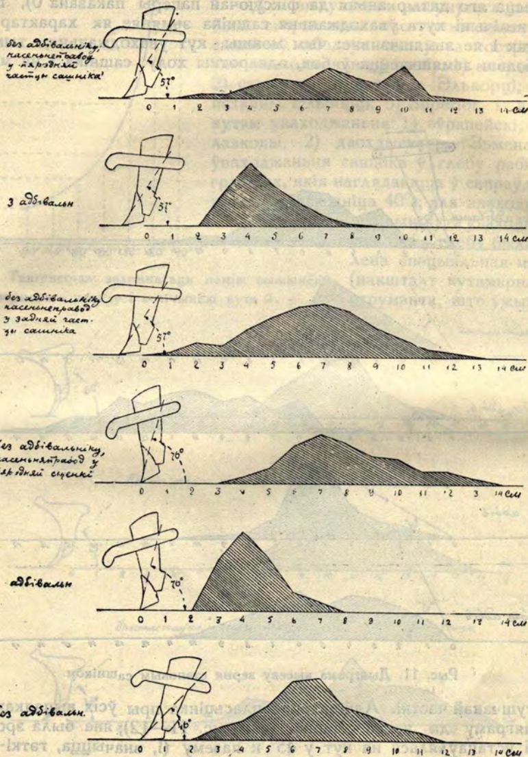
Рис. 12. Дьяграма высева зерня пятачным сашніком.
