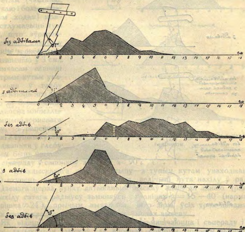
Рис. 11. Дыяграма высеу зерня стэповым сашніком.
