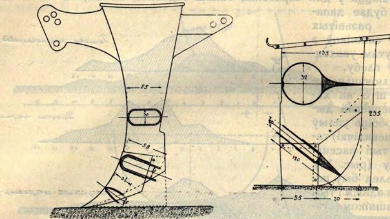
Рис. 16. Сашнікі з гострым і тупым кутам уваходжання ў глебу.
