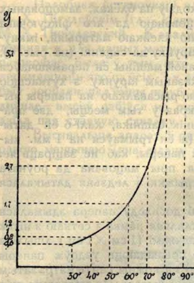
Рис. 9. Тангенсоїда: залежність паміж вишиною зерневого каналу і величиною кута \alpha .
