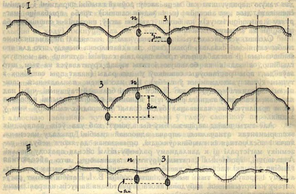
Рыс. 1. Стан зерневых каналаў і профілі поля пры розных нагрузках на сашнік; n—зерневый канал пярэдняга сашніка, 3—задняга.
