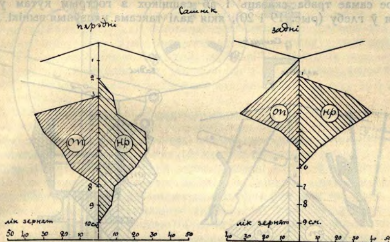
Рис. 18. Дыяграма высеву зерня ў глебу сашніком а тупым кутам уваходжання ў глебу.
