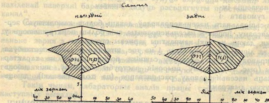
Рис. 17. Дыяграма высеву зерна ў глебу сашніком з тупым кутам уваходжання ў глебу.
