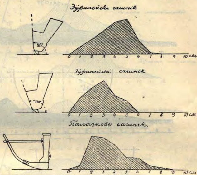
Рис. 13. Дыяграма высеву зерня эўрапейскім і палазковым сашніком.
