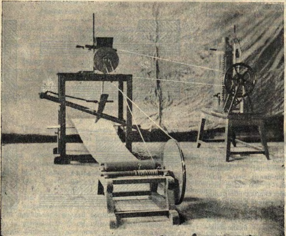
Рыс. 6. Устаноўка для высева зерня на рухавую роўніцу.
