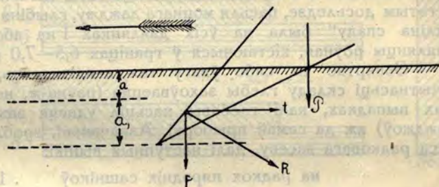
Рис. 4. Уплыў сіл на сашнік.
