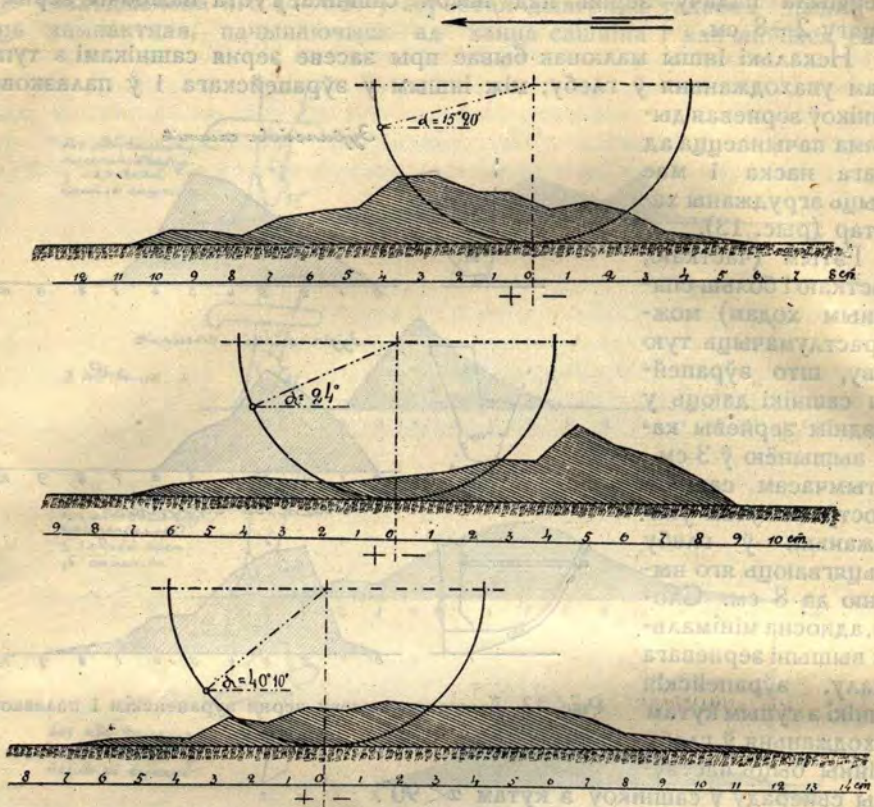
Рис. 14. Дыяграма высеву зерня двохдыскавым сашніком (диск не ў маштабе).
