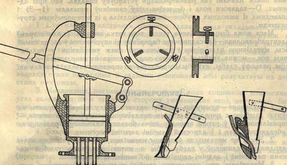
Рис. 21. Деталі приладу для азначення глєбіні ходу сашніка.
