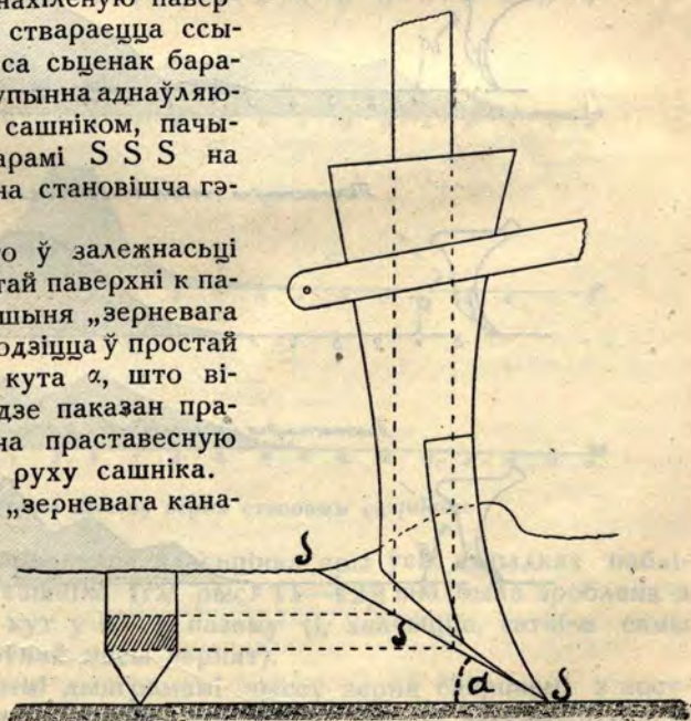
Рис. 8. Спад зернят на нахіленую паверхню глебы.
