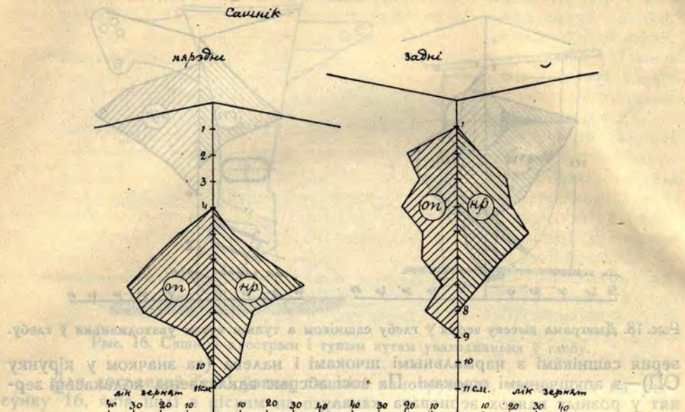
Рис. 20. Дыяграма высеву зерня ў глебу сашніком з гострым кутам уваходжання ў глебу.
