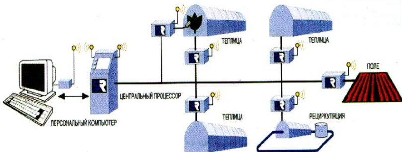
Рис. 3.2. Схема станции фитомониторинга
