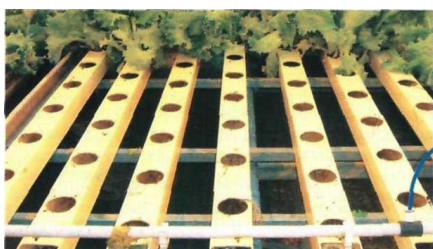
Рис. 9.1. Культивационные каналы с распределительной гребенкой для подачи питательного раствора
