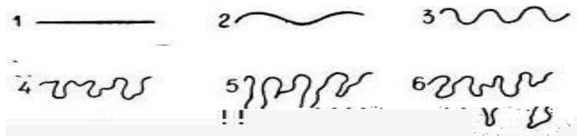
Рис. 5.5. Формы границ между генетическими горизонтами в профиле почв 1 – ровная; 2 – волнистая; 3 – карманная; 4 – языковатая; 5 – затечная; 6 – размытая
