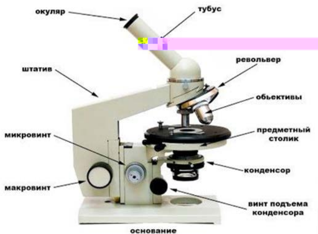
Рис. 1.2. Устройство микроскопа
