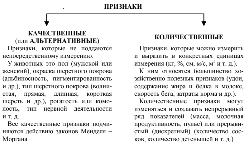
Рис. 1. Классификация признаков
