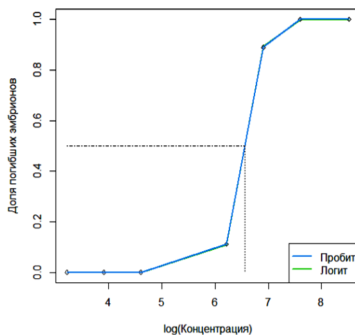
Рис. 4. Пробит-логит (log) зависимости для выживаемости эмбрионов радужной форели под влиянием «кукурузной» фульвовой кислоты
