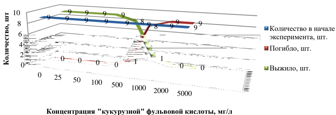
Рис. 3. Выживаемость эмбрионов и личинок радужной форели под влиянием «кукурузной» фульвовой кислоты
