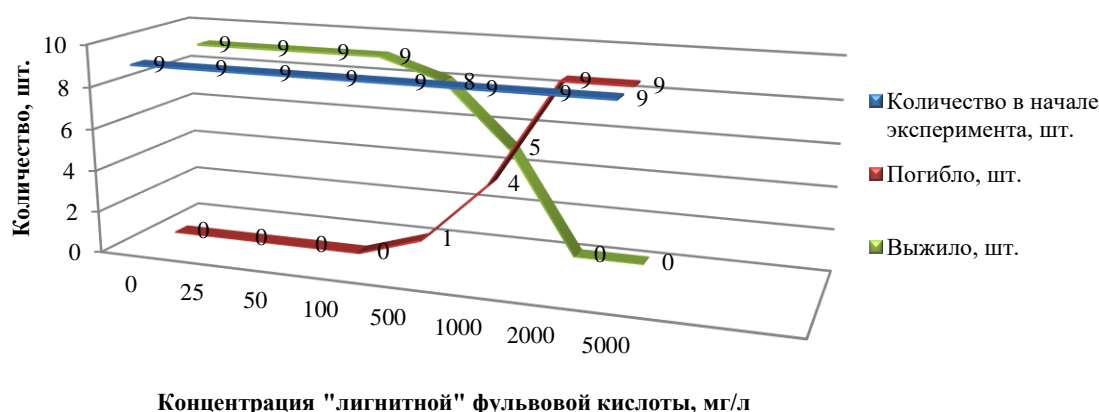
Рис. 1. Выживаемость эмбрионов и личинок радужной форели под влиянием «лигнитной» фульвовой кислоты
