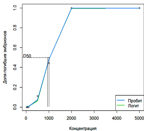
Рис. 2. Пробит-логит зависимости для выживаемости эмбрионов радужной форели под влиянием «лигнитной» фульвовой кислоты
