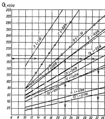
Рис. 4. Диаграмма зависимости нормы высева семян от длины рабочей части катушки при различных передаточных отношениях сеялки СЗ-3,6А: П – пшеница; Р – рожь; О – овес; Гр – гречиха; Л – лен
