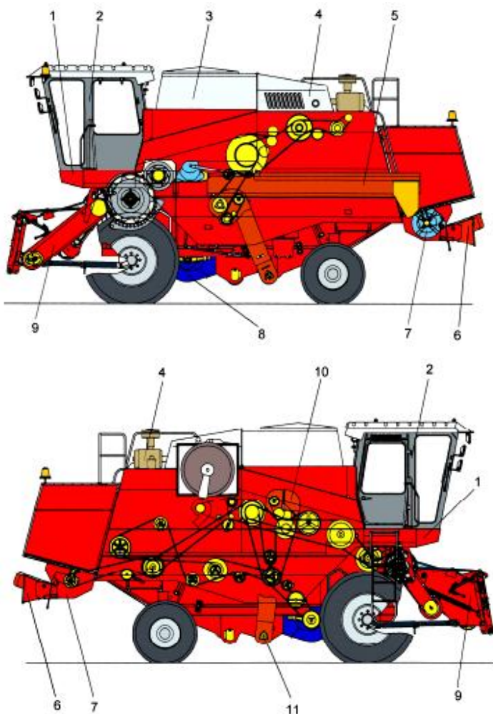
Рис. 14. Самоходный зерноуборочный комбайн КЗС-10 ПАЛЕССЕ GS10: 1 – площадка управления; 2 – кабина; 3 – бункер зерновой; 4 – моторная установка; 5 – шнек поворотный выгрузной; 6 – дефлектор; 7 – соломоизмельчитель; 8 – очистка; 9 – камера наклонная; 10 – шнек загрузной зерновой; 11 – элеватор зерновой
