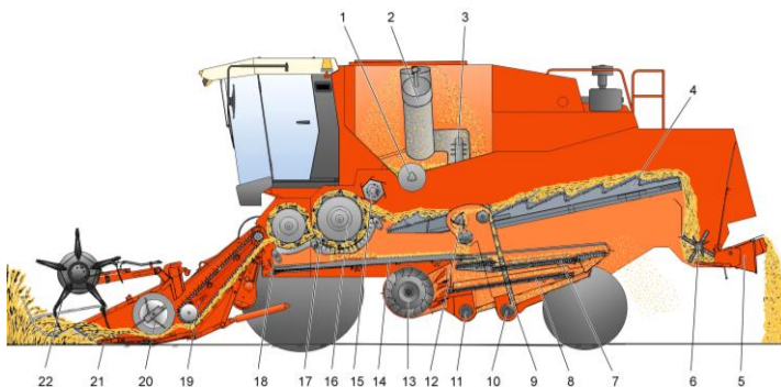
Рис. 11. Схема технологического процесса работы комбайна ПАЛЕССЕ GS12: 1 – шнек горизонтальный; 2 – шнек загрузной зерновой; 3 – элеватор зерновой; 4 – соломотряс; 5 – дефлектор; 6 – соломоизмельчитель; 7 – верхний решетный стан; 8 – нижний решетный стан; 9 – элеватор колосовой; 10 – шнек колосовой; 11 – шнек зерновой; 12 – домолачивающее устройство; 13 – вентилятор; 14 – стрясная доска; 15 – отбойный битер; 16 – барабан молотильный; 17 – подбарабанье; 18 – барабан-ускоритель; 19 – транспортер наклонной камеры; 20 – шнек; 21 – режущий аппарат; 22 – мотовило
