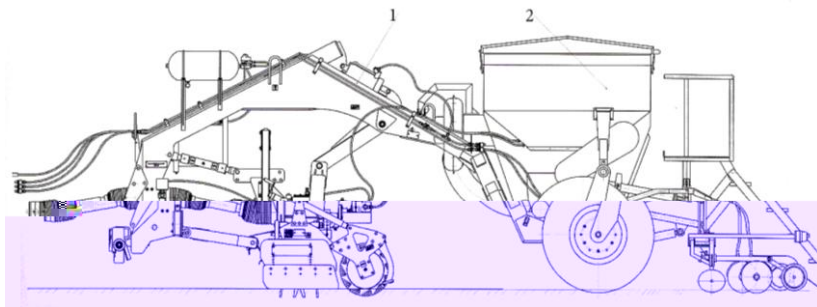
Рис. 6. Общий вид агрегата почвообрабатывающе-посевного АППА-4 с активными рабочими органами: 1 – адаптер почвообрабатывающий; 2 – сеялка
