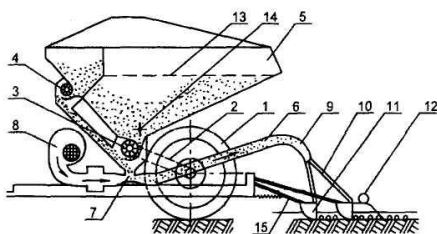
Рис. 3. Технологическая схема пневматической универсальной сеялки С-6: 1 – опорно-приводное колесо; 2 – цепная передача; 3, 4 – высевающие аппараты; 5 – бункер; 6, 10 – семявоздухопроводы; 7 – эжектор; 8 – вентилятор; 9 – распределитель; 11 – сошник; 12 – пружинный загортач; 13 – сетка; 14 – ворошилка
