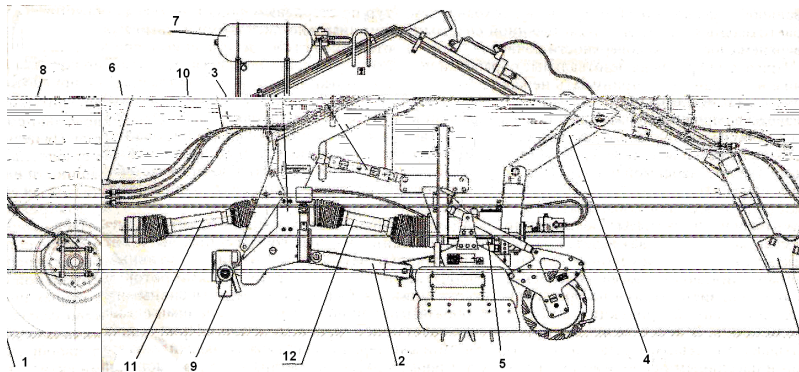
Рис. 7. Адаптер почвообрабатывающий (вид сбоку):
