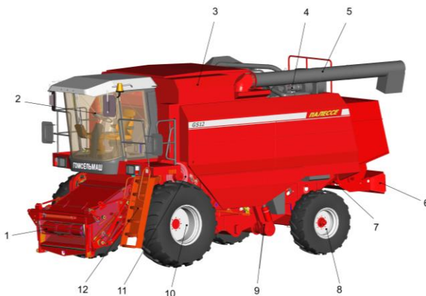
Рис. 10. Молотилка самоходная:
