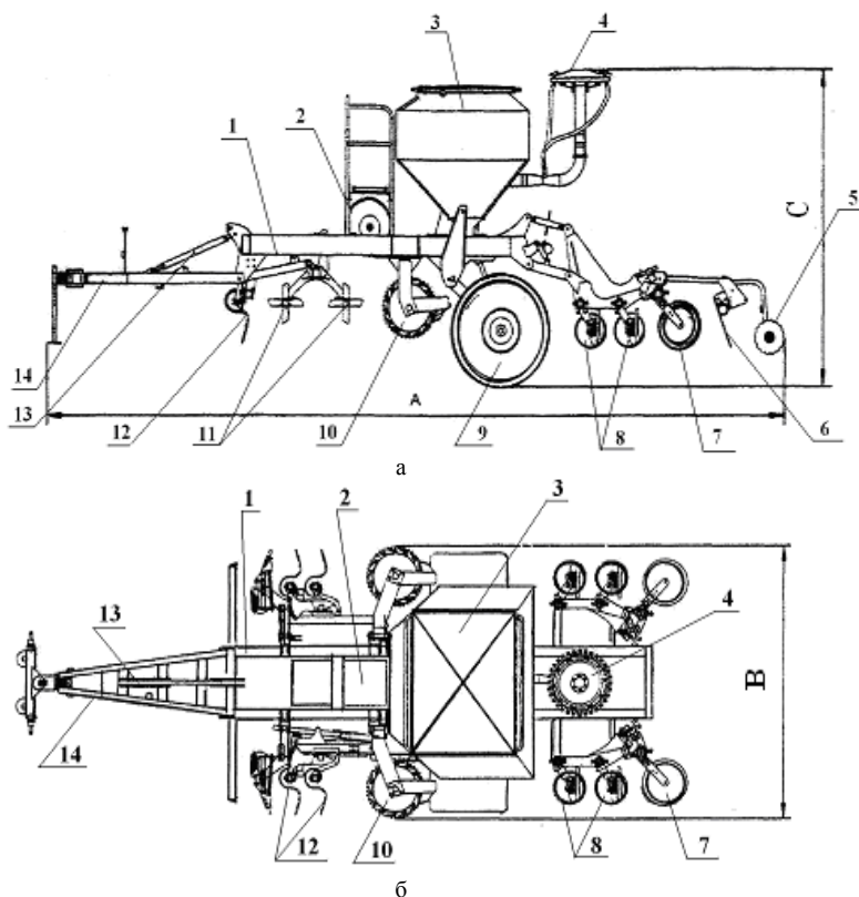
Рис. 5. Комбинированная сеялка MegaSeed: а – вид сбоку; б – вид сверху;
