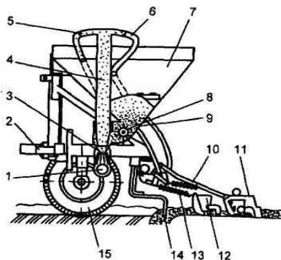
Рис. 2. Технологическая схема сеялки СПУ-6: 1 – вентилятор; 2 – рама; 3 – диффузор; 4 – вертикальный семьявоздухопровод; 5 – распределительная головка; 6 – отдельный семьявоздухопровод; 7 – бункер; 8 – катушка-дозатор; 9 – семена; 10 – семянаправитель; 11 – сошник; 12 – клапан; 13 – регулировочная пружина; 14 – рыхлитель колеи колес; 15 – опорно-приводное колесо
