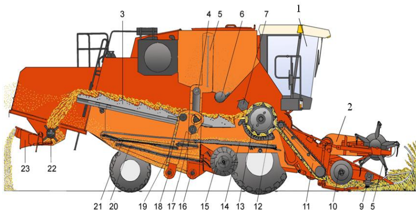
Рис. 13. Схема технологического процесса работы комбайна ПАЛЕССЕ GS812: 1 – кабина с блоком управления; 2 – жатка для зерновых культур; 3 – соломотряс; 4 – элеватор зерновой; 5 – шнек загрузной зерновой; 6 – шнек горизонтальный; 7 – битер отбойный; 8 – мотовило; 9 – режущий аппарат; 10 – шнек; 11 – транспортер наклонной камеры; 12 – подбарабанье; 13 – молотильный барабан; 14 – стрясная доска; 15 – вентилятор; 16 – шнек зерновой; 17 – устройство домолачивающее; 18 – шнек колосовой; 19 – элеватор колосовой; 20 – стан решетный нижний; 21 – стан решетный верхний; 22 – соломоизмельчитель; 23 – дефлектор
