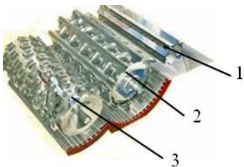
Рис. 18. Схема системы обмолота с барабаном-ускорителем зерноуборочного комбайна ПАЛЕКСЕ GS14: 1 – отбойный битер; 2 – молотильный аппарат; 3 – барабан-ускоритель
