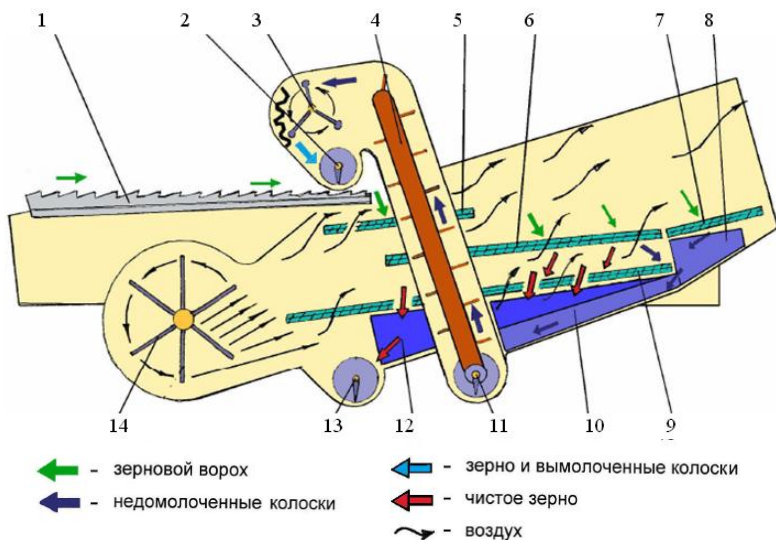
Рис. 8. Схема работы системы очистки зерноуборочного комбайна «ПАЛЕССЕ GS12»:
