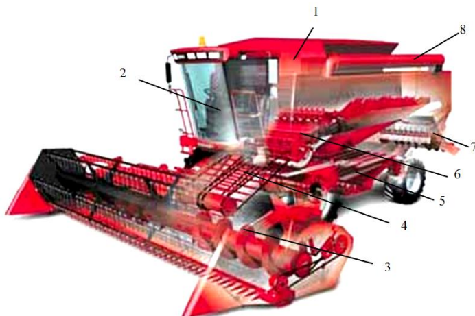
Рис. 16. зерноуборочный комбайн «Лида-1600»: 1 – бункер зерновой; 2 – площадка с кабиной управления; 3 – жатка; 4 – наклонная камера; 5 – очистка; 6 – молотильный аппарат; 7 – соломоизмельчитель; 8 – шнек выгрузной
