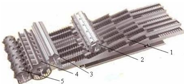
Рис. 19. Соломотряс зерноуборочного комбайна ПАЛЕКСЕ GS14: 1 – клавиши соломотряса; 2 – активатор; 3 – отбойный бiter; 4 – молотильный аппарат; 5 – барабан-ускоритель
