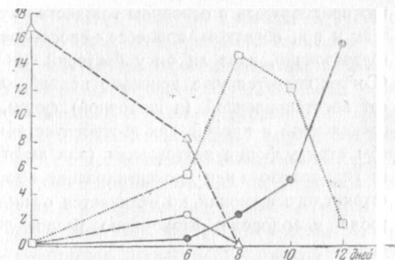
Рис. 10. Ход процесса денитрификации Δ — нитратный азот, ○ — азот нитритов, ● — свободный азот ( \text{N}_2 ), □ — неизвестное промежуточное соединение (гипонитриты?) (опыт М. П. Корсаковой)
