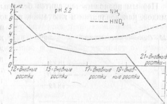
Рис. 23. Влияние возраста этиолированных ростков гороха на поглощение аммиачного и нитратного азота из раствора \text{NH}_4\text{NO}_3
