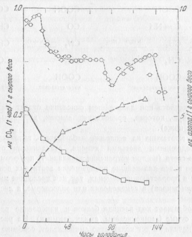
Рис. 7. Изменения в содержании неперевариваемого и общего растворимого азота в голодающих листьях ячменя и средняя скорость образования \text{CO}_2 . — \text{CO}_2 , \square — общий неперевариваемый азот, \triangle — общий растворимый азот (опыт Уетт)
