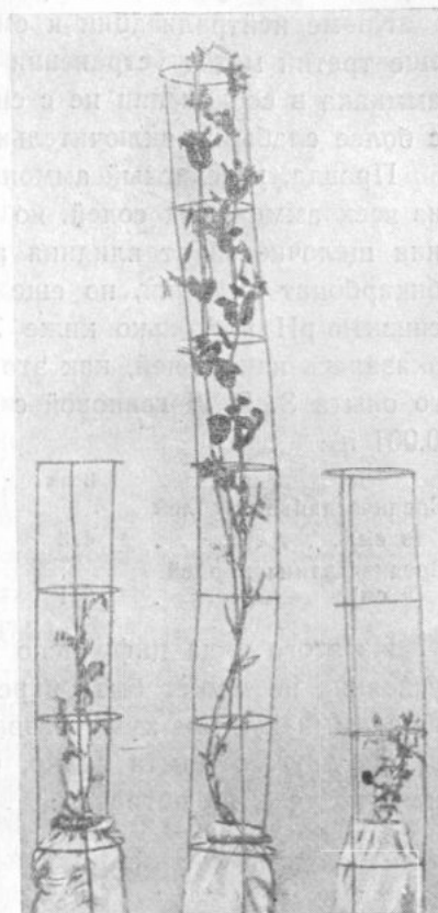
Рис. 12. Влияние смены раствора при питании (\text{NH}_4)_2\text{SO}_4 I — без смены раствора, II — при смене раствора, III — без смены раствора (\text{NH}_4)_2\text{SO}_4 + \text{CaCO}_3
