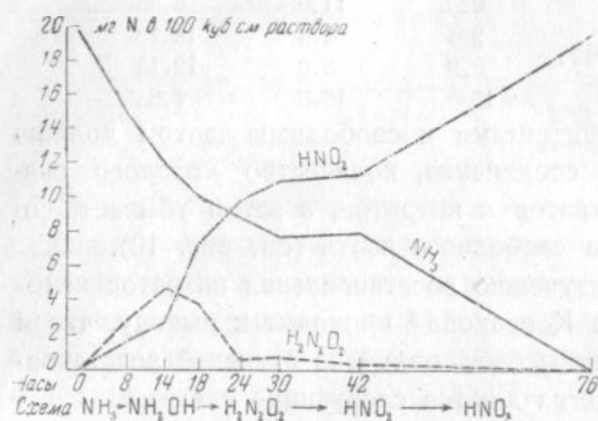
Рис. 11. Образование гипонитритов в процессе нитрификации (опыт Corbet с Nitrosomonas )
