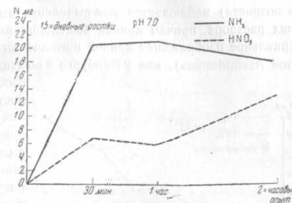
Рис. 20. Влияние продолжительности опыта на поглощение аммиачного и нитратного азота этиолированными ростками гороха 15-дневного возраста
