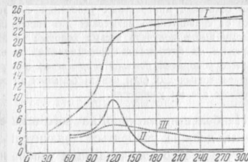
Рис. 34. Действие возрастающих доз \text{NH}_4\text{NO}_3 на урожай хлопка-сырца I — прибавка сырца, II — оплата урожая каждой вновь вводимой единицы удобрения, III — средняя оплата урожая единицы удобрения
