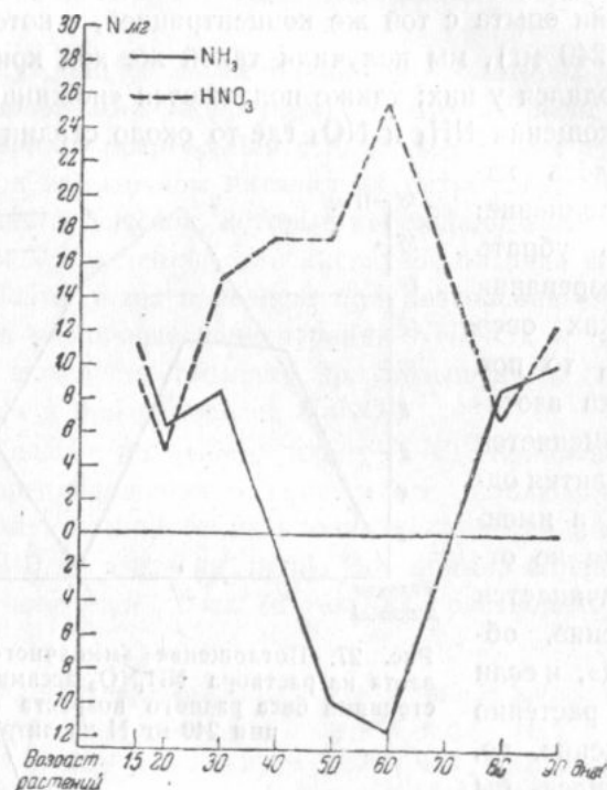
рис. 28. Поглощение аммиачного и нитратного азота из раствора \text{NH}_4\text{NO}_3 ассимилирующими растениями овса разного возраста (при концентрации 480 мг N на литр)
