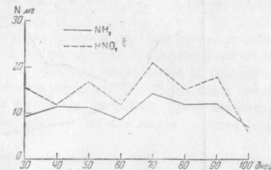
Рис. 29. Поглощение аммиачного и нитратного азота из раствора \text{NH}_4\text{NO}_3 . Состав питательной смеси по Naftel (опыт с хлопчатником)
