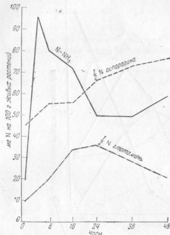
Рис. 9. Синтез глутамина и аспарагина в листьях ржи после инфильтрации глутаминовокислого аммония (опыт Mothes)
