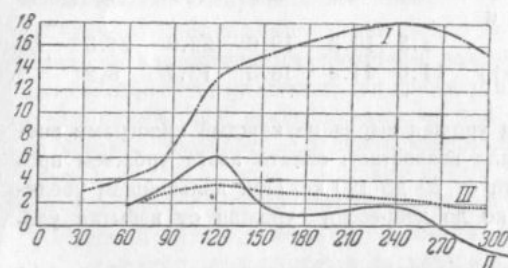
Рис. 35. Действие возрастающих доз (\text{NH}_4)_2\text{SO}_4 на урожай хлопка-сырца I — прибавка урожая сырья, II — оплата урожая каждой вновь вводимой единицы удобрения, III — средняя оплата урожая единицы удобрения
