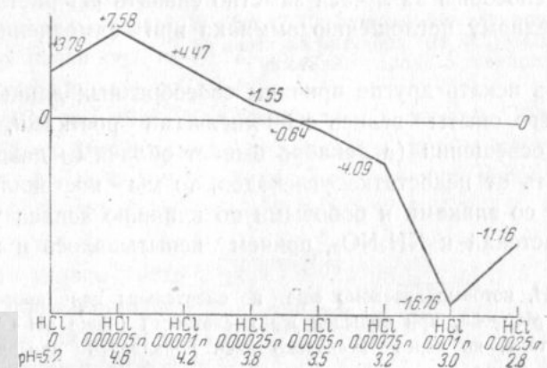
Рис. 16. Влияние pH раствора \text{NH}_4\text{H}_2\text{PO}_4 на поглощение и выделение аммиака проростками гороха
