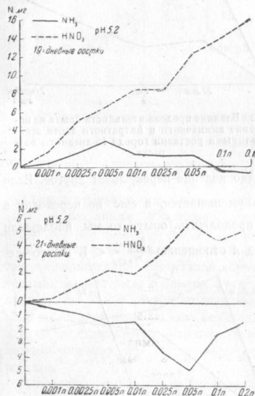
Рис. 22. Влияние концентрации раствора \text{NH}_4\text{NO}_3 на поглощение аммиачного и нитратного азота этиолированными ростками гороха 19-дневного и 21-дневного возраста
