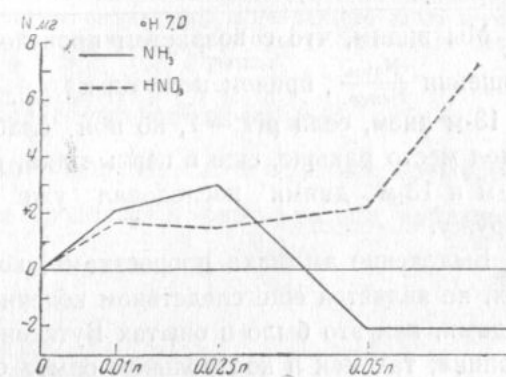
Рис. 19. Влияние концентрации раствора \text{NH}_4\text{NO}_3 на поглощение аммиачного и нитратного азота 15-дневными этиолированными ростками сахарной свеклы
