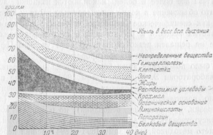
Рис. 2. Превращение веществ при прорастании семян вики
