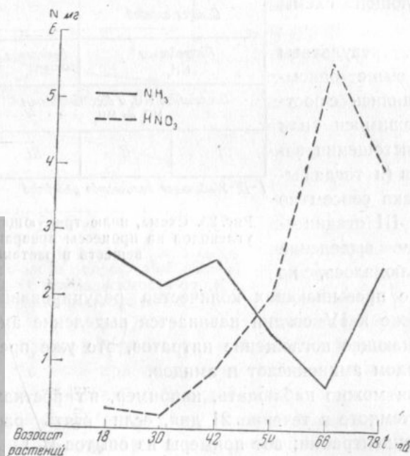
Рис. 26. Влияние возраста ассимилирующих растений овса на поглощение нитратного и аммиачного азота из раствора \text{NH}_4\text{NO}_3 (опыт Сталя и Шайва)
