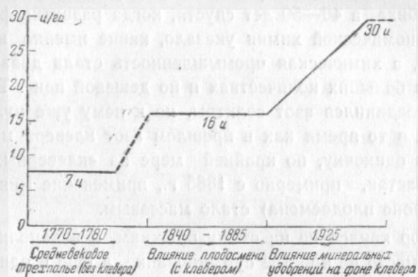
Рис. 33. Изменение уровня урожаев пшеницы в Западной Европе за 150 лет (схема)
