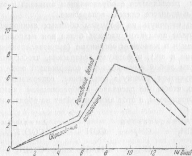
Рис. 4. Суточная скорость распада белка и образования аспарагина
