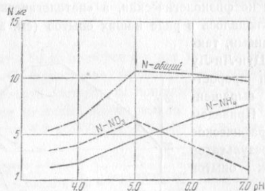
Рис. 32. Поглощение аммиачного и нитратного азота из раствора \text{NH}_4\text{NO}_3 при различных pH (по Naphtel)
