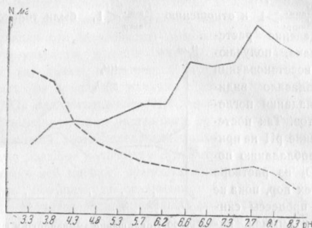
Рис. 31. Поглощение аммиачного и нитратного азота из раствора \text{NH}_4\text{NO}_3 при различных pH (по данным опытов Tsung - Lee - Loo) — \text{NH}_3 , — \text{HNO}_3
