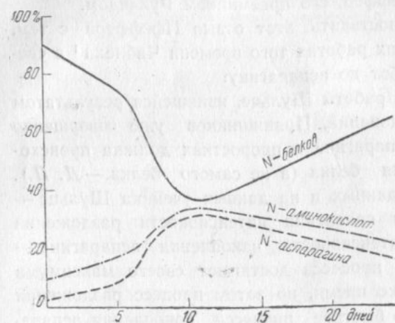
Рис. 5. Регенерация белков на свету (опыт с Lupinus luteus )
