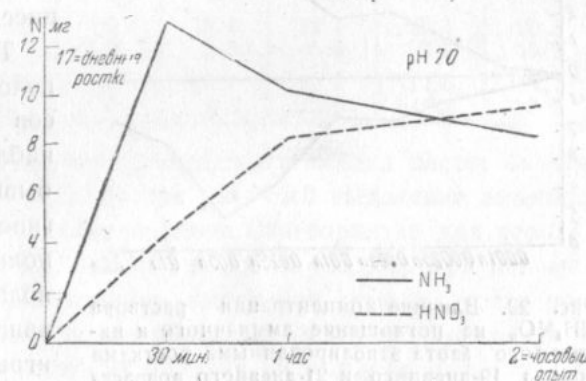
Рис. 21. Влияние продолжительности опыта на поглощение аммиачного и нитратного азота этиолированными ростками гороха 17-дневного возраста
