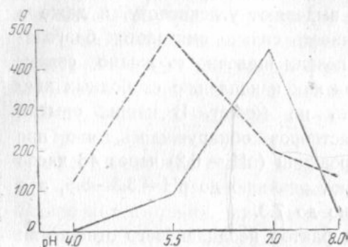
Рис. 13. Вес корней сахарной свеклы при различных величинах pH и питании аммиачным (сплошная линия) и нитратным (пунктирная линия) азотом
