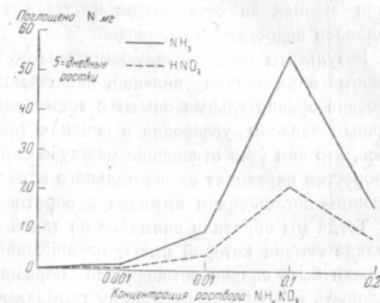
Рис. 17. Поглощение аммиачного и нитратного азота из раствора \text{NH}_4\text{NO}_3 этиолированными ростками гороха 5-дневного возраста
