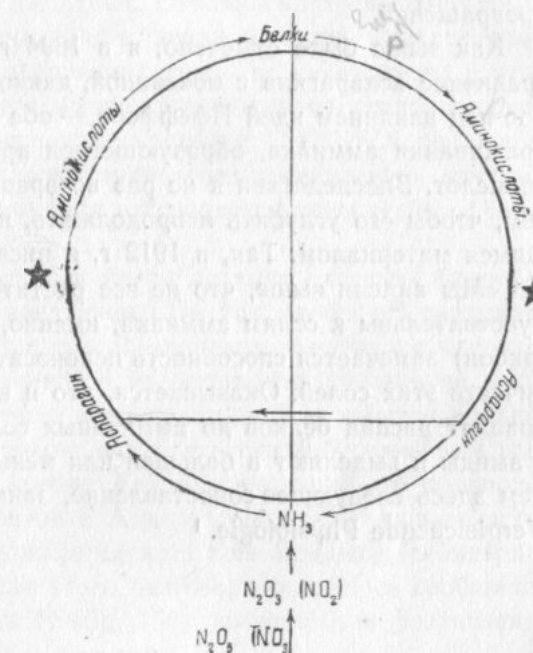
Рис. 6. Схема превращений азотистых веществ в растении
