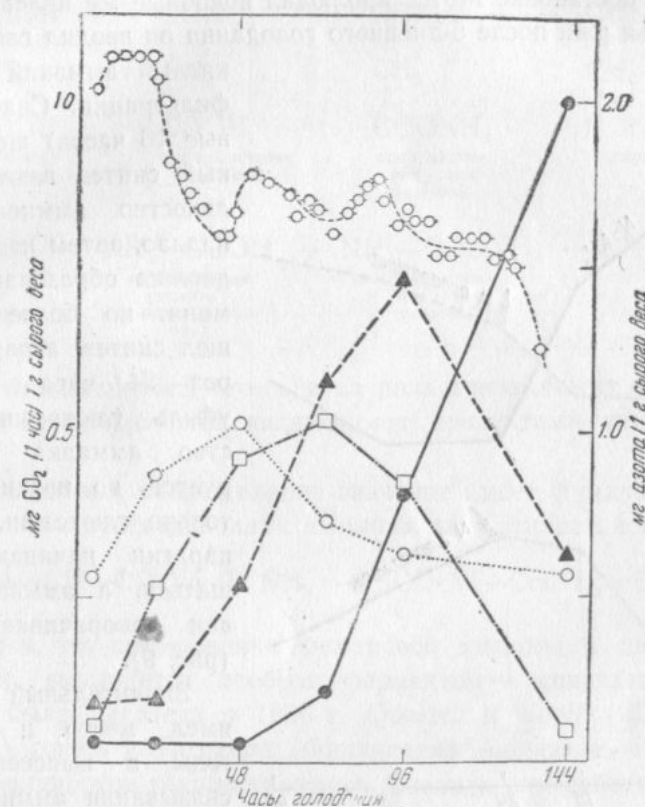
Рис. 8. Изменения в содержании аминокислотного, амидного и аммиачного азота в голодающих листьях ячменя и средняя скорость образования \text{CO}_2 . — \text{CO}_2 , \square — азот аминокислот, \square — неустойчивый амидный азот (глутамин), \triangle — устойчивый амидный азот (аспарагин), \bullet — аммиачный азот (опыт Уетт)
