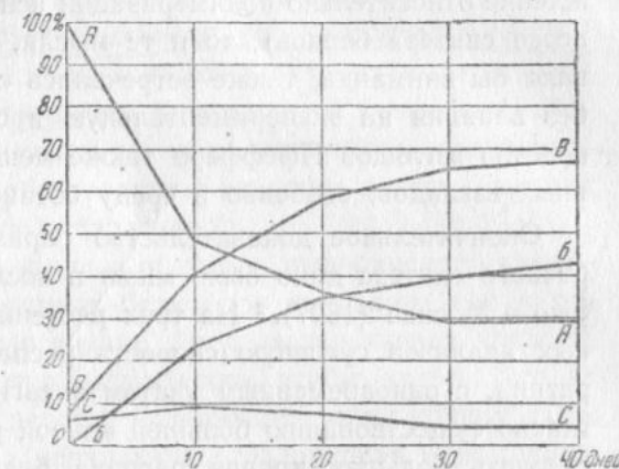
Рис. 3. Обмен азотистых веществ при прорастании семян вики. Линия AA соответствует азоту белков, BB — сумме азота аминокислот и амидов, CC — азоту органических оснований и cc — азоту аспарагина (в процентах от общего количества азота)
