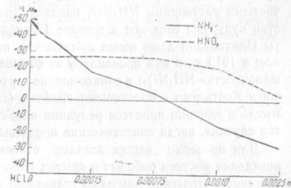
Рис. 15. Влияние концентрации кислоты на поглощение нитратного и аммиачного азота проростками гороха
