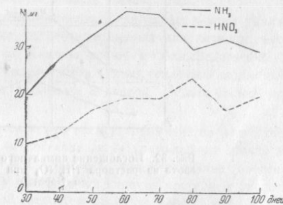
Рис. 30. Поглощение аммиачного и нитратного азота из раствора \text{NH}_4\text{NO}_3 . В питательной смеси увеличена концентрация кальция (опыт с хлопчатником)
