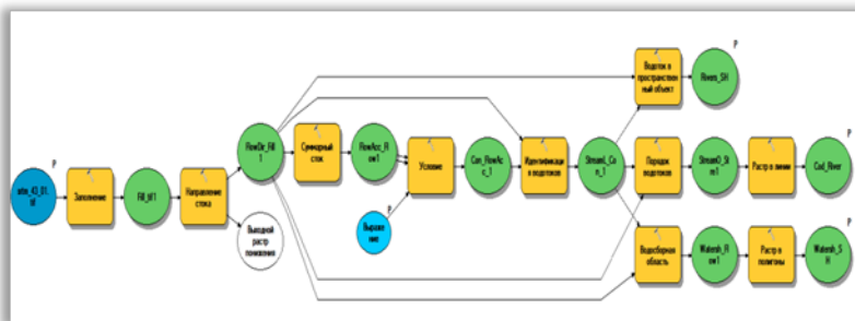
Рис. 1. Модель, позволяющая моделировать систему водотоков и их бассейнов, созданная с помощью приложения Model Builder (в модели синим цветом обозначены исходные данные, желтым – процесс, зеленым – результат)
