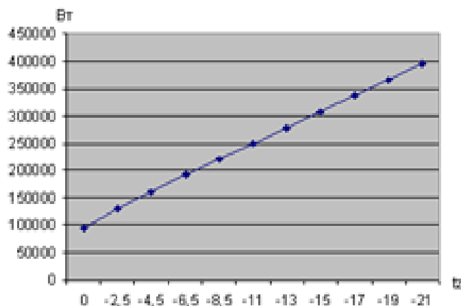
Рис. 1. Зависимость расхода тепла на нагрев птичника от температуры на улице, до установки на объект теплообменника
