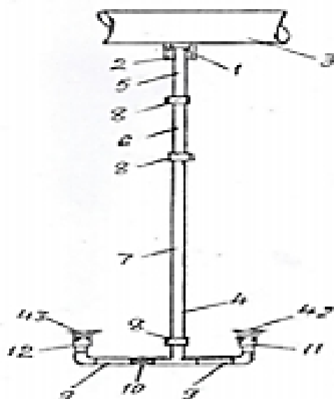
Рис. 2. Фрагмент напорного трубопровода дождевальной машины (вид сбоку) и возможное положение горизонтальной трубки с диффузором с дождевателями-опрыскивателями
