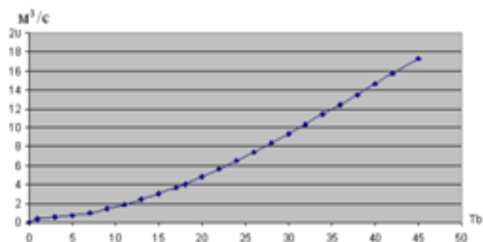
Рис. 3. График расхода вентиляционного воздуха в зависимости от возраста бройлеров
