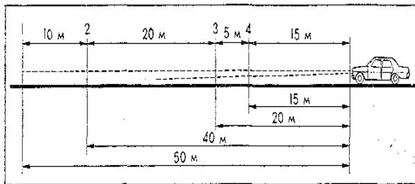
Рис. 11.10. Определение расстояний видимости световых приборов транспортного средства: 1 – дальний свет; 2 – ближний свет; 3 – подфарники; 4 – все приборы выключены
