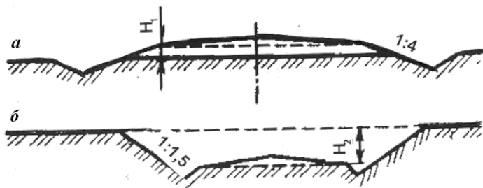
Рис. 4.3. Поперечные профили насыпи (а) и выемки (б): H_1 – высота насыпи; H_2 – глубина выемки
