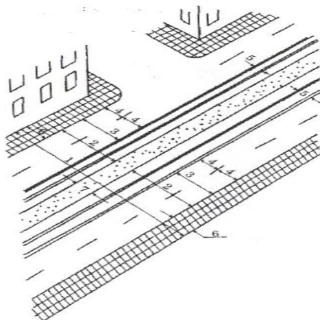
Рис. 4.4. Элементы улицы: 1 – общая ширина улицы; 2 – проезжая часть; 3 – проезжая часть для транспортных средств; 4 – полоса движения; 5 – трамвайный путь; 6 – тротуар; 7 – разделительная полоса
