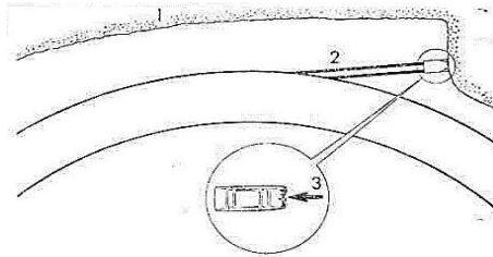
Рис. 3.26. Схема ДТП: 1 – насыпь и зеленые насаждения; 2 – следы шин; 3 – фронтальное повреждение автомобиля
