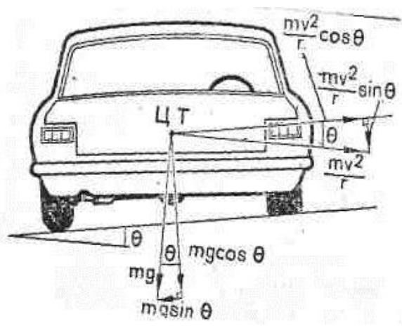
Рис. 8.23. Схема сил при движении по кривой с виражом
