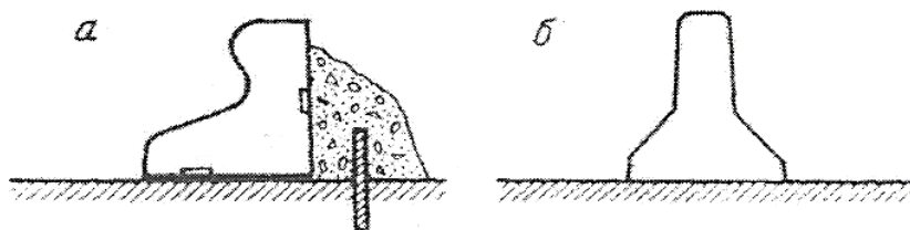
Рис. 4.16. Профили высоких бетонных ограждений: а – «Триэф»; б – «Нью-Джерси»
