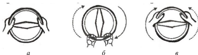
Рис. 3.12. Поворот рулевого колеса направо силовым способом: a – положение рук до начала поворота; б – правая рука поворачивает рулевое колесо, а левая скользит вниз; в – левая поворачивает, правая скользит вверх
