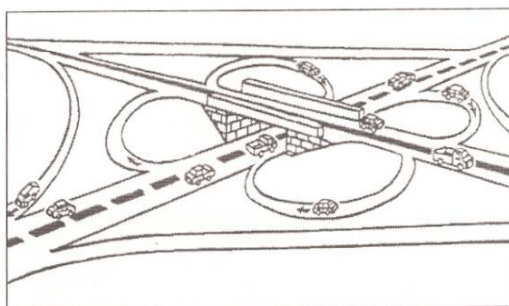
Рис. 4.12. Пересечение типа «клеверный лист»
