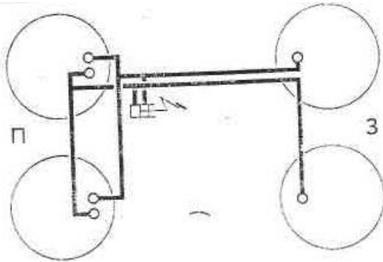
Рис. 3.30. Раздельный тормозной привод с включением в каждый контур тормозов
