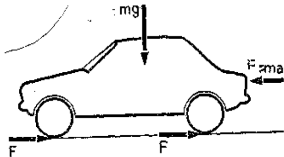
Рис. 3.32. Схема сил, действующих при торможении: mg – вертикальная сила; ma – горизонтальная сила; F – тормозная сила
