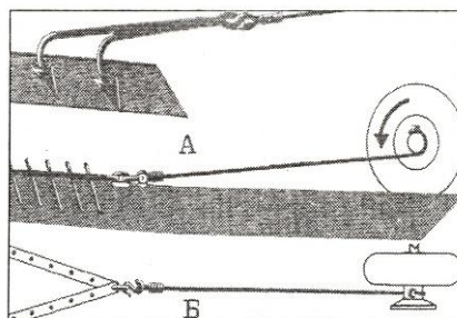
Рис. 8.15. Якоря для вытаскивания транспортного средства
