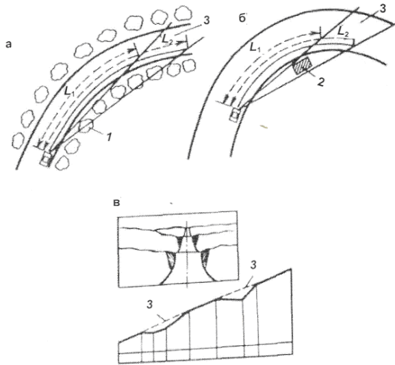
Рис. 8.3. Схемы ограничения обзорности: а – неправильное расположение посадок; б – неправильное расположение павильона на автобусной остановке; в – устройство частых переломов в продольном профиле (вид дороги в плане и профиле); 1 – посадки; 2 – павильон; 3 – зоны отсутствия обзорности; L_1 и L_2 – фактическое и необходимое расстояние обзорности соответственно
