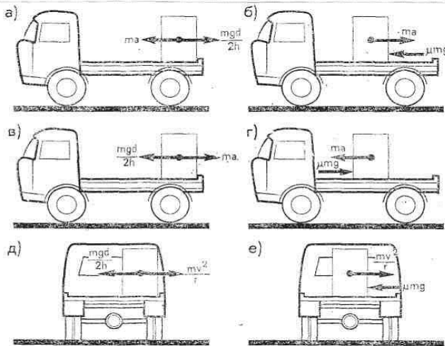
Рис. 3.34. Поведение груза при маневрировании транспортного средства: a – ускорение, груз опрокидывается; б – ускорение, груз сдвигается; в – замедление, груз опрокидывается; г – замедление, груз сдвигается; д – движение по кривой, груз опрокидывается; е – движение по кривой, груз сдвигается
