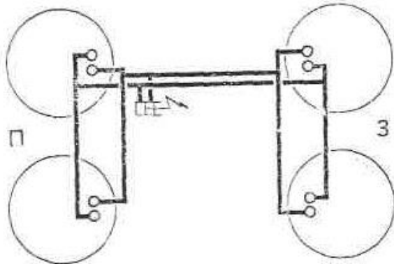
Рис. 3.31. Двойная тормозная система
