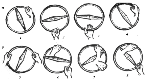
Рис. 3.13. Поворот рулевого колеса направо скоростным способом, выполняемый одной рукой (а) и поочередно двумя руками (б) с перехватами: 1 – положение рук до начала поворота рулевого колеса; 2 – поворот рулевого колеса направо до момента начала осуществления перехвата через тыльную сторону кисти; 3 – поворот рулевого колеса направо, осуществляемый одновременно с перехватом руки через тыльную сторону кисти; 4 – поворот рулевого колеса направо после перехвата руки; 5 – положение рук до начала поворота рулевого колеса; 6 – поворот рулевого колеса направо до момента начала осуществления перехвата правой рукой и продолжение поворота левой; 7 – поворот рулевого колеса направо левой рукой с одновременным перехватом правой; 8 – поворот рулевого колеса направо правой рукой с одновременным перехватом левой
