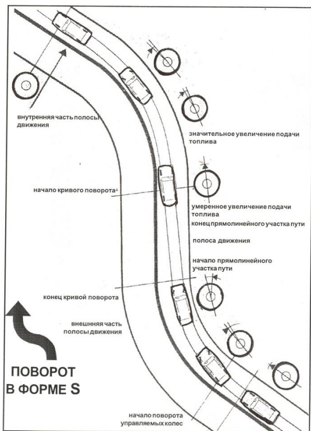
Рис. 8.21. Поворот в форме S
