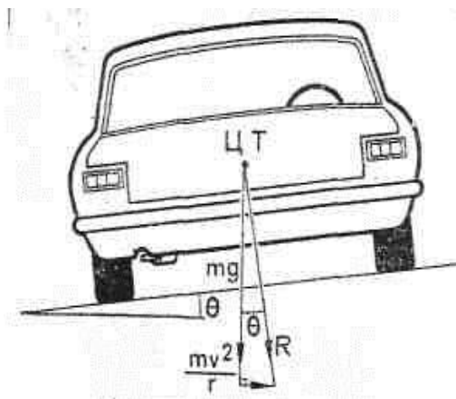
Рис. 8.26. Схема для установления максимальной скорости для данного угла поперечного уклона виража
