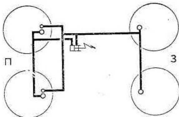
Рис. 3.29. Схема раздельного тормозного привода с двумя рабочими цилиндрами на каждом тормозе передних колес
