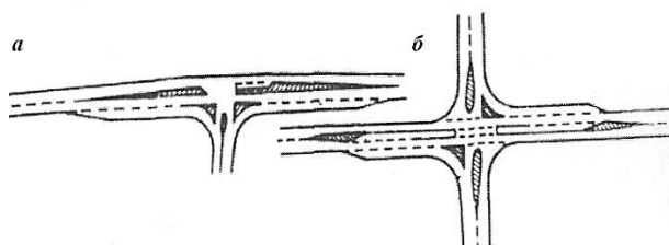
Рис. 4.7. Пересечение (а) и примыкание (б) дорог с канализованным движением в одном уровне
