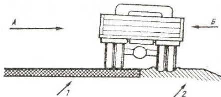
Рис. 8.33. Направление возможного заноса при резком увеличении скорости (А) и резком торможении (Б): 1 – покрытие; 2 – обочина
