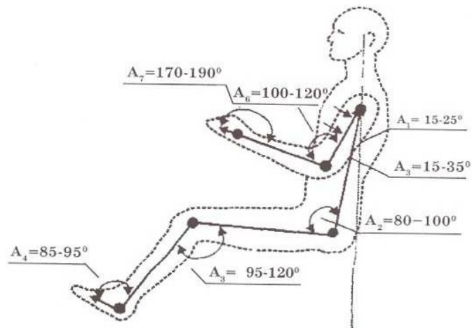
Рис. 3.4. Схема антропометрических показателей оптимальной рабочей посадки водителя
