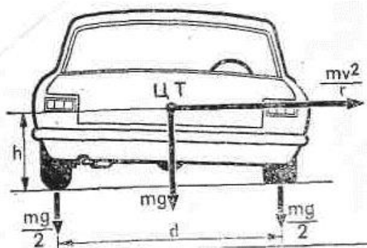
Рис. 8.24. Схема к определению скорости, при которой происходит опрокидывание, для случая движения по кривой при горизонтальной поверхности дороги
