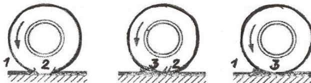
Рис. 8.31. Этапы возникновения аквапланирования: 1 – пленка воды на покрытии; 2 – зона контакта между шиной и покрытием; 3 – водяной клин
