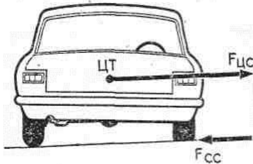
Рис. 8.22. Схема сил, возникающих при движении по кривой с горизонтальной поверхностью дороги:
