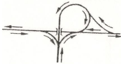
Рис. 4.14. Схема примыкания автомобильных дорог по типу «труба»
