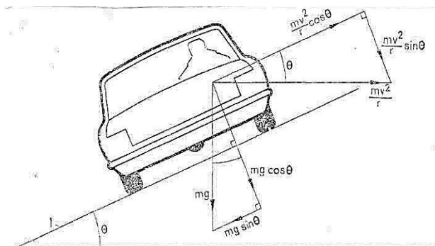
Рис. 8.28. Схема движения с критической скоростью: l – поверхность дороги
