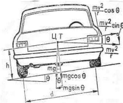
Рис. 8.25. Схема к определению скорости, при которой происходит опрокидывание, для случая движения по кривой с виражом
