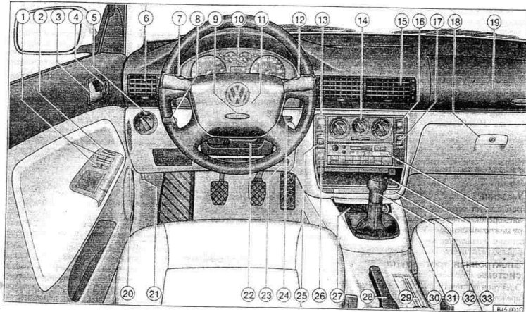
Рис. 3.1. Общий вид места водителя легкового автомобиля:
