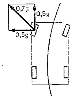
Рис. 3.25. Схема сил, действующих на автомобиль при торможении на повороте
