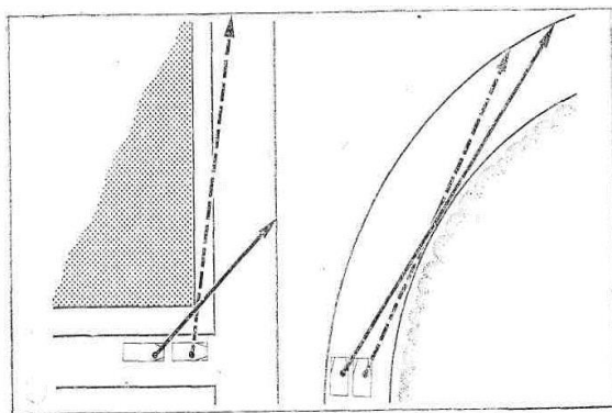
Рис. 11.2. Схемы зависимости расстояния видимости от положения транспортного средства
