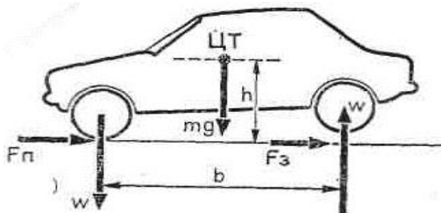
Рис. 3.33. Схема перераспределения массы автомобиля при торможении: ЦТ – центр тяжести
