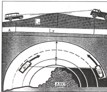
Рис. 8.16. Условия обзорности дороги: А – на участке с переменным продольным профилем; Б – на криволинейном участке дороги
