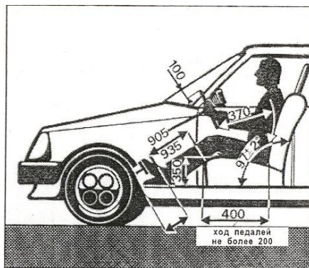
Рис. 3.5. Правильно установленное и отрегулированное сиденье водителя
