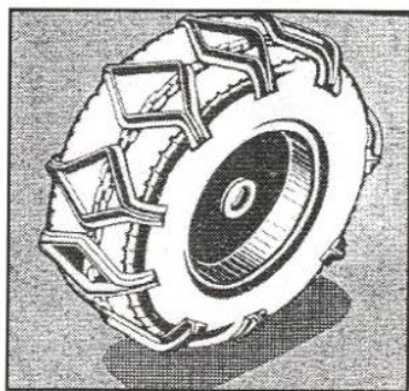
Рис. 8.9. Цепи с ромбовидными траками
