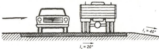
Рис. 8.32. Направление наиболее вероятного смещения транспортного средства при заносе на проезжей части с односкатным профилем: i_1 – поперечный уклон обочины; i_2 – поперечный уклон проезжей части
