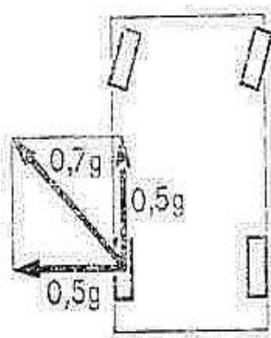
Рис. 3.23. Схема сил, действующих на автомобиль с силовым приводом на задние колеса при ускорении на повороте
