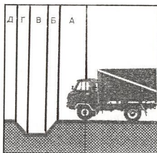
Рис. 8.5. Схема преодоления препятствия в виде канав или ям
