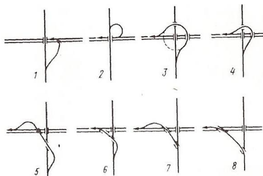
Рис. 4.8. Типы левоповоротных съездов на транспортных развязках: 1 – съезд на неполных развязках; 2 – петлевой съезд на развязках типа «клеверный лист»; 3, 4 – съезды с использованием распределительного кольца; 5, 6 – полупрямые съезды; 7, 8 – прямые съезды
