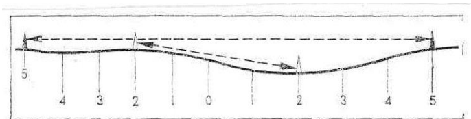
Рис. 11.5. Линии прямой видимости на дороге с неровным продольным профилем
