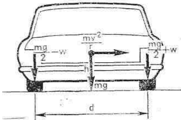
Рис. 8.27. Перераспределение нагрузки на повороте
