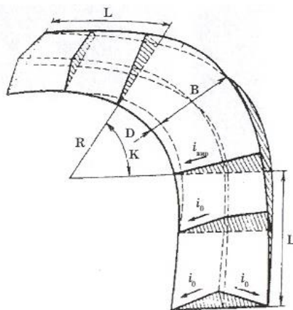
Рис. 4.1. Схема виража: i_{\text{вир}} и i_0 – поперечные уклоны соответственно на вираже и на переходной кривой; L – участок отгона виража и переходная кривая; D – уширение; K – круговая кривая; B – ширина проезжей части; R – радиус круговой кривой
