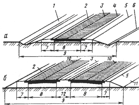
Рис. 4.2. Элементы поперечного профиля дороги: а – с одной проезжей частью; б – с двумя проезжими частями и разделительной полосой; 1 – внешний откос канавы; 2 – укрепленная полоса обочины; 3 – ось дороги; 4 – кромка проезжей части; 5 – бровка земляного полотна; 6 – внутренний откос; 7 – обочина; 8 – проезжая часть; 9 – земляное полотно; 10 – ось проезжей части; 11 – откос насыпи; 12 – разделительная полоса
