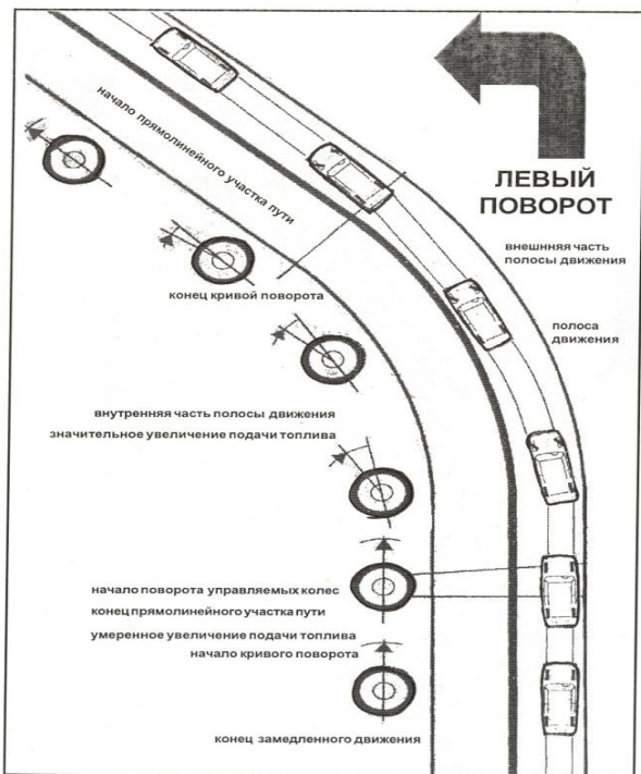
Рис. 8.18. Левый поворот
