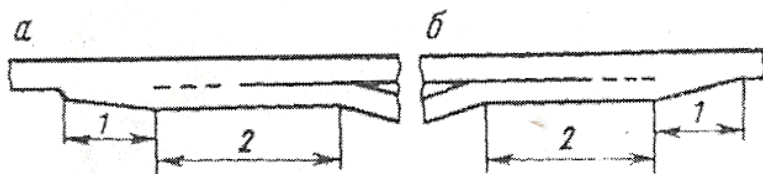
Рис. 4.15. Схема переходно-скоростных полос: а – торможения; б – разгона; 1 – отгон переходно-скоростной полосы; 2 – длина полосы для разгона и торможения
