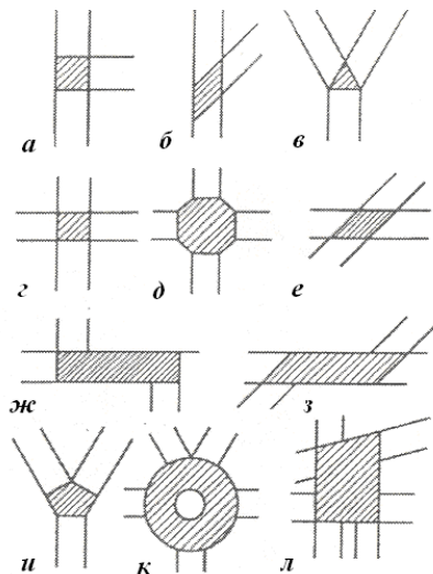
Рис. 4.5. Формы пересечения дорог
