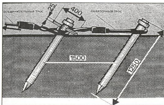
Рис. 8.14. Упоры для вытаскивания транспортного средства
