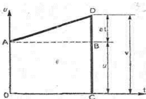
Рис. 2.3. График ускорения
