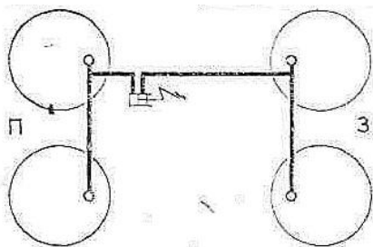
Рис. 3.27. Схема раздельного привода тормозов передних (П) и задних (З) колес
