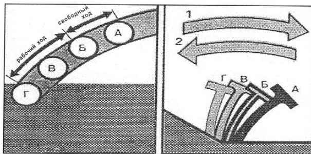
Рис. 3.16. Свободный и рабочий ход педали
