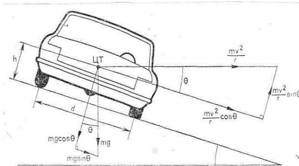
Рис. 8.30. Силы, действующие на транспортное средство при опрокидывании и заносе на кривой с отрицательным поперечным уклоном дороги
