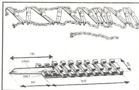
Рис. 8.10. Цепи с косым расположением траков
