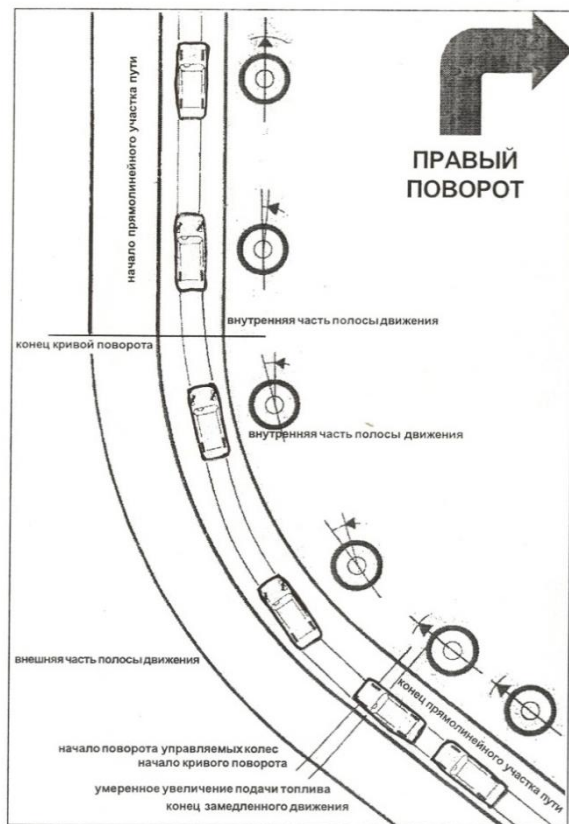
Рис. 8.17. Правый поворот
