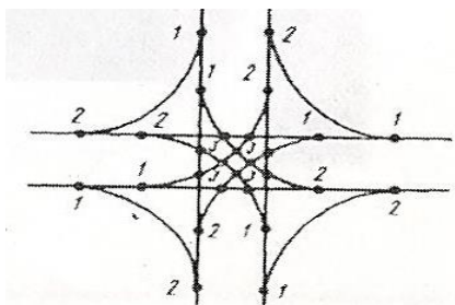
Рис. 4.6. Конфликтные точки на пересечениях дорог в одном уровне: 1 – разделение транспортных потоков; 2 – слияние транспортных потоков; 3 – пересечение транспортных потоков
