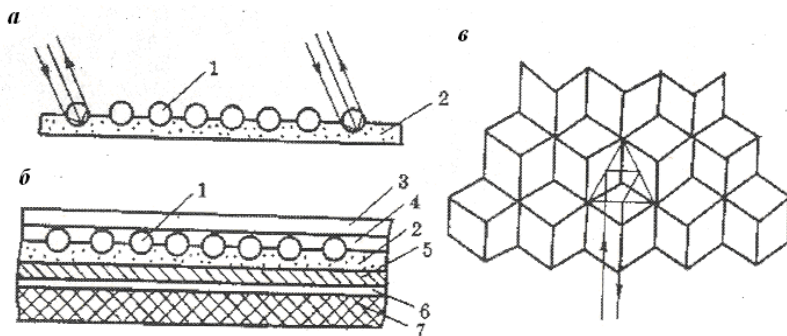
Рис. 3.36. Конструкция световозвращателей: а – простейший; б – пленочный закрытый; в – плоскопризмный; 1 – шаровая линза; 2 – слой порошкообразного алюминия; 3 – защитная пленка; 4 – связывающий слой; 5 – фольга; 6 – слой клея; 7 – бумажное основание
