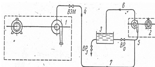
Рис. 7.6. Гидромеханическая схема соединения вакуум-установки с основным насосом: ВР 0 – ручной вентиль открытый; ВР 3 – ручной вентиль закрытый; ВЭМ – электромагнитный вентиль; 1 – насос; 2 – вакуум-установка; 3 – бачок; 4 – устройство для контроля уровня или тока воды; 5 – всасывающий трубопровод; 6 – нагнетательный трубопровод; 7 – слив
