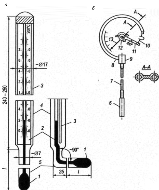
Рис. 3.12. Термометры: а – технический жидкостный стеклянный; б – показывающий манометрический
