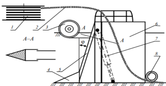
Рис. 11.4. Схема рабочего органа дреноукладчика МД-12:
