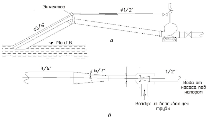
Рис. 7.3. Вариант приподнятой всасывающей трубы в комбинации с эжектирующим устройством: а – общий вид; б – схема эжектора
