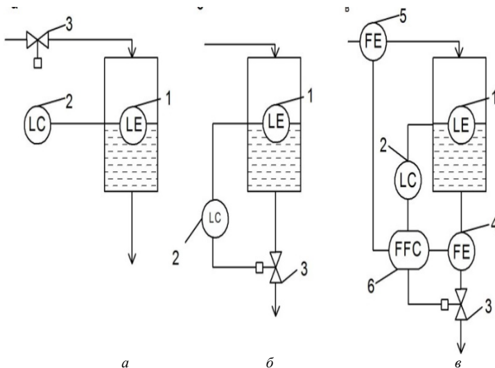
Рис. 4.16. Схемы непрерывного регулирования уровня: а – регулирование «на притоке»; б – регулирование «на стоке»; в – каскадная АСР; 1 – измеритель уровня; 2 – регулятор уровня; 3 – регулирующий клапан; 4, 5 – измерители расхода; 6 – регулятор соотношений
