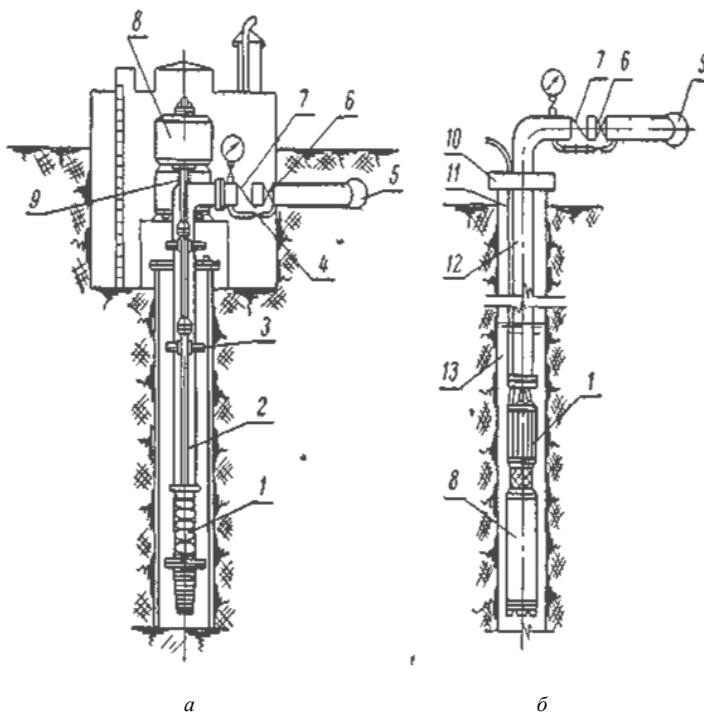
Рис. 8.1. Схема расположения насосной установки в скважине: а – оборудованной насосом типа АТН; б – оборудованной насосом типа АП; 1 – насос; 2 – приводной вал; 3 – резиновый подшипник; 4 – обводная труба; 5 – магистральный трубопровод; 6 – задвижка; 7 – обратный клапан; 8 – электродвигатель; 9 – опорный подшипник; 10 – опорная плита; 11 – кабель; 12 – водоподъемная труба; 13 – обсадная труба
