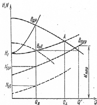
Рис. 7.11. Сравнение экономичности разных способов регулирования подачи центробежных насосов
