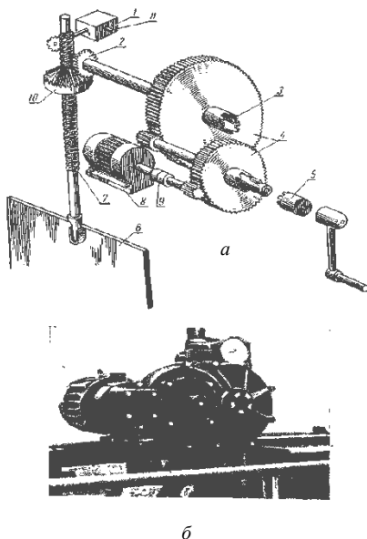
Рис. 9.2. Винтовой подъемный механизм серии ВУП:
