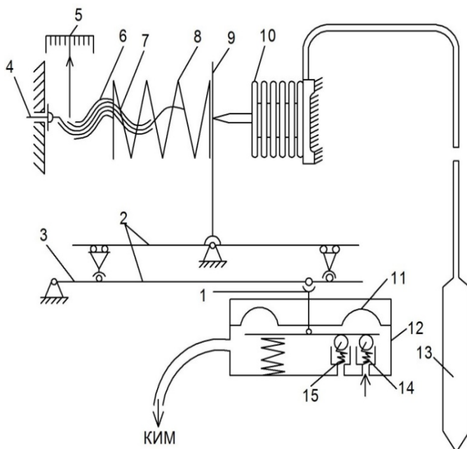
Рис. 4.7. Схема пневматического П-регулятора температуры с манометрической термосистемой: 1 – шток пневмореле; 2 – узел неравномерности; 3, 9 – рычаги; 4, 7 – винты; 5 – шкала; 8 – пружина; 10 – сильфон; 11 – мембрана; 12 – пневмореле; 13 – термобаллон; 14 – питающий клапан; 15 – стравливающий клапан
