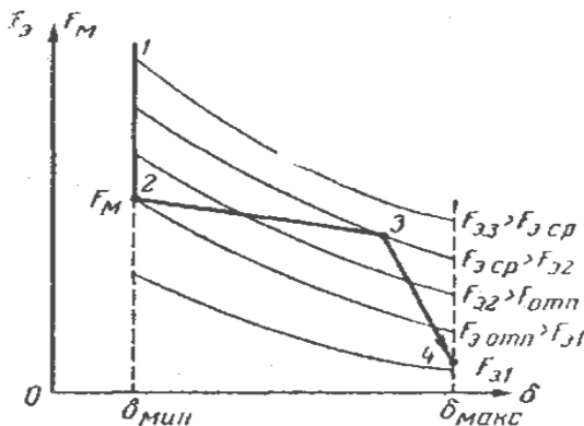
Рис. 5.8. Тяговые F_{\Sigma} и механическая F_M характеристики электромагнитного реле
