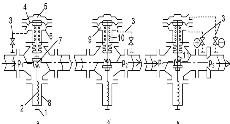
Рис. 4.10. Принципиальные схемы включения регулятора типа УРРД: а – регулирование давления «до себя»; б – регулирование давления «после себя»; в – регулирование перепада давления или расхода; 1 – винт; 2 – пружина; 3 – импульсная трубка; 4 – мембрана; 5, 6 – исполнительный механизм; 7 – регулирующий орган; 8 – стакан; 9 – камеры; 10 – пружины; 11 – шток
