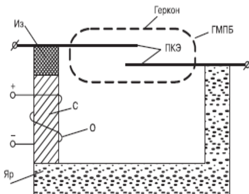
Рис. 5.11. Схема ЭМР с МУК и замкнутой магнитной цепью:
