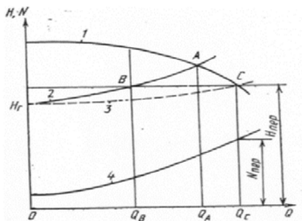
Рис. 7.9. Регулирование подачи центробежного насоса перепуском
