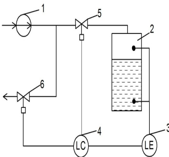
Рис. 4.15. Схема позиционного регулирования уровня: 1 – насос; 2 – аппарат; 3 – сигнализатор уровня; 4 – регулятор уровня; 5, 6 – регулирующие клапаны
