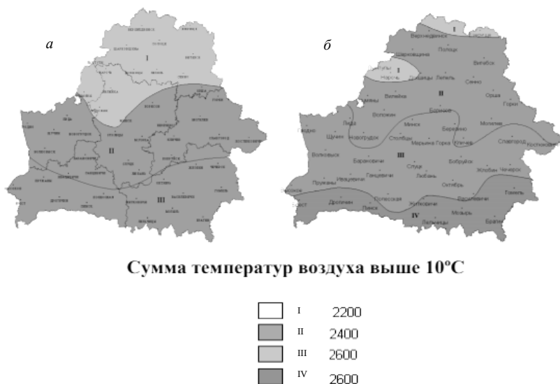
Рис. 1.1. Перемещение агроклиматических зон: а – Границы агроклиматических областей по А. Х. Шкляру (1973 г.); б – Границы агроклиматических областей за период потепления 1989–2015 гг.; I – Северная, II – Центральная, III – Южная, IV – Новая
