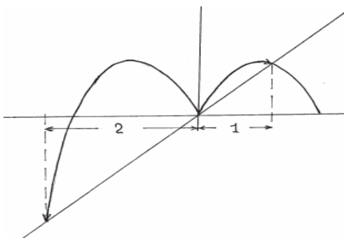
Рис. 10.2. Разбрызгивание почвывкаплями дождя на 450
