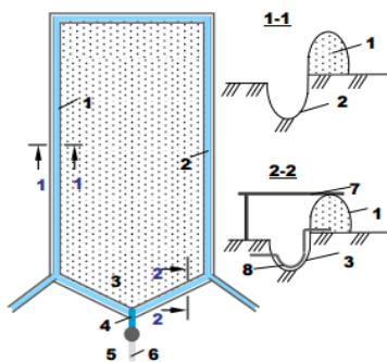
Рис. 10.3. Схема стоковой площадки: 1 – бортик площадки; 2 – водоотводящие канавки; 3 – водопримемная канавка; 4 – водоподводящий лоток; 5 – измерительная емкость; 6 – сбросная канавка; 7 – защитный козырек; 8 – полиэтиленовая пленка
