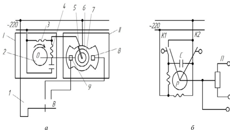
Рис. 6.3. Исполнительные механизмы с электродвигательным приводом: а — типа ДР-1М; б — типа ПР; I — конденсаторный двигатель; II — контактное управляющее устройство; 1 — контактный датчик; 2 — ротор двигателя; 3, 4 — статорные обмотки двигателя; 5 — ползунок контактного управляющего устройства; 6, 7 — контактные пластины; 8, 9 — контакты; С — конденсатор; K1, K2 — конечные выключатели; П — резистивный датчик положения; В — выключатель
