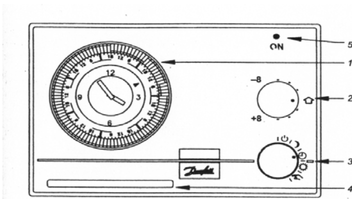
Рис. 4.8. Погодный компенсатор ECL с настройкой доступной потребителю
