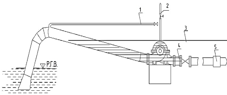
Рис. 7.2. Схема приподнятой всасывающей трубы и воздухоотводящей трубы: 1 – воздухоотводящая трубка; 2 – клапан для первоначальной заливки насоса и всасывающей трубы и для выпуска воздуха; 3 – нижняя кромка приподнятого колена и верх корпуса насоса; 4 – задвижка; 5 – обратный клапан; Р.Г.В. – расчетный горизонт воды
