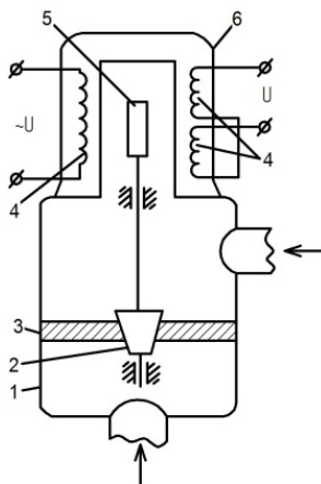
Рис. 3.8. Ротаметр с дифференциально-трансформаторным преобразователем:
