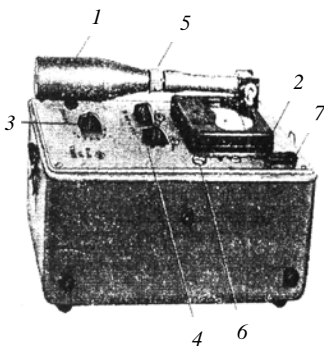
Рис. 23. Шумомер Ш-63
