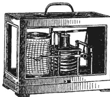
Рис. 9. Барограф М-22С
