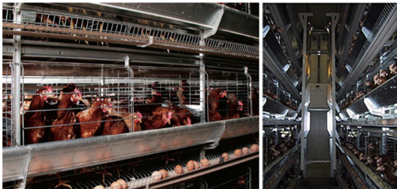
Рис. 43. Клеточная батарея для кур-несушек
