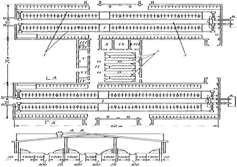
План коровника для боксового содержания на 400 гол.
