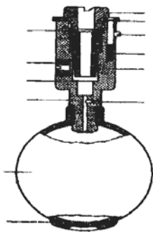
Рис. 20. Универсальный газоанализатор фирмы «Хехст»
