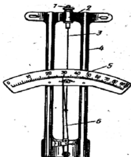
Рис. 12. Гигрометр МВ-18
