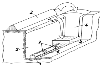
Рис. 4.5. Конструкция дрены:
