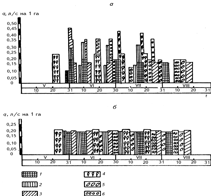
Рис. 5.4. Неукомплектованный (а) и укомплектованный (б) графики полива:
