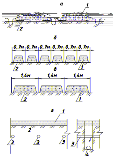
Рис. 4.18. Агромелиоративные мероприятия: а – узкозагонная вспашка; б – гребневание; в – грядование; з – кротование; 1 – пахотный слой; 2 – подпочва; 3 – кротовины; 4 – материальные дрены
