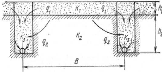
Рис. 4.12. Расчетная схема поступления воды в закрытые собиратели
