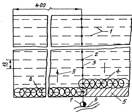
Рис. 5.10. Примерная схема полива ДКШ-64:
