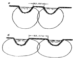
Рис. 5.19. Схемы контуров увлажнения почвы при поливе по бороздам: a – легкие почвы; б – тяжелые почвы
