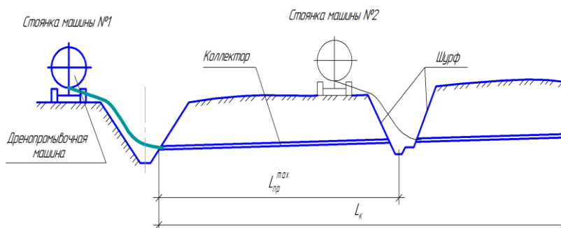
Рис. 4.45. Схема промывки дренажа дренопромывочной машиной
