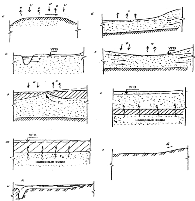
Рис. 3.2. Типы водного питания:
