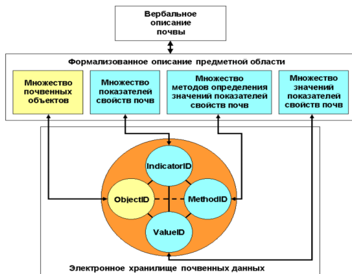
Рис. 1. Концептуальная схема цифровой модели описания почвенных данных
