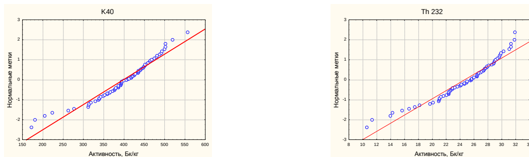
Рис.2. Нормальные графики активностей ^{40}\text{K} и ^{232}\text{Th}
