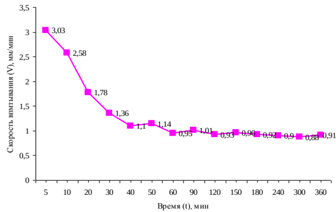
Рис. 2. График изменения скорости впитывания (опыт № 2 – орошаемый участок)
