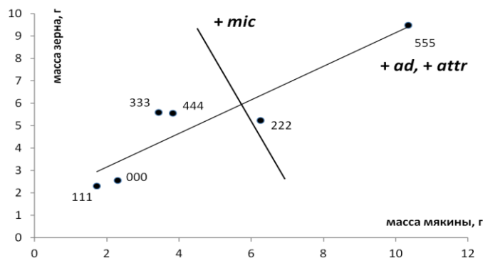
Рис. Графическое представление работы физиолого-генетических систем аттракции, адаптивности и микрораспределения ассимилятов у растений озимой ржи сорта Фаленская 4 при возрастающих дозах минеральных удобрений
