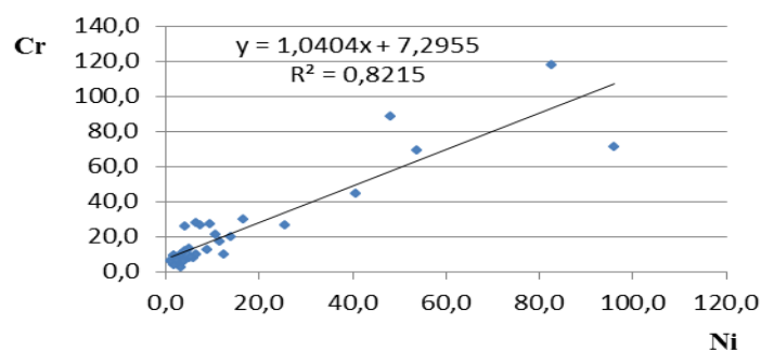
Рис. 3. Корреляция между Cr и Ni в золе растений пригородной зоны г. Молодечно
