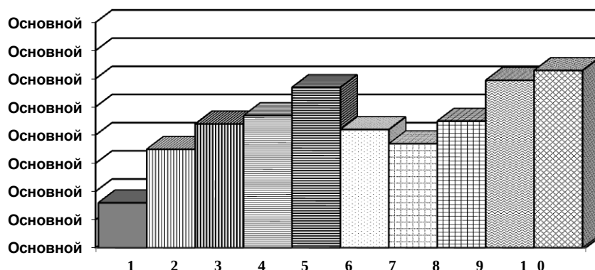
Рис. 2. Среднее содержание (мг/кг) подвижного фосфора за вегетационный период под подсолнечником в результате последствий горных пород, 2016 г. Условные обозначения как в рис. 1.
