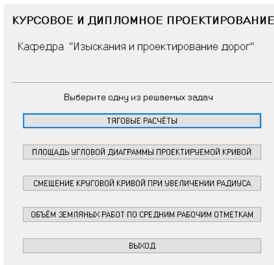
Рис. 1. Программа Railroudcalc
