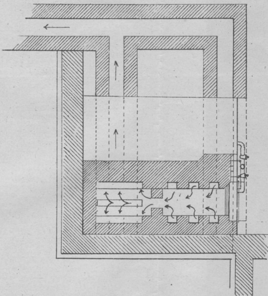
ЧЕРТЕЖ № 2.
