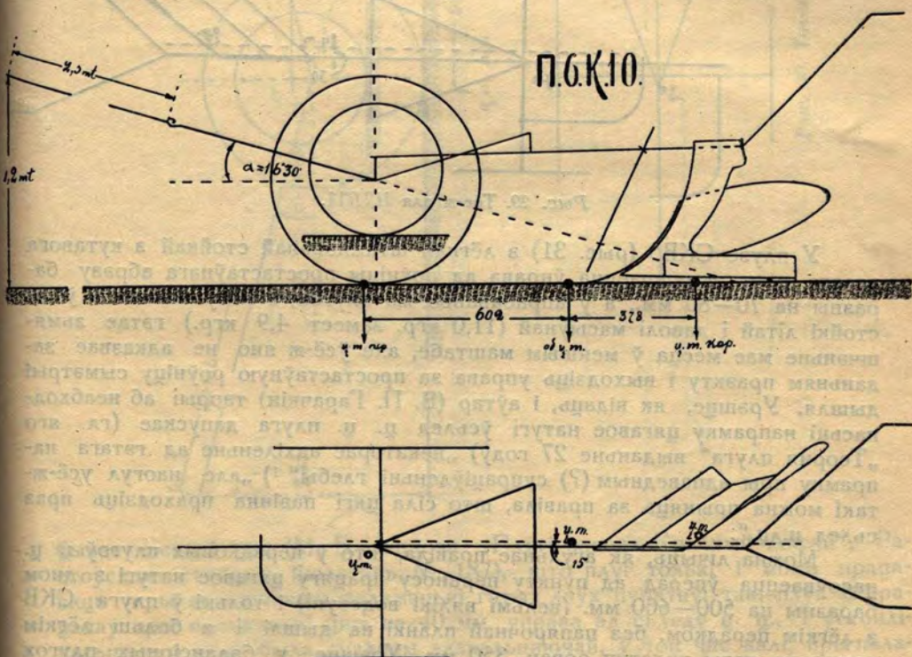
Рыс. 28. Палажэньне праэкцыі ц. ц. ў плуге П6К10.
