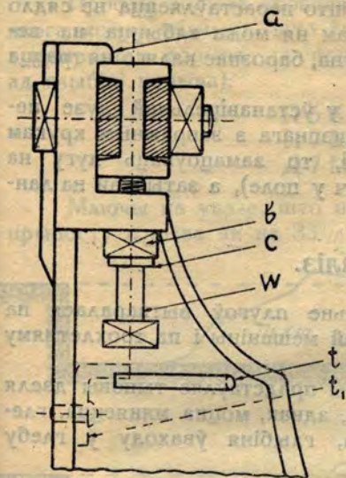
Рис. 32. Упор для нажимнаго шруба і дышла.
