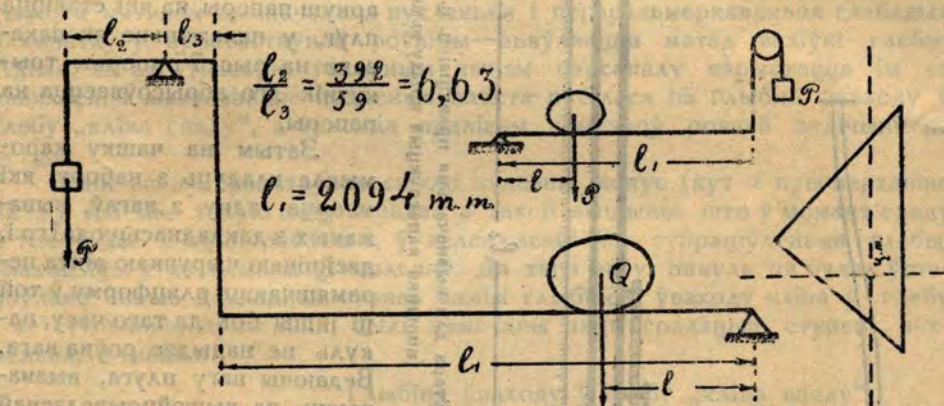
Рис. 6. Схэма вагаў і засечка праэкцыі ц. ц.
