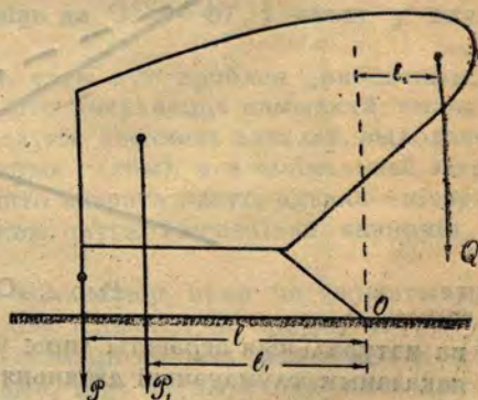
Рыс. 3. Дзеяньне сіл абварочваючых плуг
