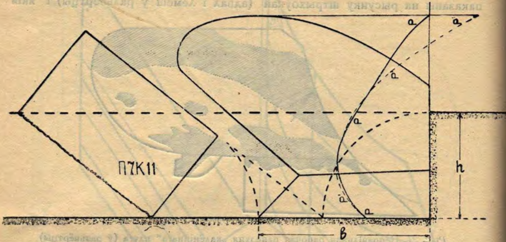
Рис. 26. Тое-ж для плуга П7К11.
