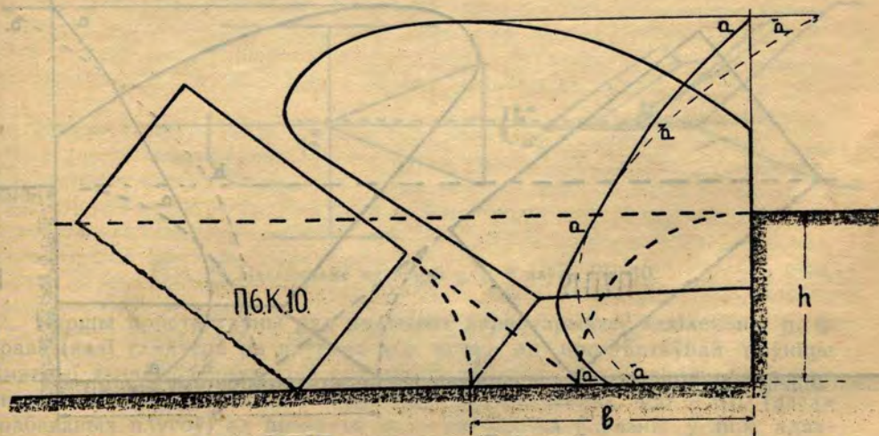
Рис. 25. Палажэньне адваленых пластоў для плуга П6К10.
