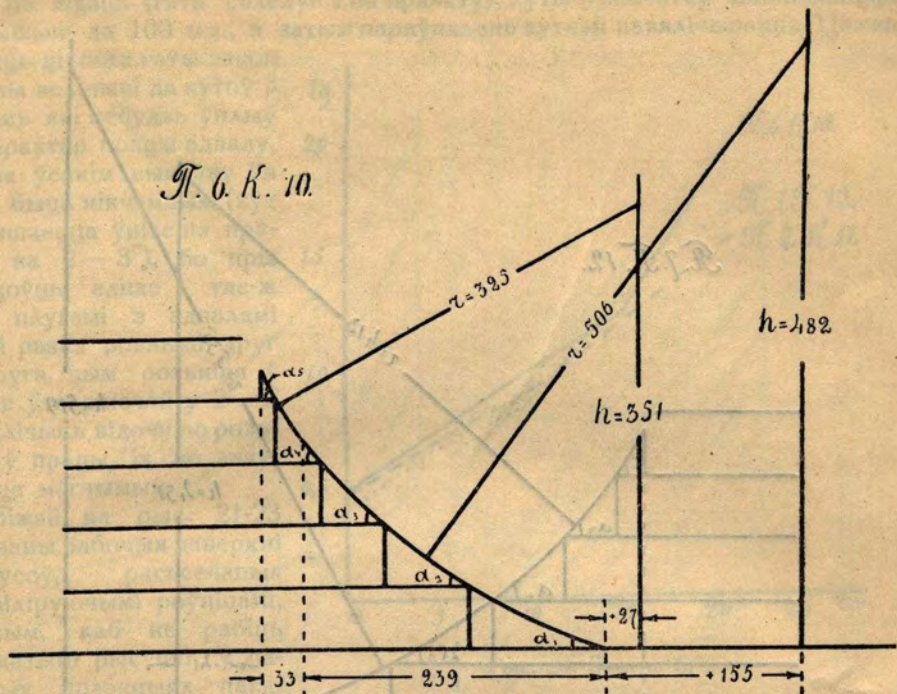
{[Рис. 17. Накіроуваючая корпусу плуга П6К10, яка ляжыць у роўніцы палявой дошкі.
