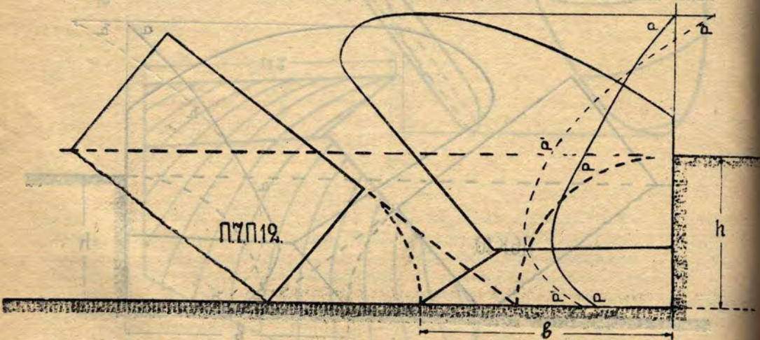
Рис. 27. Тое-ж для плуга П7П12.
