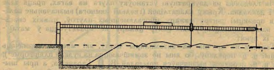
Рис. 8. Профілямер для глебы.
