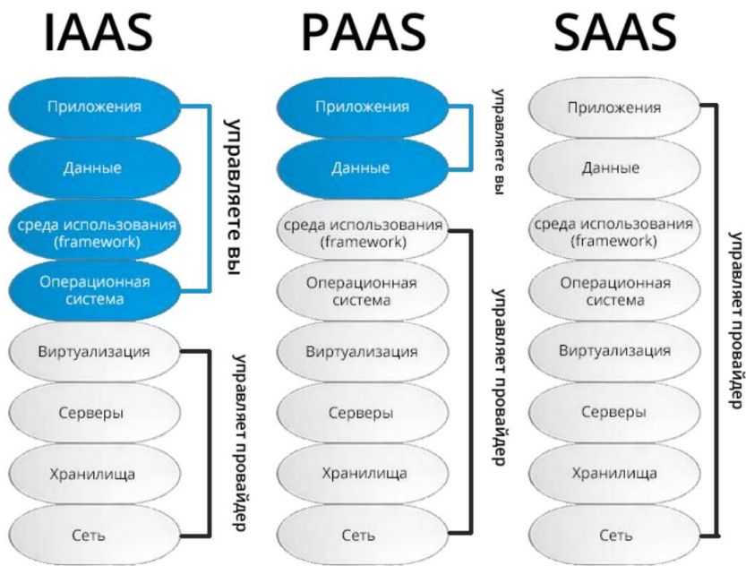
Рис. 1. Составные элементы модели обслуживания облачных сервисов
