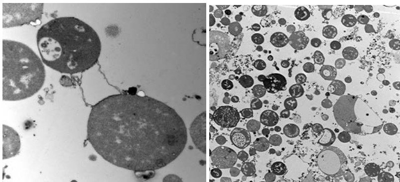
Рис. 5.3. L-формы бактерий
