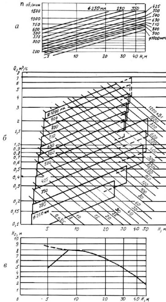
Рис. 1: а – график связи числа оборотов гидротурбины с напором; б – подбор диаметра рабочего колеса гидротурбины; в – определение высоты отсасывания радиально-осевой гидротурбины
