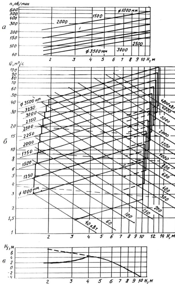
Рис. 1: а – график связи числа оборотов гидротурбины с напором; б – подбор диаметра рабочего колеса гидротурбины; в – график определения высоты отсасывания горизонтальной прямоточной гидротурбины
