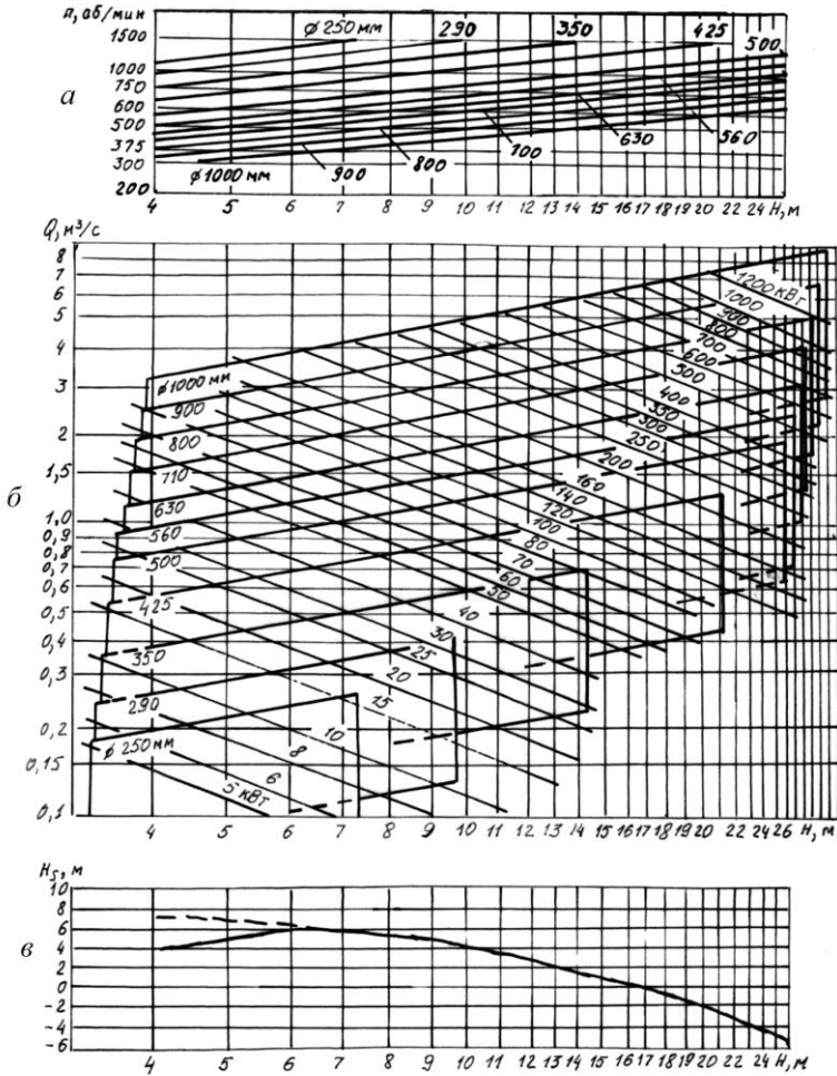
Рис. 1: а – график связи числа оборотов гидротурбины с напором; б – подбор диаметра рабочего колеса гидротурбины; в – определение высоты отсасывания поворотно-лопастной гидротурбины
