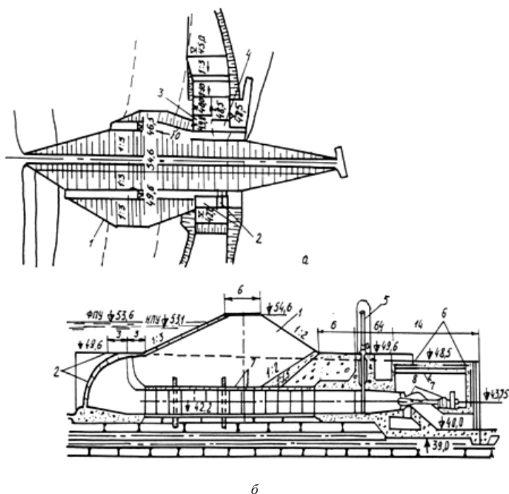
Рис. 9.3. Компоновка основных сооружений плотинной малой ГЭС:
