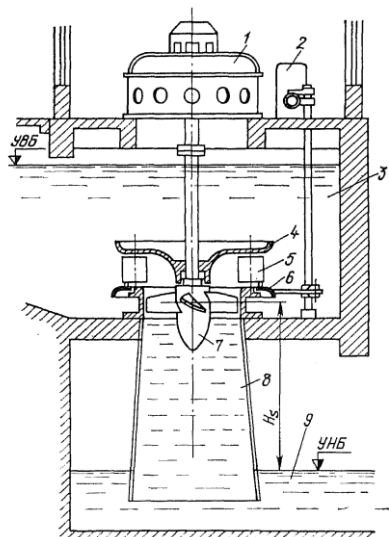
Рис. 8.4. Схема установки с пропеллерной турбиной в открытой турбинной камере:
