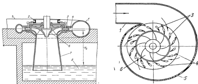
Рис. 8.3. Схема установки с радиально-осевой турбиной: 1 – трубопровод; 2 – поворотное кольцо привода лопаток направляющего аппарата; 3 – лопатки направляющего аппарата; 4 – статорные колонны; 5 – спиральная турбинная камера; 6 – рабочее колесо турбины; 7 – отсасывающая труба; 8 – отводящий канал
