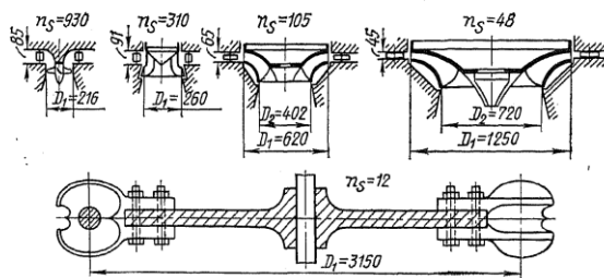
Рис. 8.1. Основные размеры рабочих колес гидротурбин разной быстроходности при N = 1 кВт и H = 1 м (размеры даны в см)
