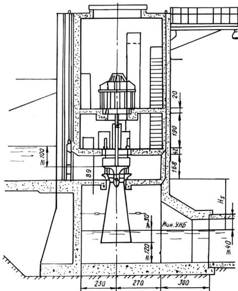
Рис. 7.4. Компонировка здания малой ГЭС с вертикальной осевой гидротурбиной с забором воды непосредственно в турбинную камеру
