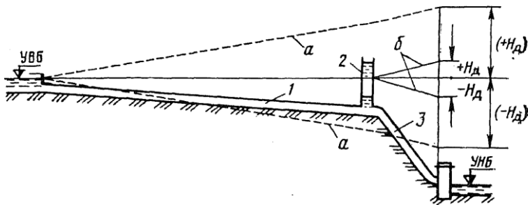
a – при отсутствии уравнительного резервуара; б – при его наличии; 1 – деривационный трубопровод; 2 – уравнительный резервуар; 3 – турбинный трубопровод
