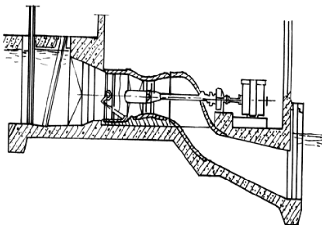
Рис. 7.1. Гидроагрегат с прямоточной горизонтальной гидротурбиной с вынесенным генератором и S-образной отсасывающей трубой
