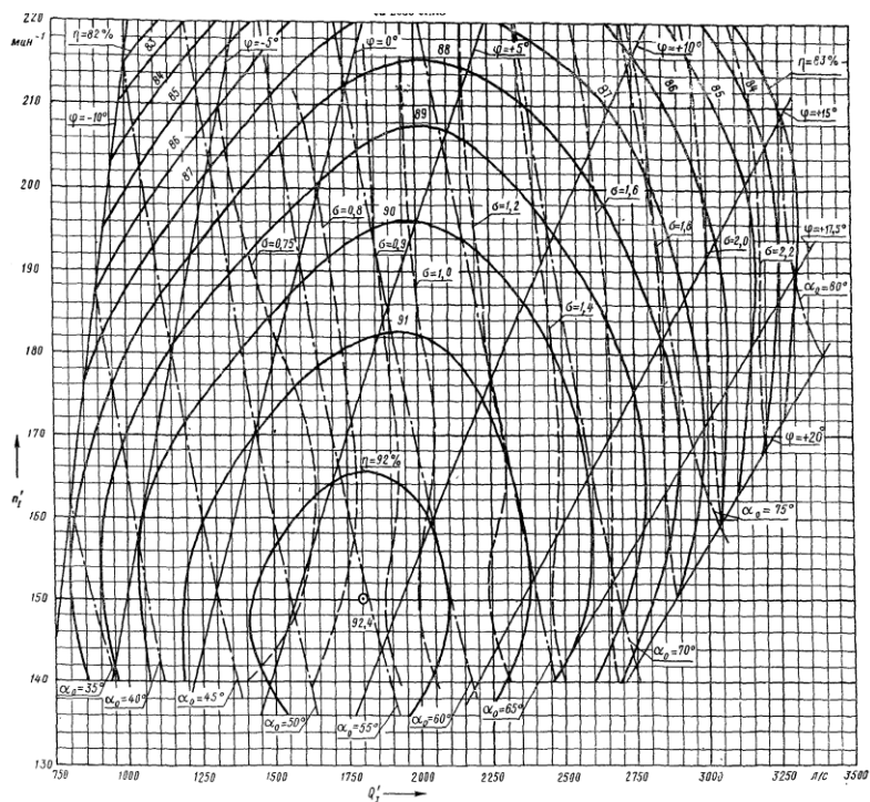
Рис. 8.6. Универсальная энергетическая характеристика гидротурбины типа ПЛ
