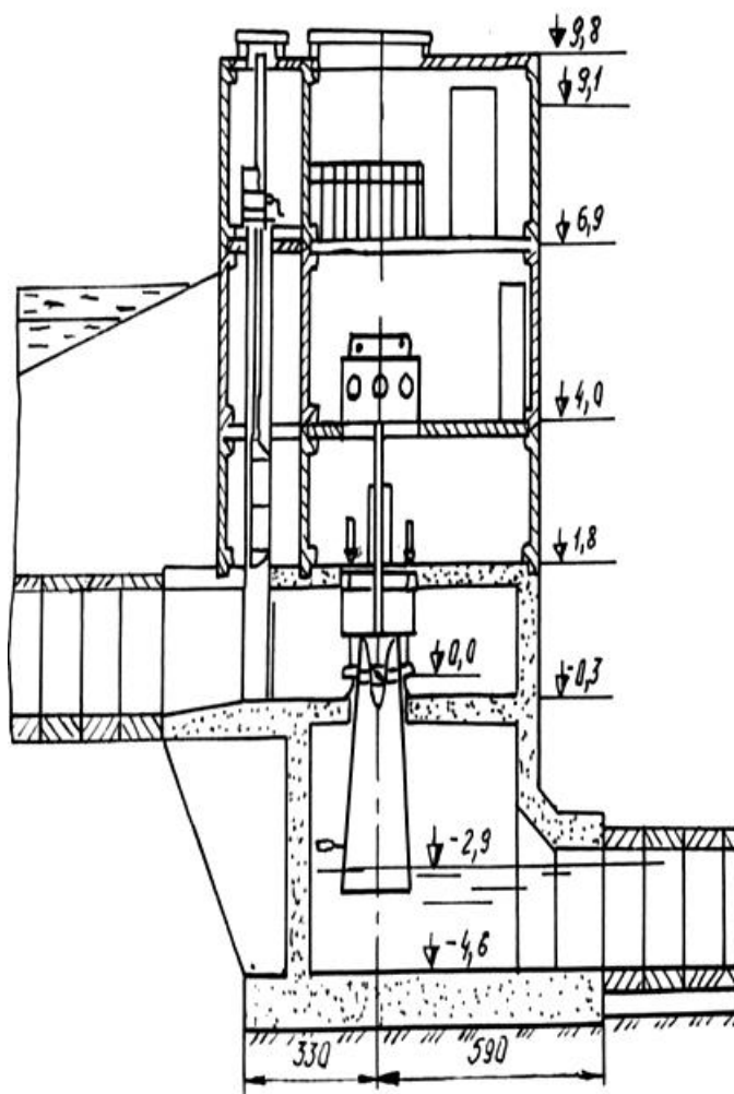
Рис. 9.2. Компонировка зданий малой ГЭС с применением сборного железобетона (вариант конструкции)
