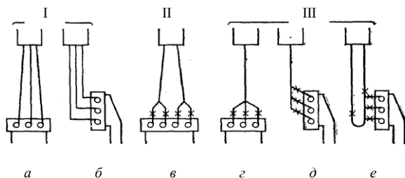
Рис. 9.4. Способы питания турбин при различном подводе трубопроводов к зданию станции: I – раздельное; II – групповое; III – объединенное; а, в, г – фронтальный подвод; б, д, е – продольный подвод
