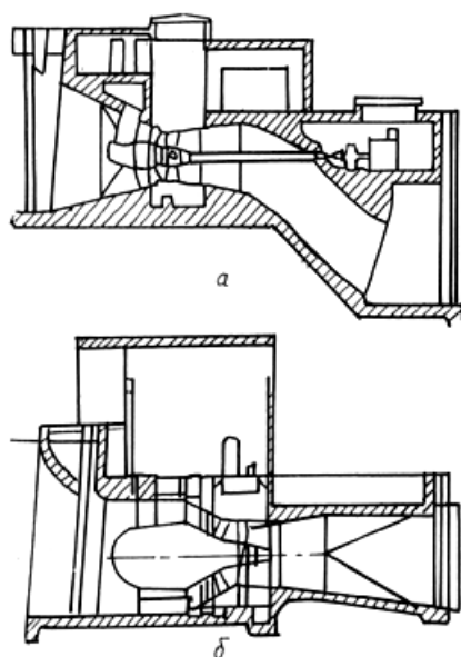
Рис. 7.2. Типовые компоновки агрегатных блоков низконапорных малых ГЭС: a – прямоточный трубный гидроагрегат с вынесенным генератором ( N = 0,5 \dots 10 кВт, H = 4 \dots 25 м); б – капсульный гидроагрегат ( N = 10 \dots 30 кВт, H = 7 \dots 20 м)
