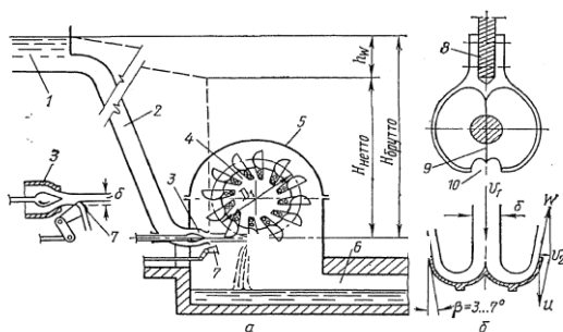
Рис. 8.2. Схема установки с активной (ковшовой) турбиной: а – схема установки; б – схема лопасти (ковша); 1 – напорный бассейн; 2 – турбинный трубопровод; 3 – сопло с регулирующей иглой; 4 – рабочее колесо; 5 – защитный кожух; 6 – отводящий канал; 7 – отклонитель струи; 8 – диск рабочего колеса; 9 – нож ковша; 10 – вырез в ковше для пропуска струи через ковш, находящийся в неблагоприятном положении к струе
