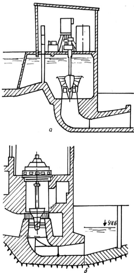
Рис. 7.3. Типовые компоновки агрегатных блоков низконапорных малых ГЭС: а – вертикальная с открытой турбинной камерой ( N = 0,5 \dots 5,0 тыс. кВт, H = 4 \dots 10 м); б – вертикальная с бетонной спиральной камерой
