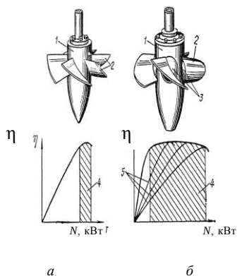
Рис. 8.5. Рабочие колеса и рабочие характеристики пропеллерной (а) и поворотно-лопастной (б) турбин: 1 – втулка рабочего колеса; 2 – лопасти турбины; 3 – поворотная втулка лопастей; 4 – зоны высоких КПД турбины; 5 – характеристики пропеллерных режимов турбины при различных углах установки лопастей
