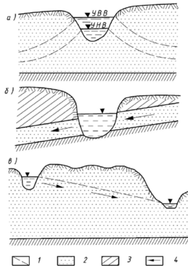
Рис. 1.8. Схема потерь речного стока на питание грунтовых вод: 1 – положение зеркала грунтовых вод; 2 – водоносные слои; 3 – водонепроницаемые или слабопроницаемые пласты; 4 – направление движения подземных вод
