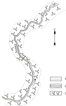
Рис. 2.1. План визуальной съемки в районе намеченного участка гидрологического поста:
