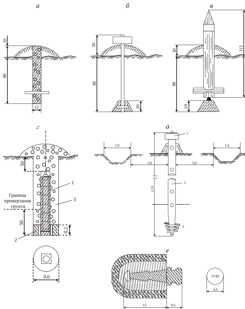
Рис. 2.7. Долговременные знаки закрепления съёмочных сетей и реперы гидрологических постов (размеры даны в см): а – бетонный пилон; б – отрезок железной трубы с бетонным монолитом; в – деревянный столб с крестовиной на бетонном монолите; г – потайной грунтовый репер: 1 – пилон; 2 – якорь-плита; 3 – котлован; д – стандартный грунтовый репер: 1 – головка; 2 – металлическая труба; 3 – винт; е – репер-марка
