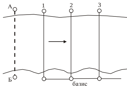
Рис. 2.30. Расположение створов для измерения скорости течения воды поплавками: 1 – верхний створ; 2 – основной створ; 3 – нижний створ; AB – пусковой створ
