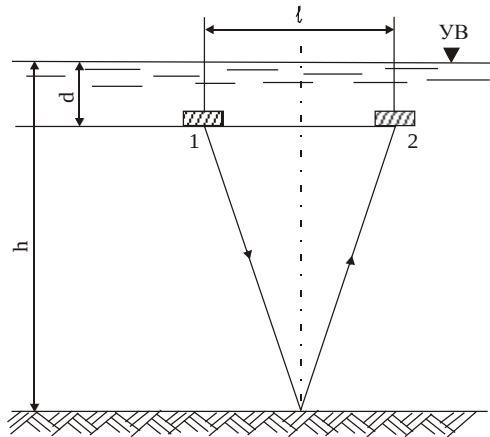
Рис. 2.15. Схема измерения глубины акустическим методом:
