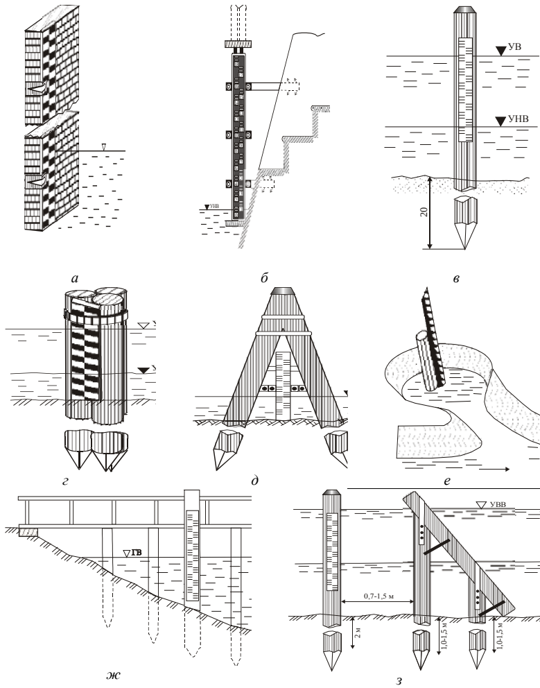
Рис. 2.3. Речной водомерный пост: а – на каменной стенке; б – на мостовом устье; в – на одиночной свае; г, д – на кусте свай; е – на свае в ковше; ж – на свае мостика; з – на одиночной свае с ледорезом
