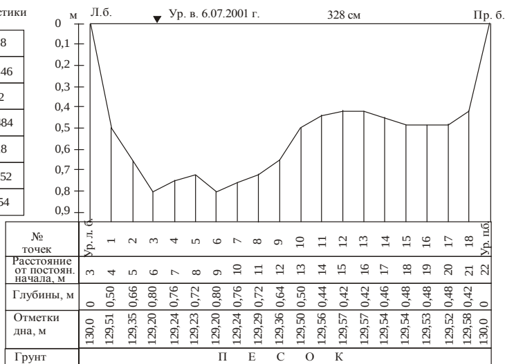
Рис. 2.17. Поперечный профиль реки
