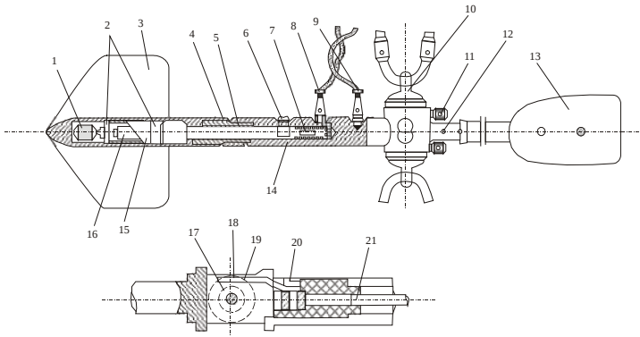
Рис. 2.26. Устройство гидрометрической вертушки ГР-21М:
