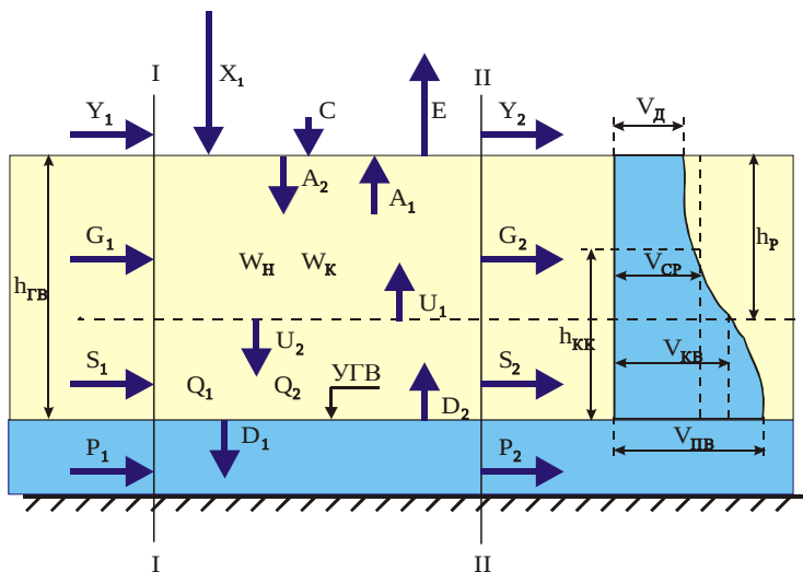
Рис. 1.17. Схема влагообмена: X_1 – сумма атмосферных осадков; C – конденсация водяных паров воздуха, не учитываемая осадкомерами; E – суммарное испарение;
