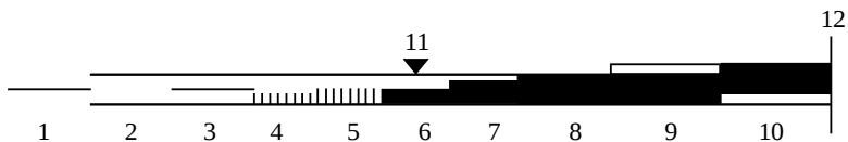
Рис. 2.51. Ледовые явления: 1 – сало; 2 – забереги; 3 – сало при берегах; 4 – редкий шугоход; 5 – шугоход; 6 – редкий ледоход; 7 – ледоход; 8 – неподвижный ледяной покров (ледостав); 9 – вода течет поверх льда; 10 – закраины и лед подняло;
